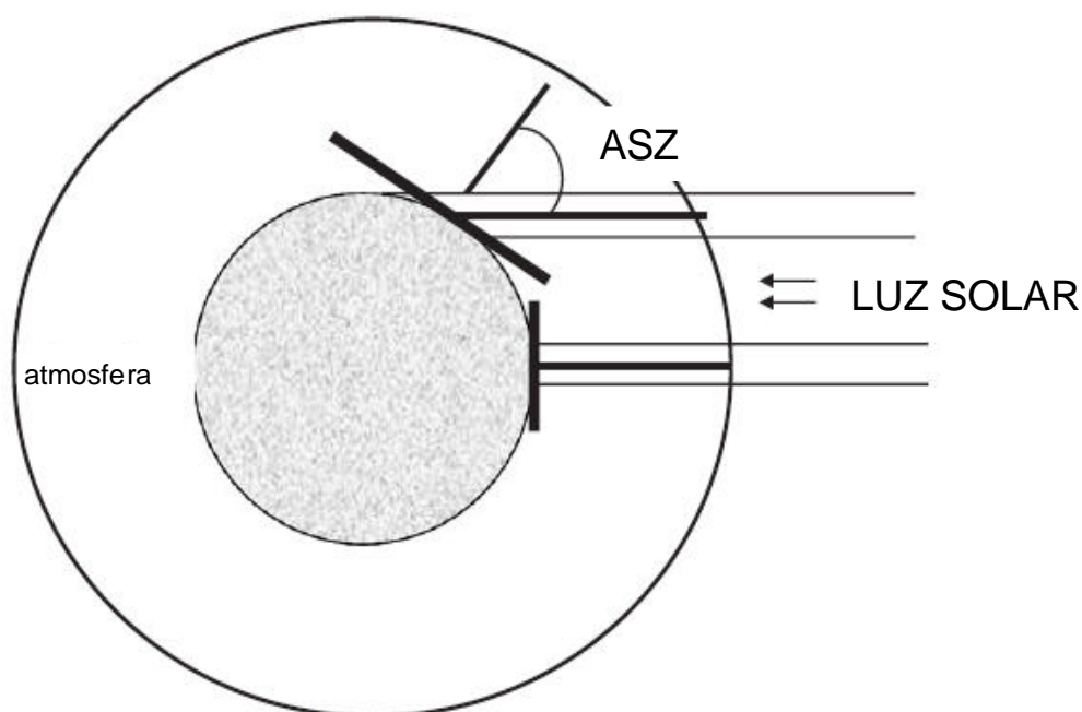
Figura 6: Ângulo Solar Zenith (ASZ) (adaptado de Webb, 2006) (102).
