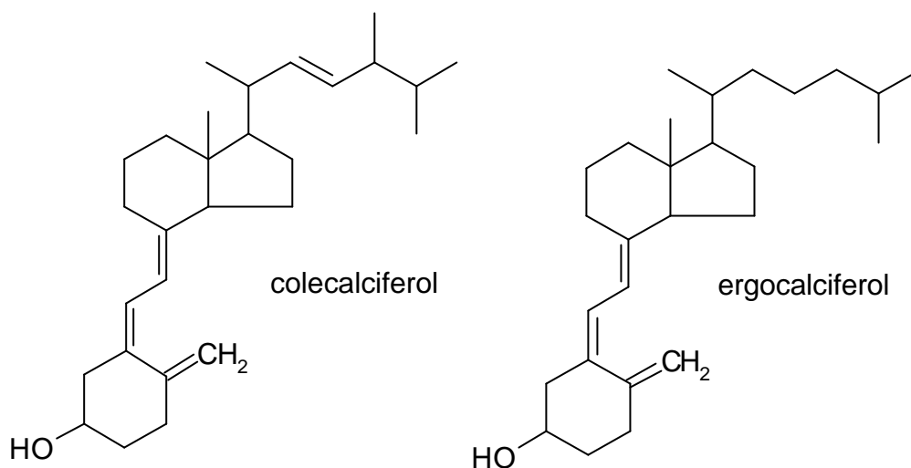
Figura 3: Estruturas químicas do colecalciferol (vitamina D3) e ergocalciferol (vitamina D2).
