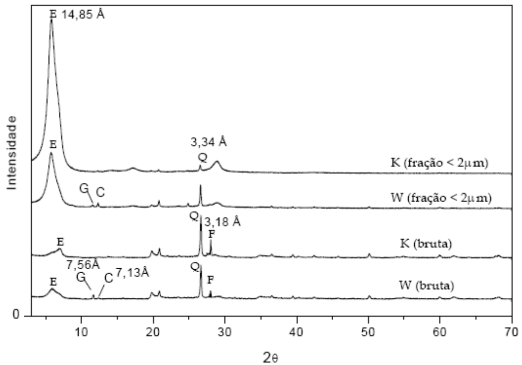
Figura 4. DRX das amostras brutas e das frações < 2 μm. (E = esmectita, C = caulinita, Q = quartzo, F = feldspato, G = gesso) [17].
