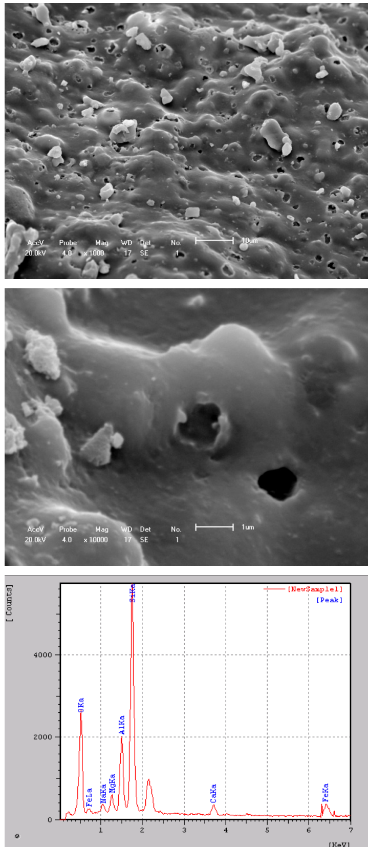
Figura – 30. Micrografias e EDS obtidos por microscopia eletrônica de varredura para a argila Brasgel seca em 150 °C e tratada termicamente em 1000 °C.
