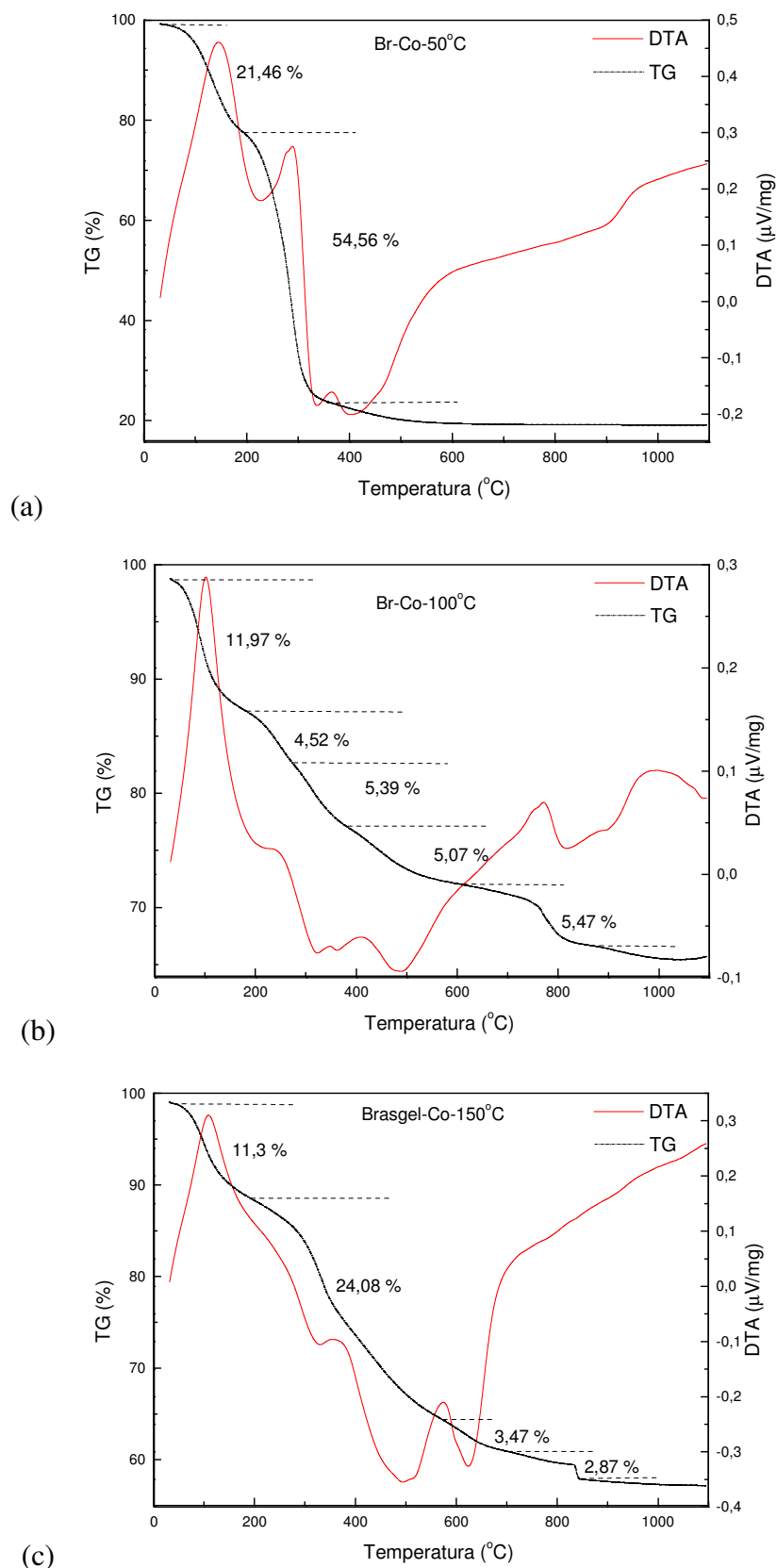
Figura – 21. Curvas TG/ATD da argila Brasgel modificada com cobalto coloidal, seca em (a) 50, (b) 100 e (c) 150 ° C. Pico para cima endotérmico e para baixo exotérmico.
