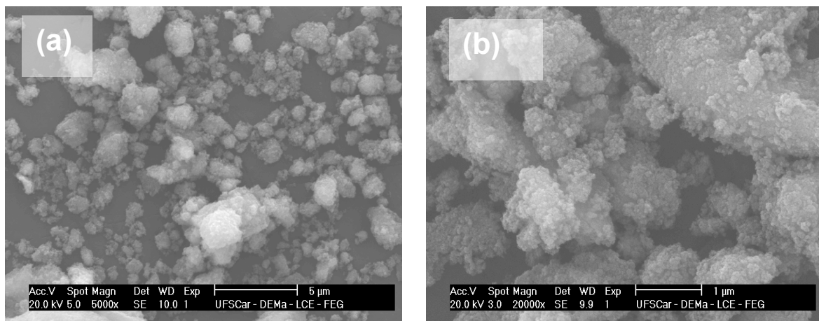
Figura 16 – Microscopia eletrônica de varredura dos pós obtidos com uréia nas condições P = 70\% (630 W) e t = 10 min. (NU4), com aumentos de (a) 5K e (b) 20K.
