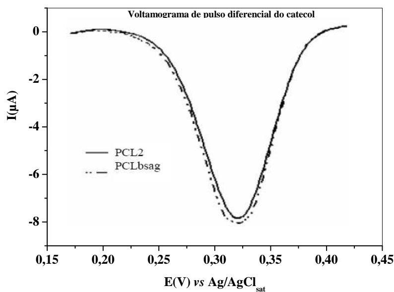
Figura 4.14. Voltamogramas de Pulso Diferencial do catecol. Tampão fosfato 0,1 \text{molL}^{-1} pH 7,0; Faixa de varredura: 0,4 a 0,0V; Velocidade de varredura: 30 \text{mVs}^{-1} ; Potencial de pulso: 50 mV.
