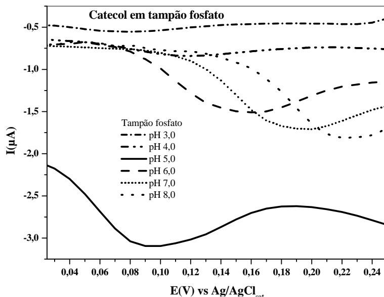
Figura 4.13. DPV do catecol [ 5,0 \times 10^{-5} \text{molL}^{-1} ] em diferentes pHs do eletrólito fosfato ( 0,1 \text{molL}^{-1} ). Eletrodo de trabalho: PCL2. Faixa de varredura: 0,4 a 0,0V. Potencial de pulso: 50mV. Velocidade de varredura: 30 \text{mVs}^{-1} .
