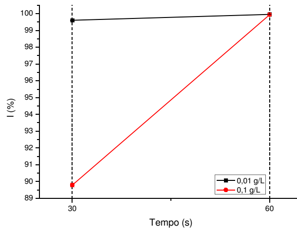
Figura 4.10 - Médias previstas para a inativação (I %) de Escherichia coli em resposta a interação dos fatores tempo de exposição à UV, 30 e 60s e concentração celular, 0,01 e 0,1g/L.
