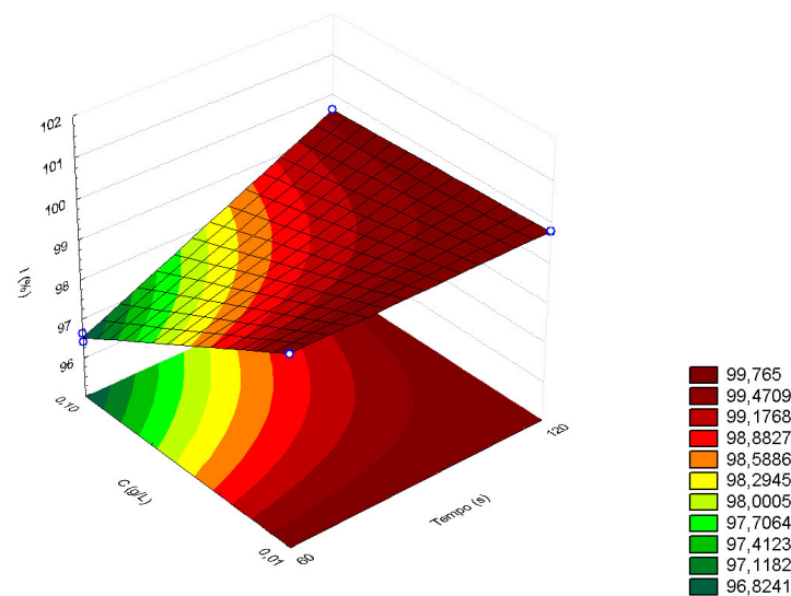
Figura 4.14 - Efeito do tempo de exposição à radiação UV, 60 e 120s e da concentração celular, 0,01 e 0,1g/L sobre a inativação (I %) de Saccharomyces cerevisiae .
