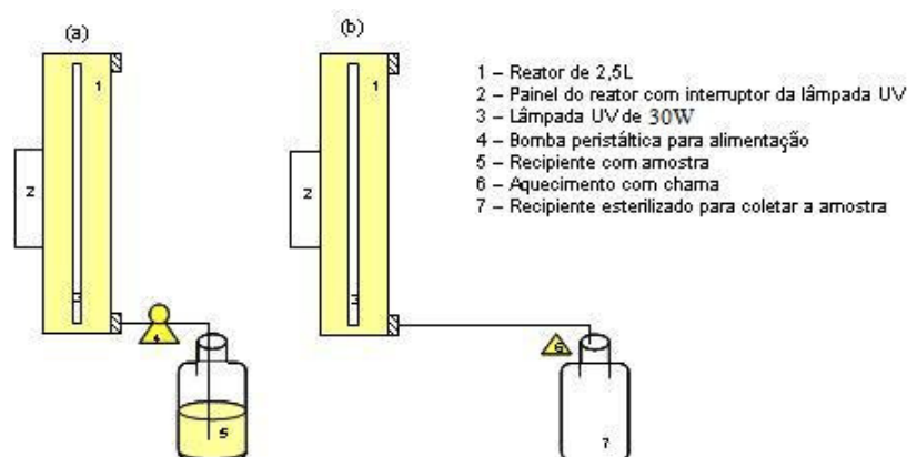
Figura 3.7 - Esquema da alimentação da amostra no reator (a) e da descarga do reator (b).
