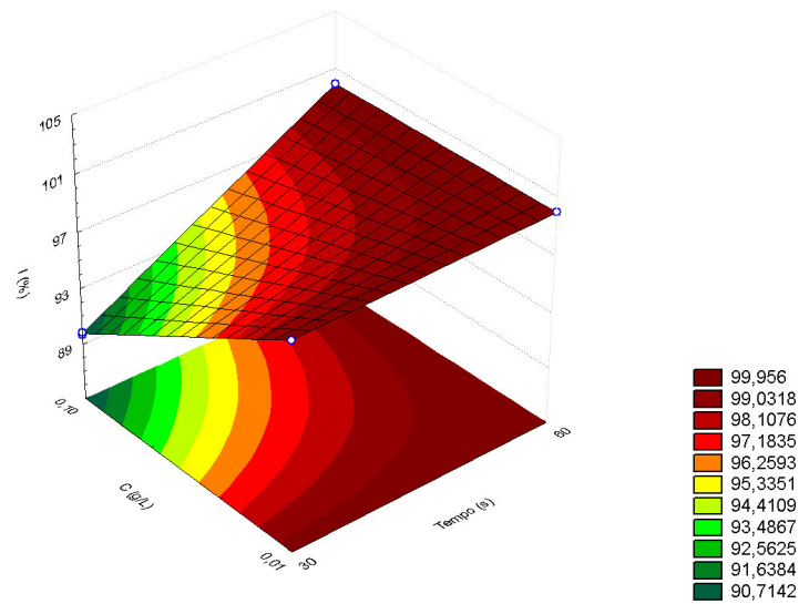
Figura 4.9 - Efeito do tempo de exposição à radiação UV, 30 e 60s e da concentração celular 0,01 e 0,1g/L sobre a inativação (I %) de Escherichia coli .
