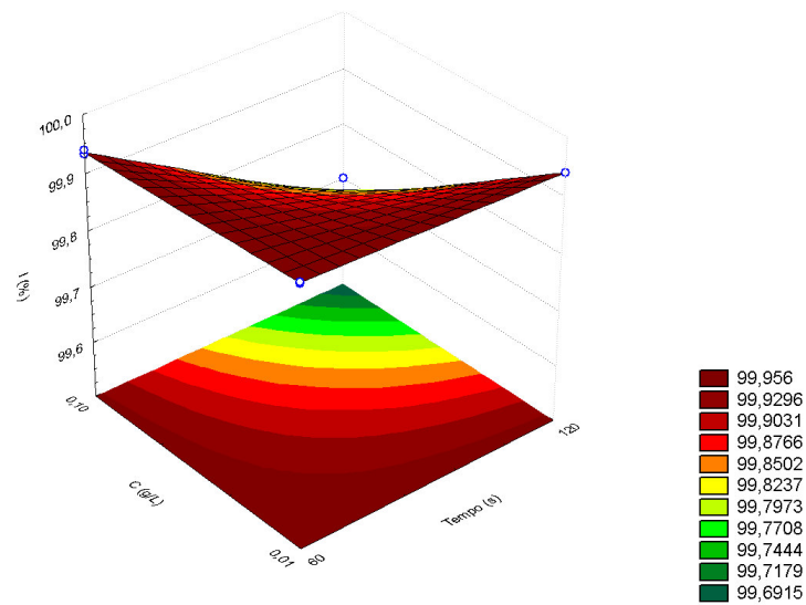
Figura 4.12 - Efeito do tempo de exposição à radiação UV, 60 e 120s e da concentração celular, 0,01 e 0,1g/L sobre a inativação (I %) de Escherichia coli .
