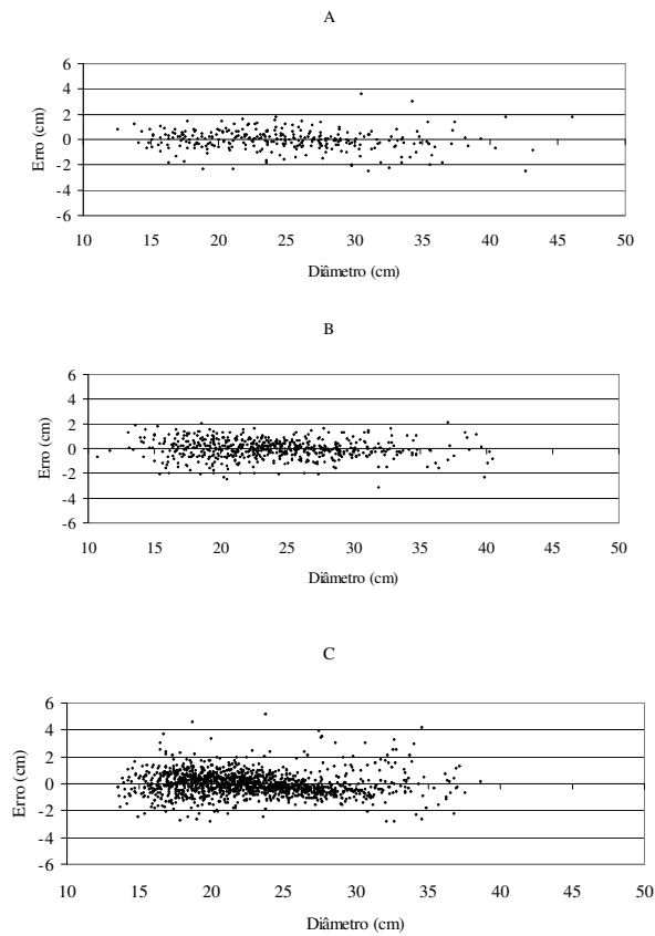
FIGURA 8 Gráficos de resíduos encontrados para as três funções de afilamento.
