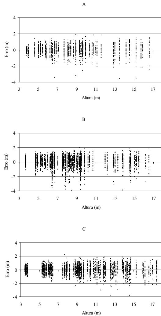
FIGURA 9 Gráficos de resíduos encontrados para as três equações de altura total.
