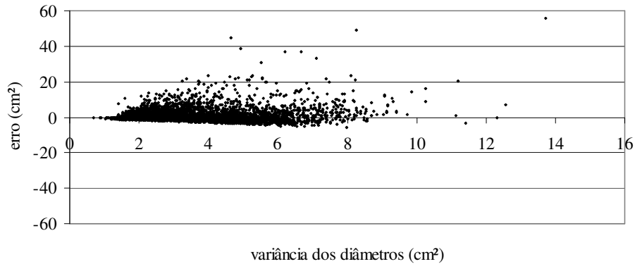
FIGURA 10 Gráfico de resíduos de variância dos diâmetros para o modelo 1.
