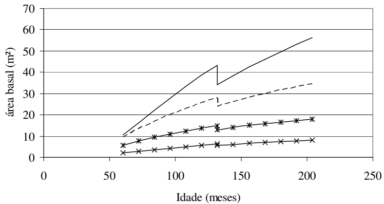
FIGURA 16 Projeção de volume e área basal com desbaste, para os quatro índices de sítio estudados.
