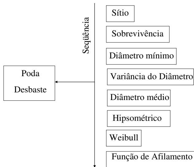
FIGURA 1 Seqüência das equações no sistema de prognose.
