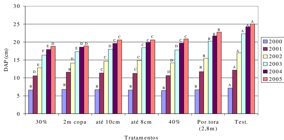
FIGURA 5 Teste de medias Scott-Knott para DAP, realizada a cada ano de medição, no experimento Tuna*.
