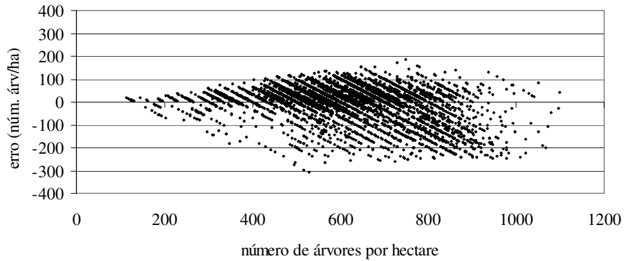
FIGURA 8 Gráficos de resíduos para os modelos de Clutter modificado selecionado para estimar a sobrevivência.
