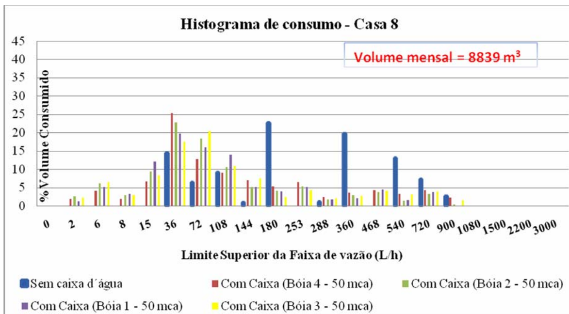
Figura 5.12 (b) – Perfis de consumo registrados, com abastecimento direto e com a simulação do uso de caixa-d'água controlada pelas bóias – Casa 8
