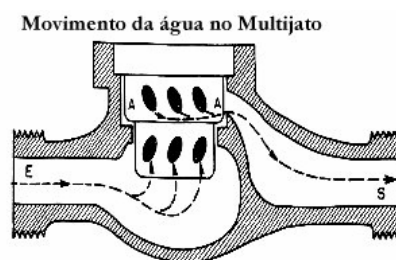
Figura 3.7– Movimento da água no medidor velocimétrico multijato (DMAE)
