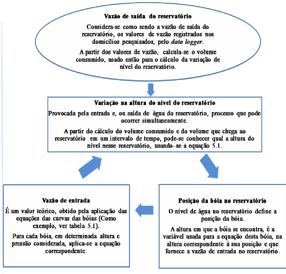
Figura 4.13 – Fluxograma da simulação do nível em um reservatório doméstico
