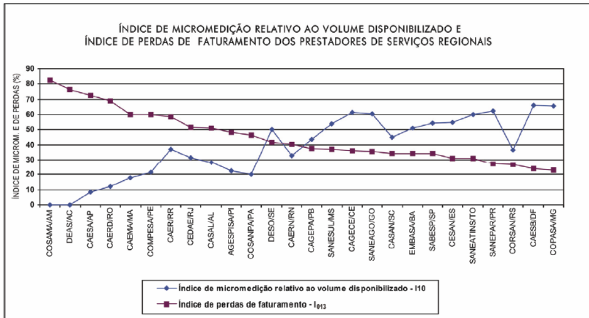
Figura 1.4 - Relação entre índice de perdas em relação ao índice de micromedição nas diversas companhias de saneamento (SNIS, 2005)
