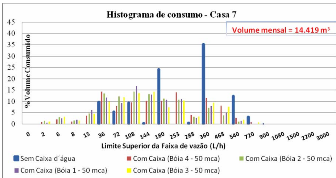
Figura 5.12 (a) – Perfis de consumo registrados, com abastecimento direto e com a simulação do uso de caixa-d'água controlada pelas bóias – Casa 7
