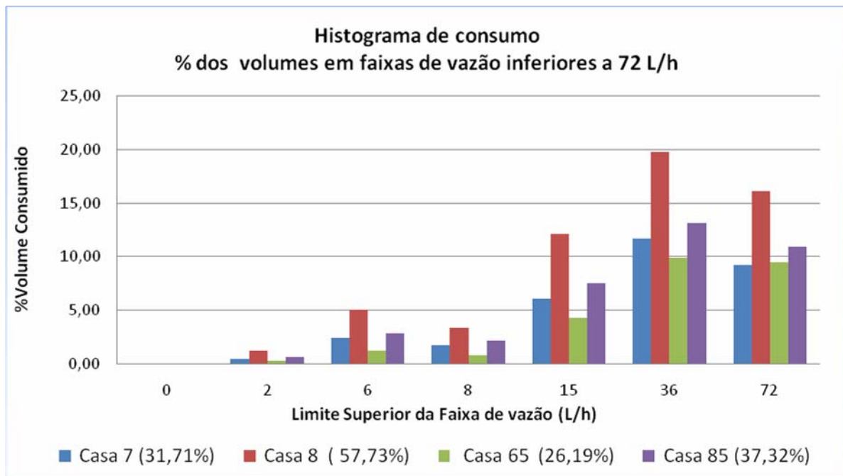
Figura 5.15 – Histograma de consumo com os percentuais de consumo nas vazões até 72 L/h, considerando-se o uso de caixa-d'água
