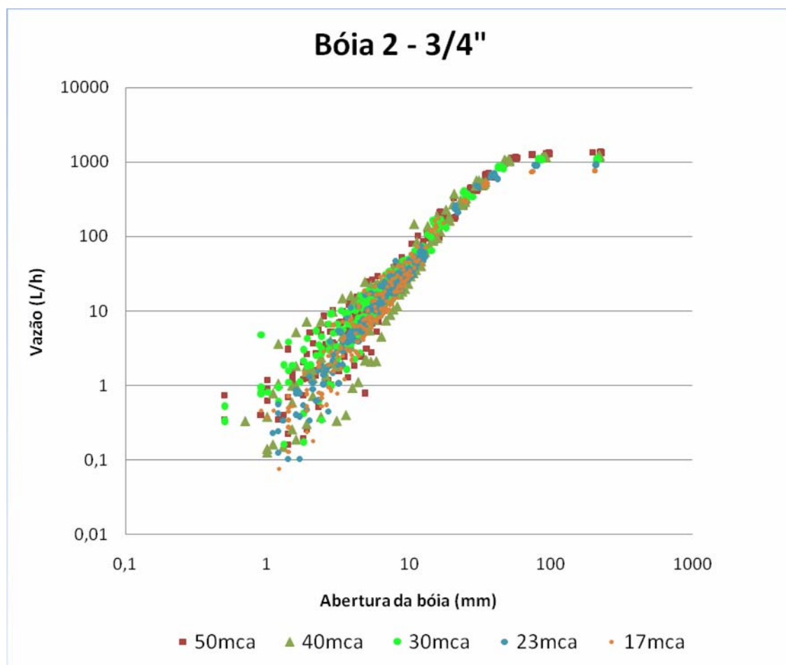
Figura 5.1 – Comportamento das vazões nas bóias da marca A para cada valor de pressão
