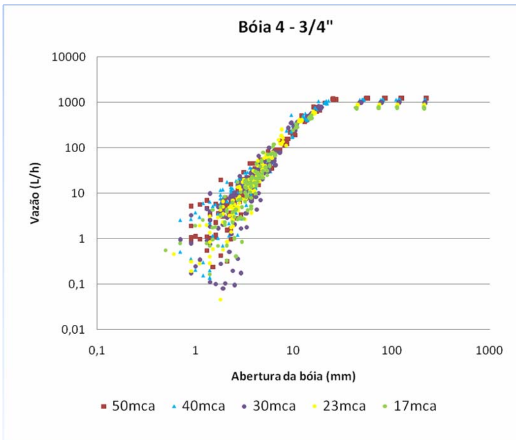
Figura 5.2 – Comportamento das vazões nas bóias da marca B para cada valor de pressão
