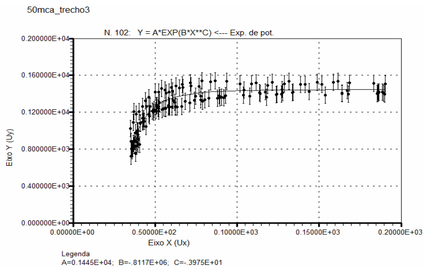
Figura 5.6 – Curvas ajustadas para a bóia 1 na pressão de 50 mca
