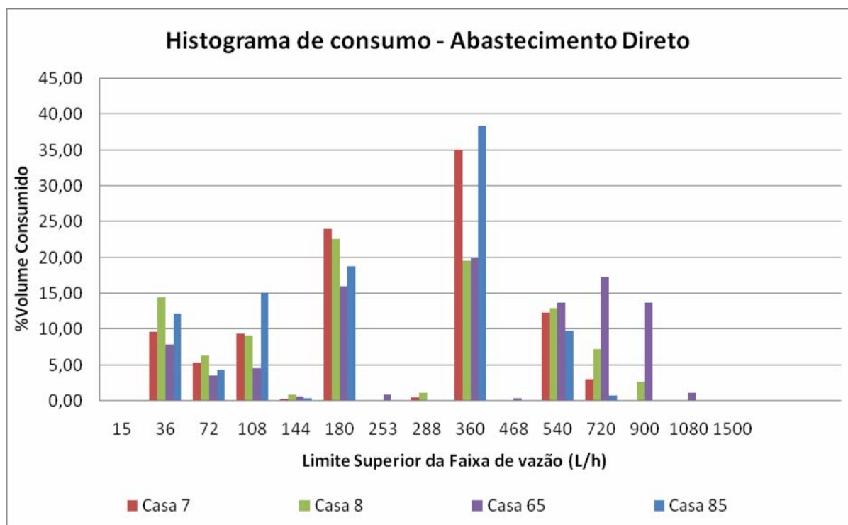
Figura 5.11 – Perfis de consumo registrados nas residências estudadas, com abastecimento direto
