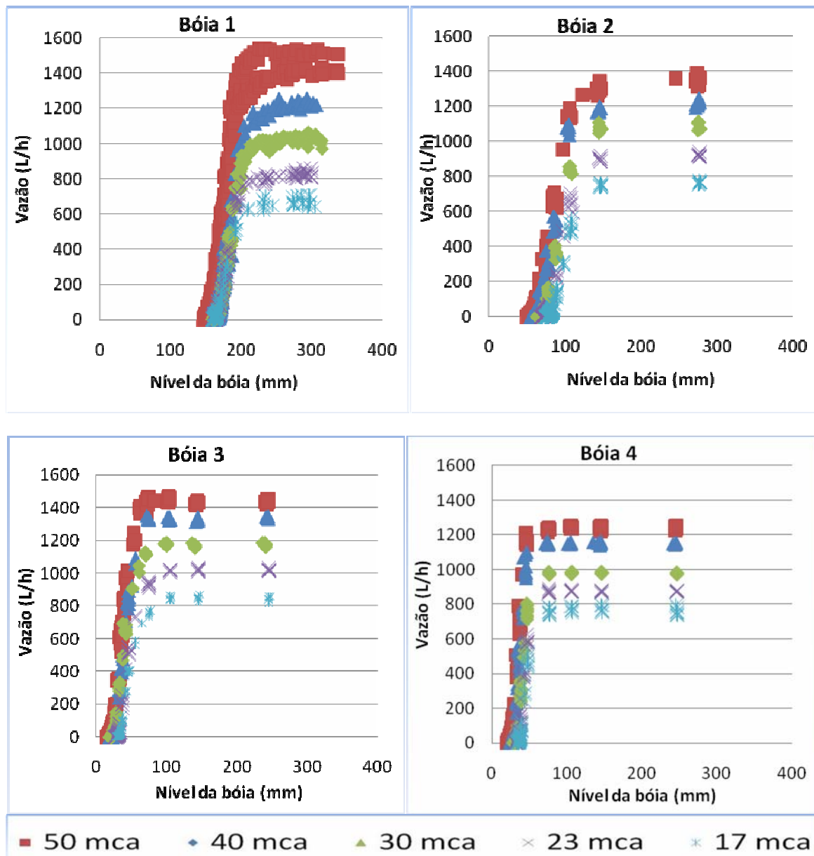
Figura 5.4– Curvas de vazões obtidas em cada uma das bóias e representação da distância de deslocamento da haste até o ponto de início de funcionamento da bóia
