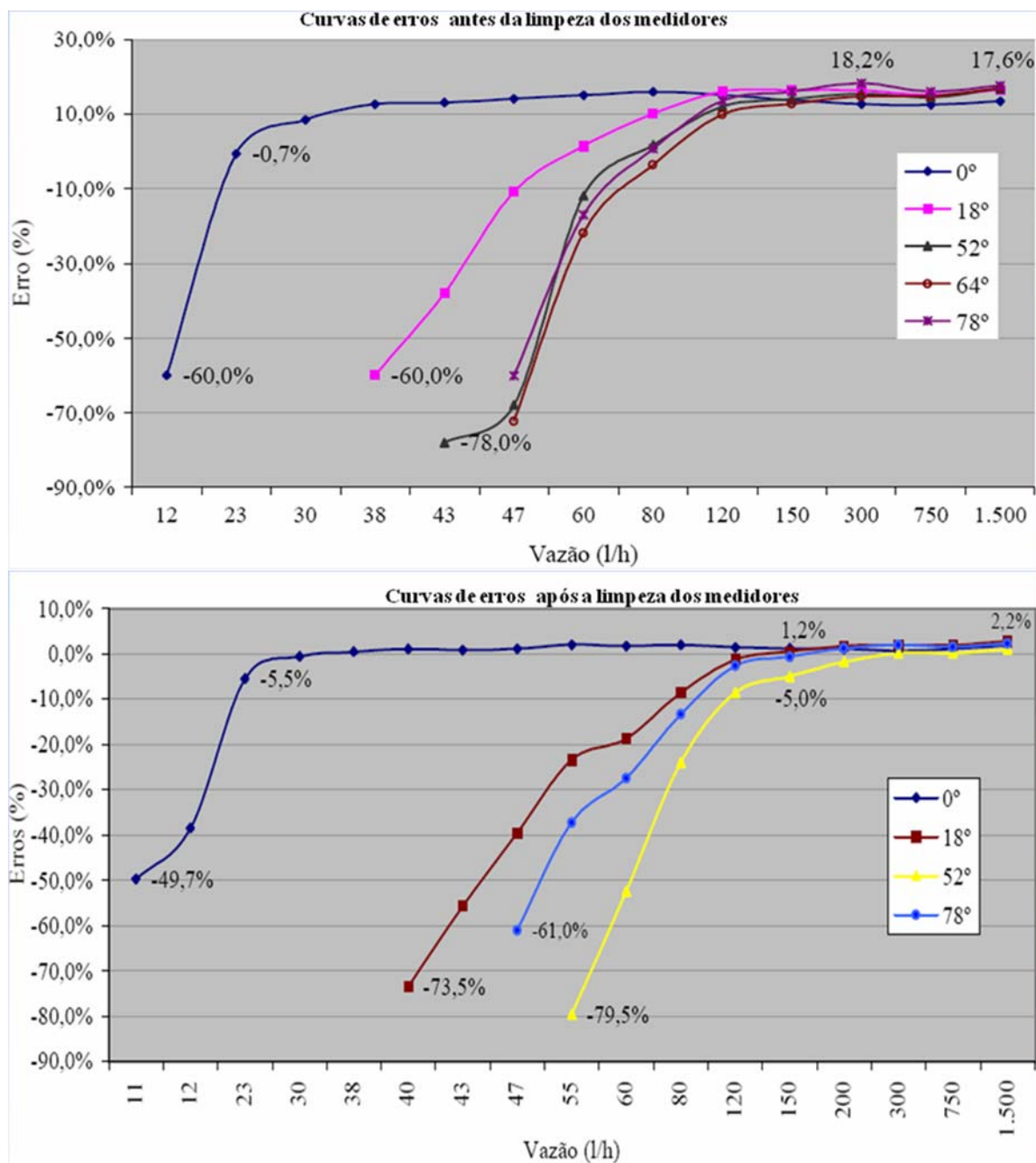
Figura 3.24 – Curvas de erros dos medidores nas posições de operação (Mello, 2000)
