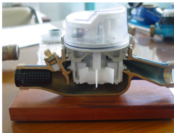
Figura 3.6 – Hidrômetro velocimétrico do tipo multijato
