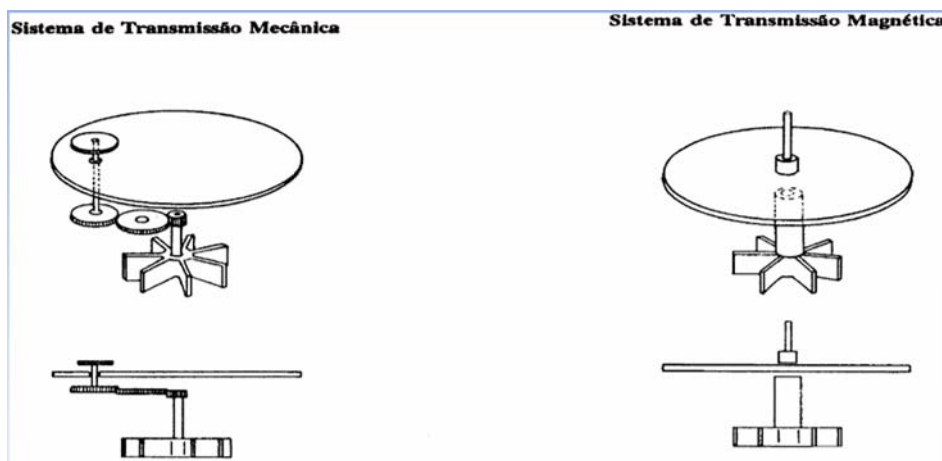
Figura 3.11 – Tipos de transmissão para medidores velocimétricos (Alves et al., 2004)
