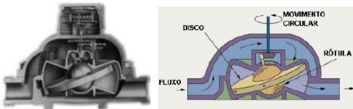
Figura 3.9 – (a) Hidrômetro volumétrico de disco nutante (Alves et al, 2004); (b) Características do hidrômetro volumétrico de disco nutante (Frangipani, 2005)
