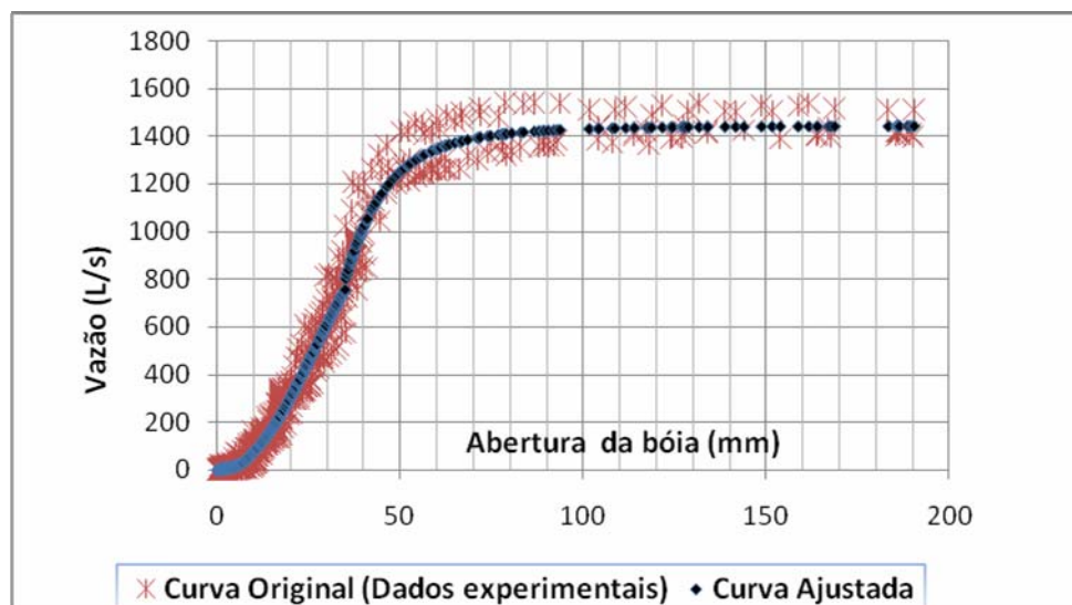
Figura 5.5 – Curva original obtida no experimento para a bóia 1 na pressão de 50 mca
