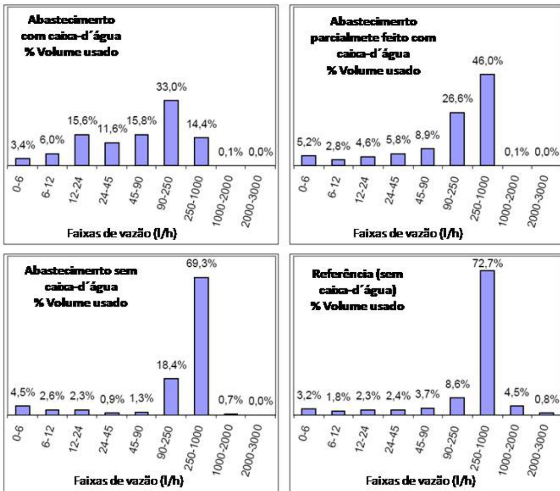
Figura 3.14 – Perfis de consumo para diferentes tipos de abastecimento (Cobacho et al., 2007, modificado)
