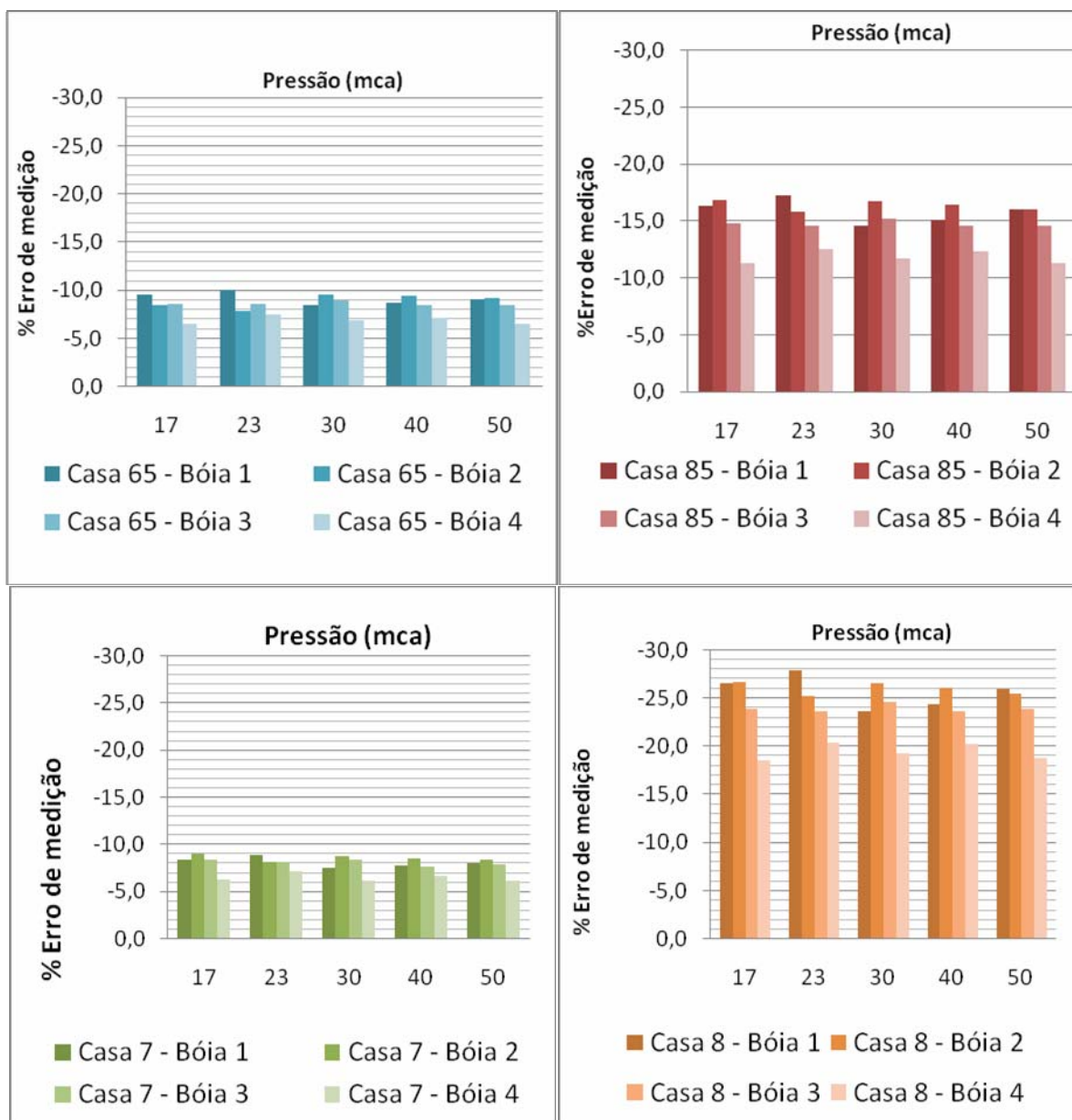
Figura 5.14 – Submedição simulada para as casas 7, 8, 65 e 85, considerando-se todas as 4 bóias utilizadas e as cinco pressões de ensaio, com a curva de erro dos hidrômetros
