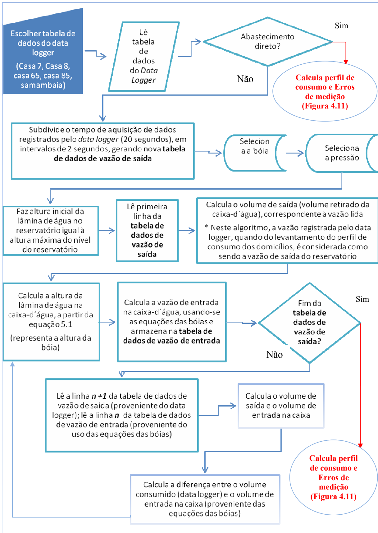
Figura 4.14 – Fluxograma para cálculo do perfil de consumo e dos erros de medição
