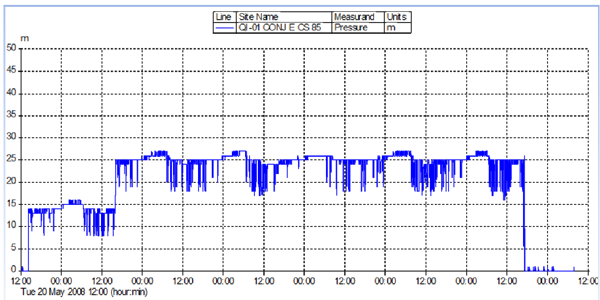
Figura 5.8 – Variação de pressão ao longo do tempo em uma das residências em estudo
