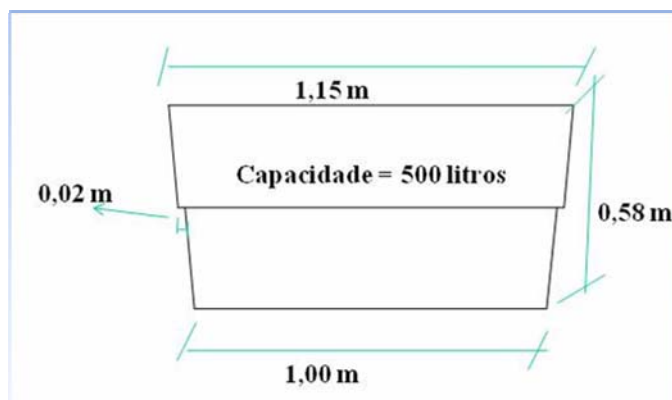
Figura 4.10 – Características do reservatório doméstico adotado como modelo
