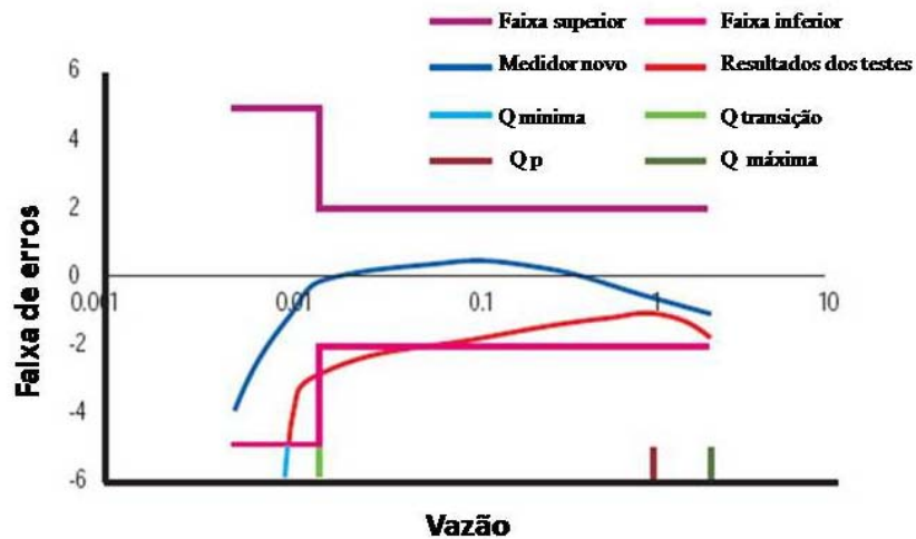
Figura 3.13 – Curva típica de exatidão de medidores de água (Rizzo, 2004)
