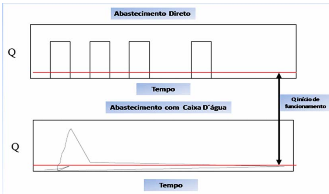
Figura 3.16 – Comportamento das vazões em abastecimento direto e com caixa-d'água (Thornton e Rizzo, 2002)
