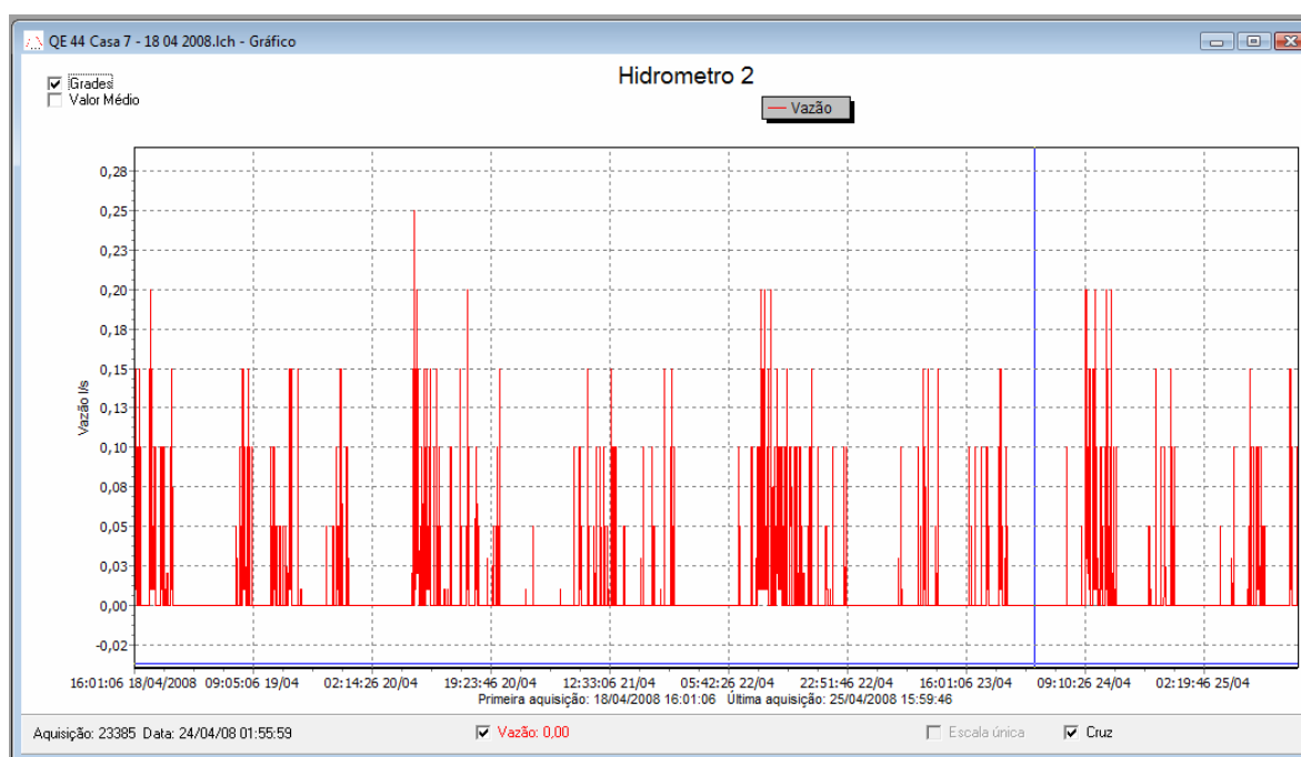
Figura 5.10 – Vazões registradas na casa 7 da QE 44
