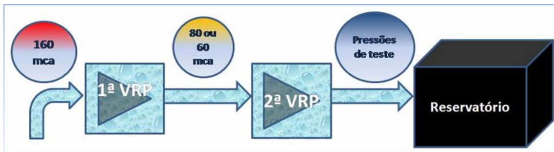
Figura 4.3– Configuração das VRP utilizadas
