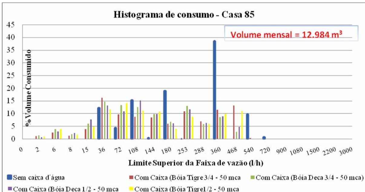
Figura 5.12 (d) – Perfis de consumo registrados, com abastecimento direto e com a simulação do uso de caixa-d'água controlada pelas bóias – Casa 85
