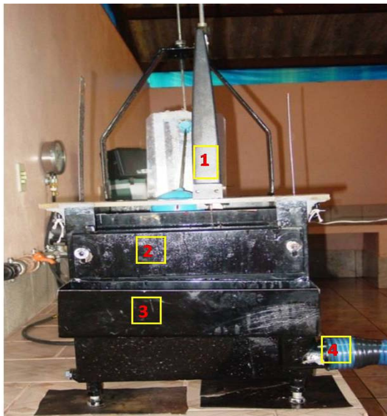
Figura 4.8 – Vista frontal da caixa (1 = linígrafo; 2 = vertedor retangular; 3 = caixa coletora da água extravasada; 4 = tubo na saída da caixa coletora para medição da vazão)
