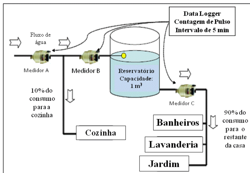
Figura 3.18 – Esquema de instalação dos equipamentos usados para determinar submedição (Rizzo, 2005, modificado)
