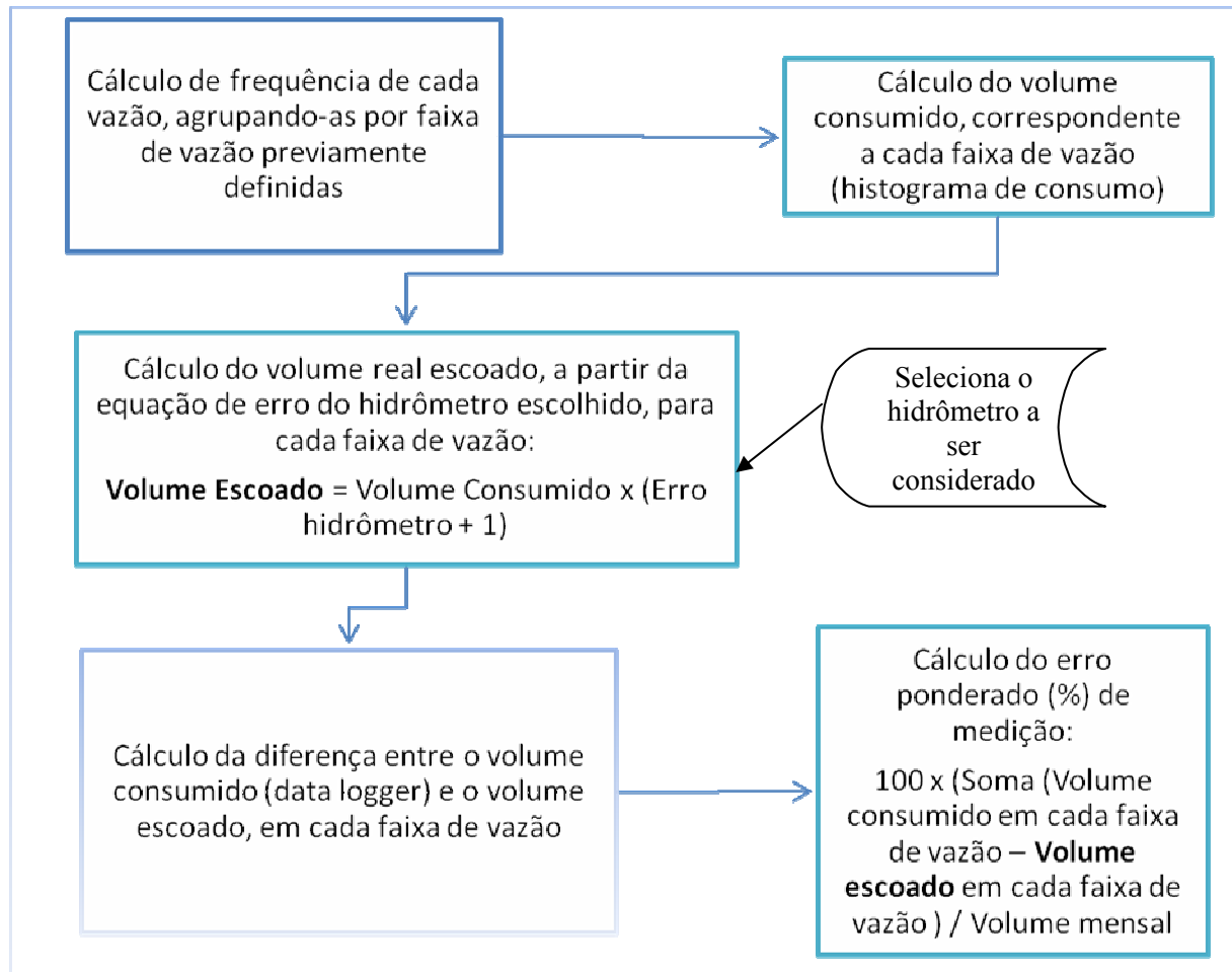
Figura 4.12 – Fluxograma para cálculo do perfil de consumo e dos erros de medição
