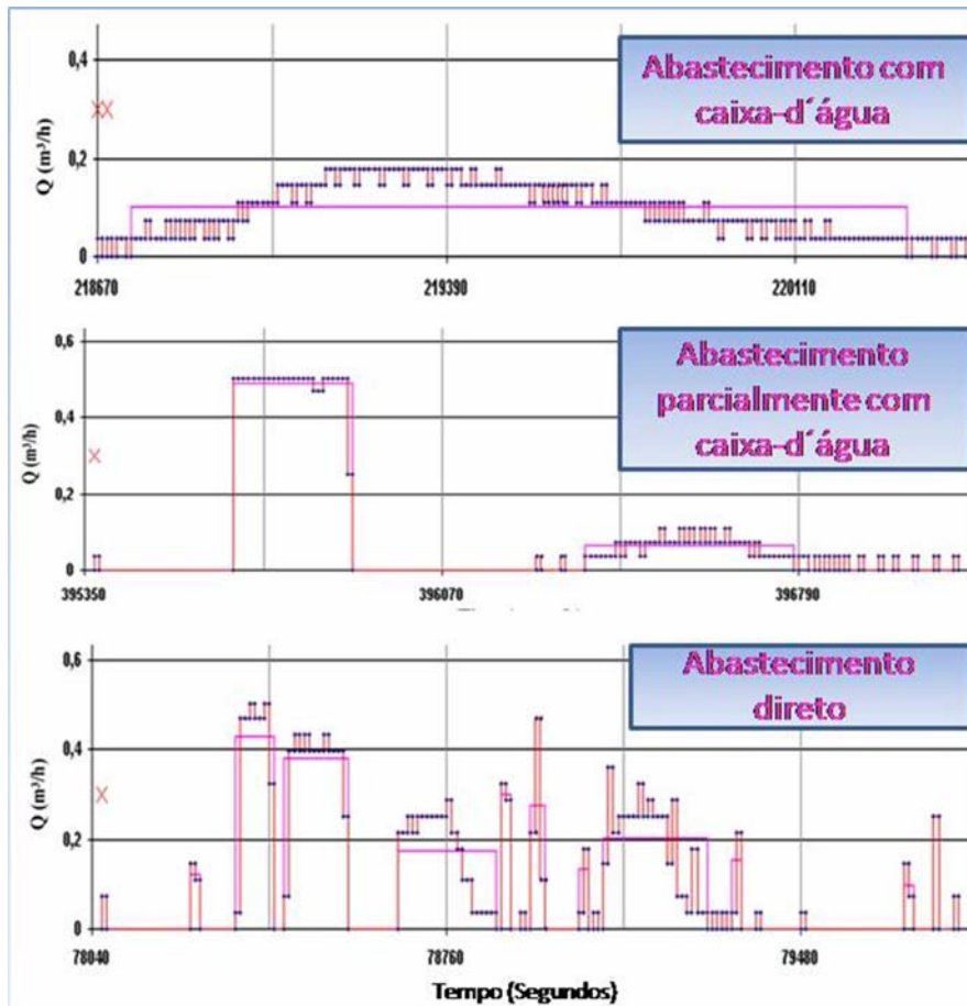
Figura 3.17 - Comportamento das vazões em abastecimento com caixa-d'água, abastecimento misto e sem caixa-d'água (Cobacho et al., 2007)
