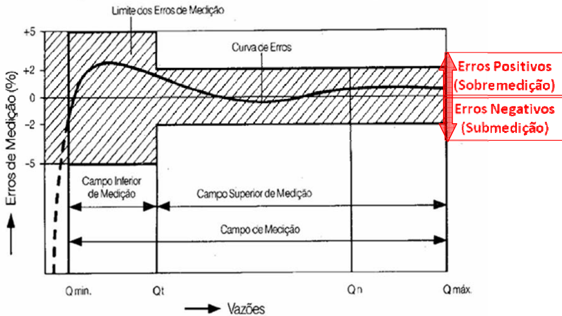
Figura 3.12 – Curva de erros (Alves et al., 2004, modificado)
