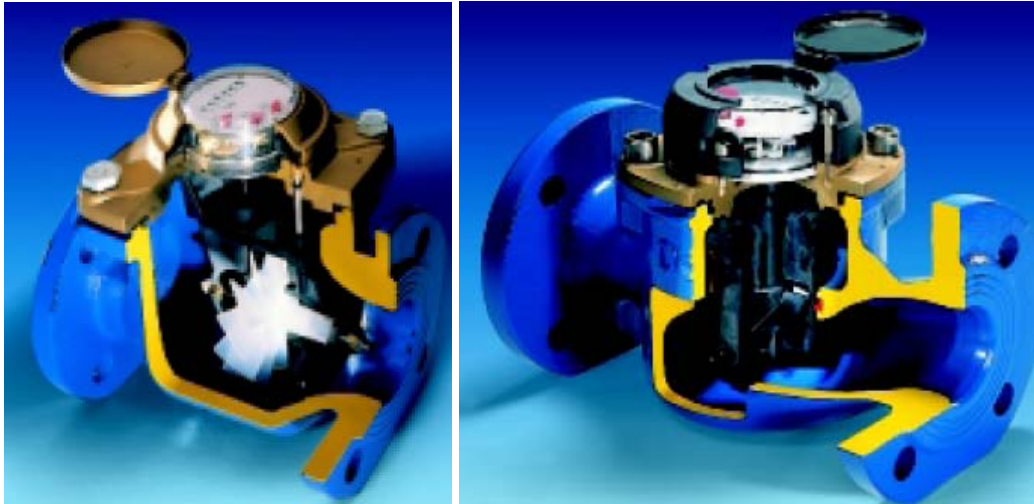
Figura 3.8 – (a) Hidrômetro Woltmann horizontal; (b) Hidrômetro Woltmann vertical
