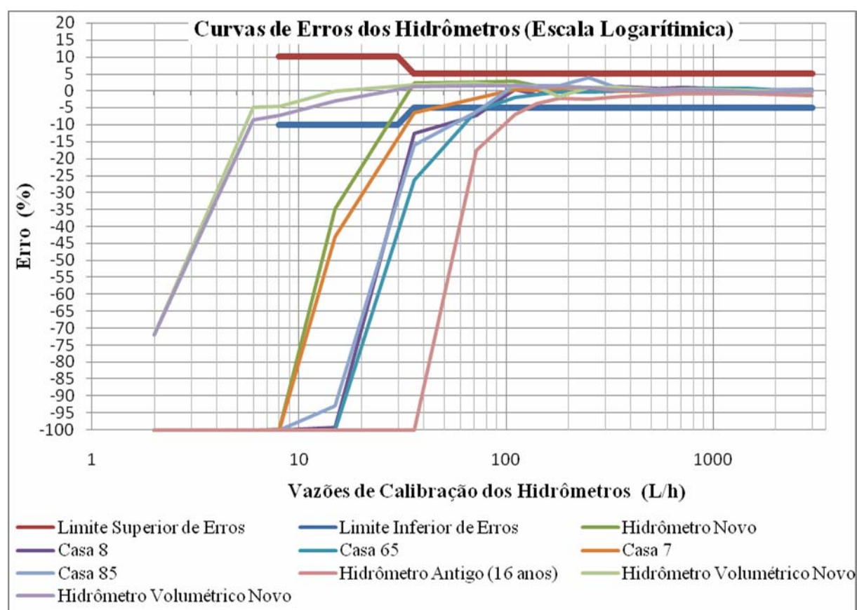
Figura 5.13 – Curvas obtidas com a calibração em bancada dos hidrômetros usados no experimento
