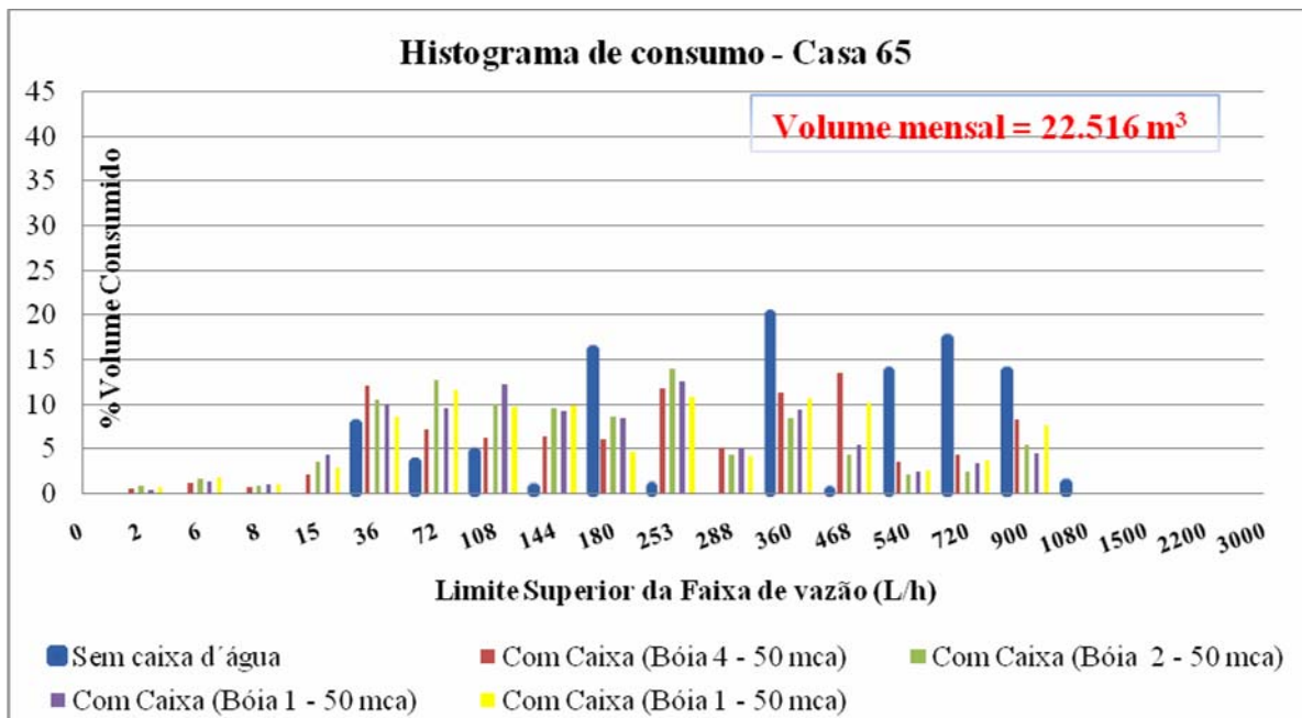
Figura 5.12 (c) – Perfis de consumo registrados, com abastecimento direto e com a simulação do uso de caixa-d'água controlada pelas bóias – Casa 65
