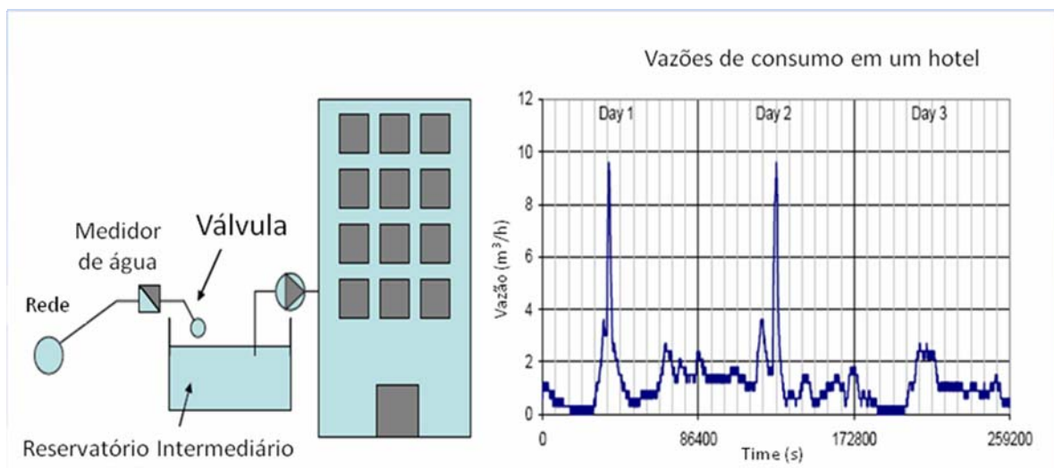
Figura 3.25 - Vazão amortecida pelo reservatório intermediário (Arregui, 2005)
