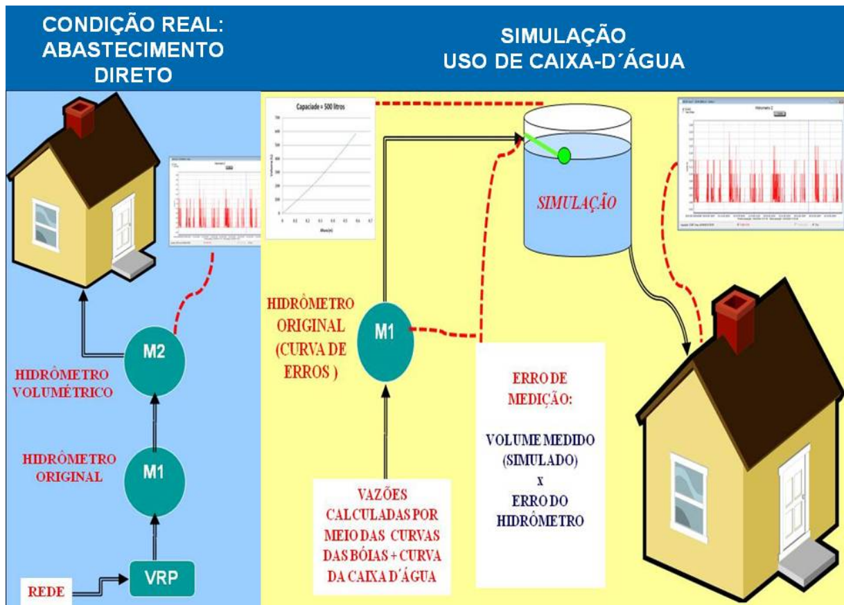
Figura 4.11 – Esquema da condição real e simulação do uso de caixa-d'água
