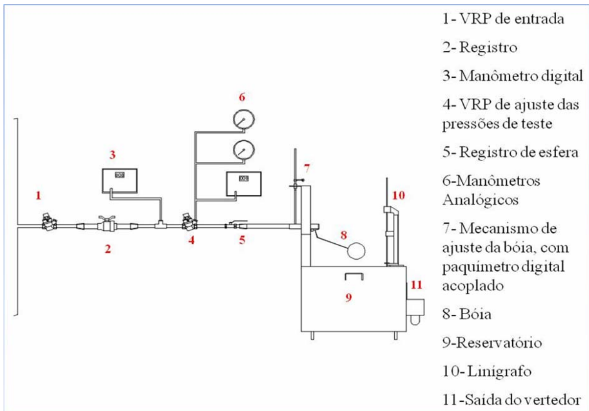
Figura 4.4 – Esquema da montagem do aparato experimental
