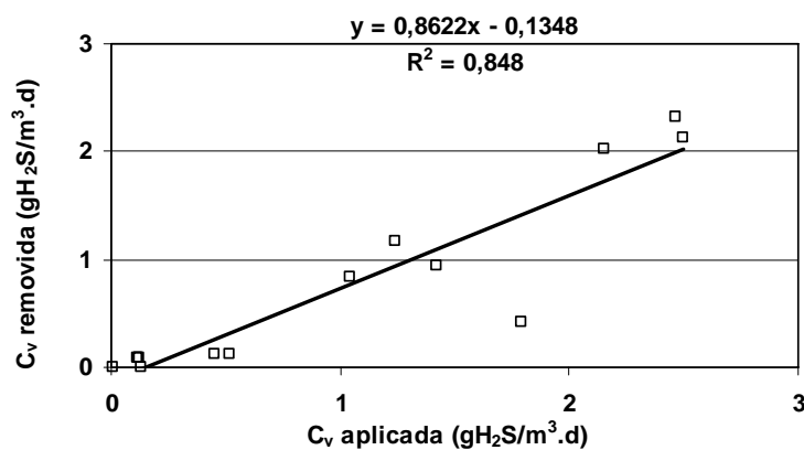
Figura 5.11: Eficiência de remoção no biofiltro de cana - etapa I.
