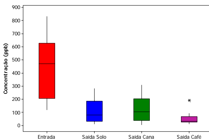
Figura 5.37: Dispersão dos dados de concentração do H 2 S na entrada e saídas - etapa IV.
