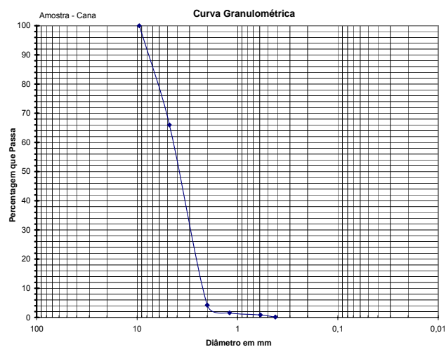
Curva granulométrica da cana picada.
