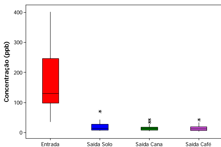
Figura 5.32: Dispersão dos dados de concentração do \text{H}_2\text{S} na entrada e saídas - etapa III.
