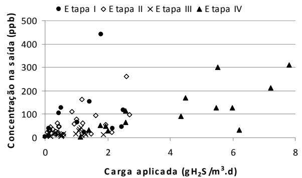
Figura 5.47: Relação da carga aplicada e da concentração de H 2 S na saída – filtro de cana.
