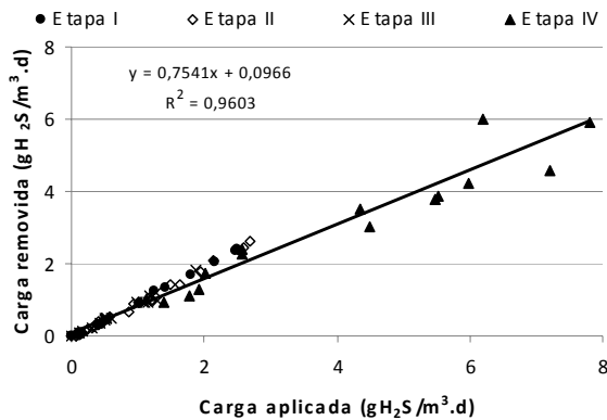
Figura 5.44: Eficiência de remoção com todas as etapas – filtro de solo.
