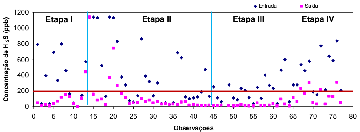
Figura 5.5: Medições feitas no biofiltro de bagaço de cana em todas as etapas.
