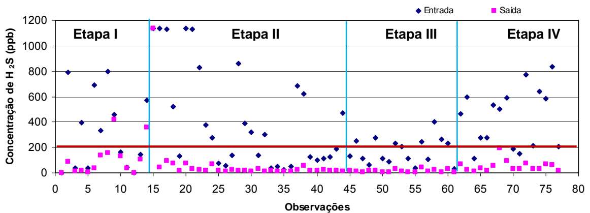
Figura 5.6: Medições feitas no biofiltro de palha de café + lodo em todas as etapas.
