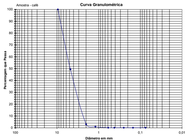
Curva granulométrica da palha de café.
