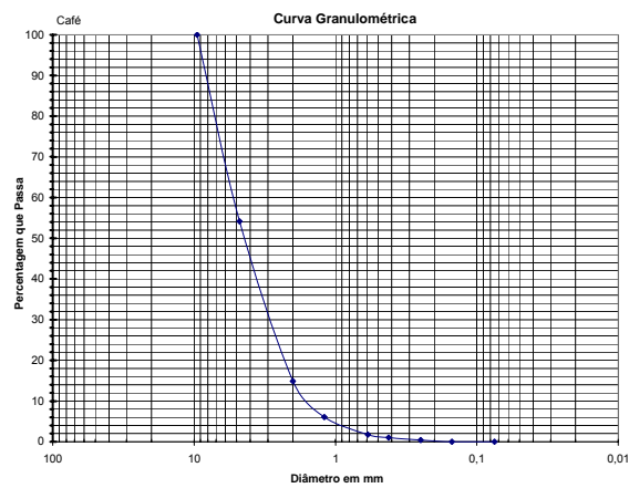
Curva granulométrica da palha de café.
