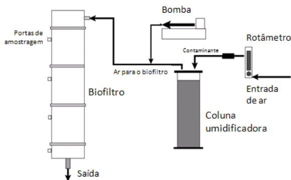
Figura 3.12: Esquema de umidificação utilizado por Morgan-Sagastume (2005).
