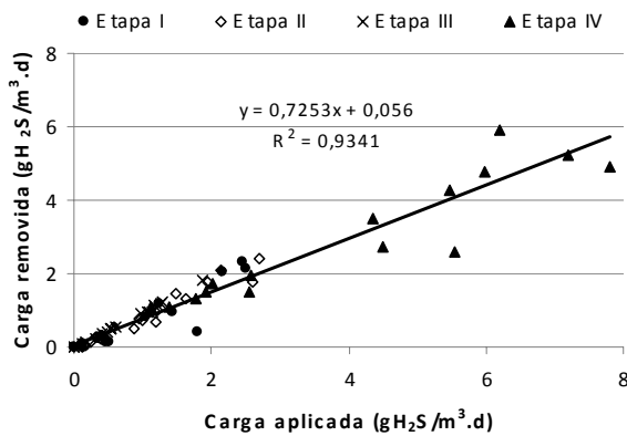
Figura 5.46: Eficiência de remoção com todas as etapas – filtro de cana.
