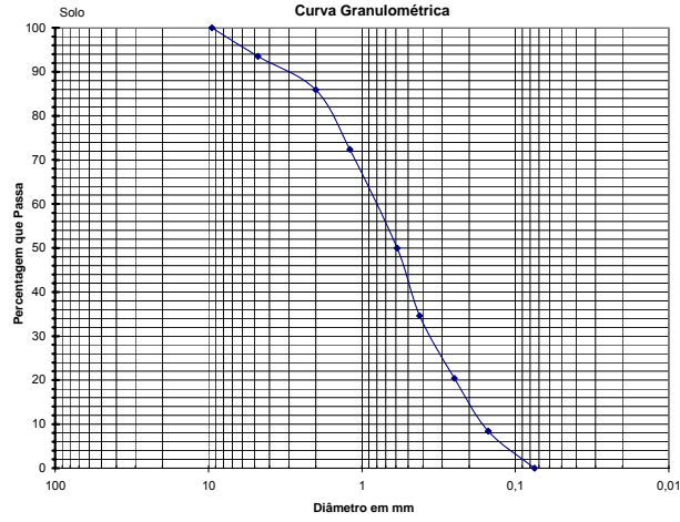
Curva granulométrica do solo.
