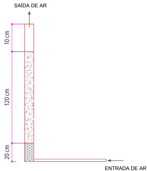
Figura 4.6: Esquema do biofiltro.
