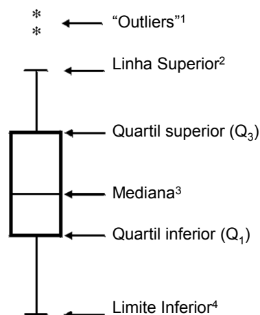
Figura 4.15: Gráfico de “box plot”.
