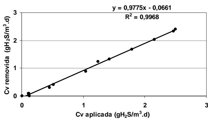
Figura 5.10: Eficiência de remoção no biofiltro de solo - etapa I.
