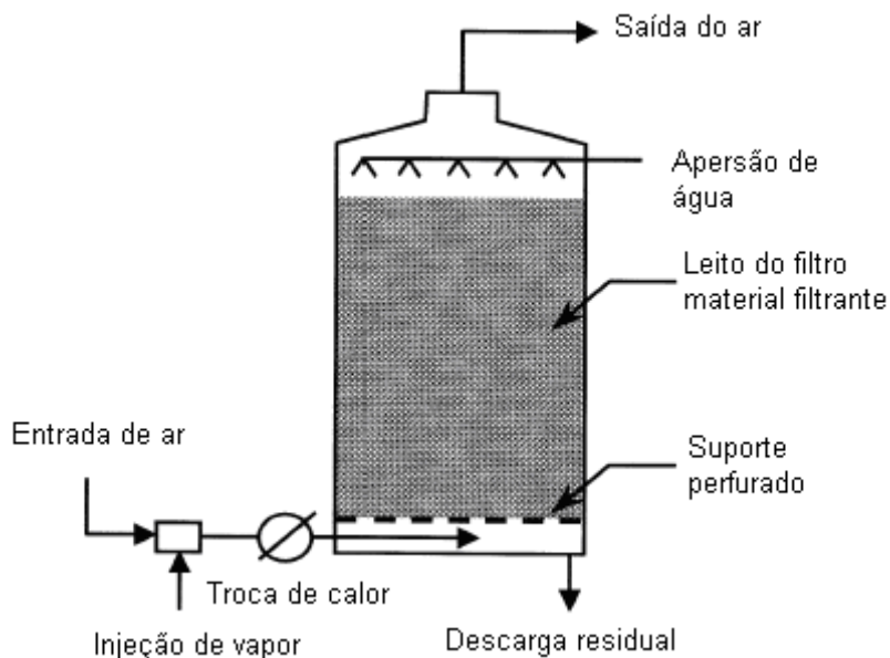
Figura 3.8: Esquema de um biofiltro fechado.
