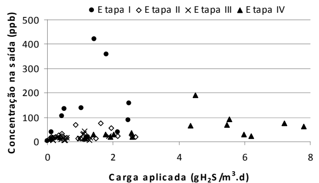
Figura 5.49: Relação da carga aplicada e da concentração de H 2 S na saída – filtro de café.
