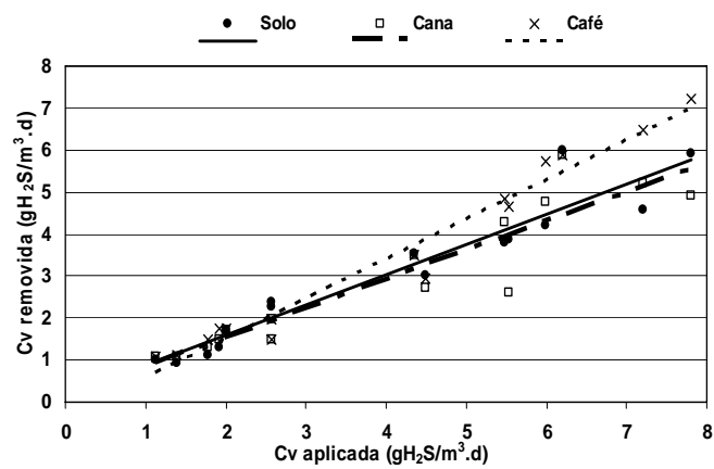
Figura 5.41: Eficiência de remoção nos três biofiltros - etapa IV.
