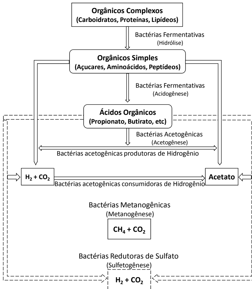
Figura 3.1: Seqüências metabólicas e grupos microbianos envolvidos na digestão anaeróbia (com redução de sulfato)
