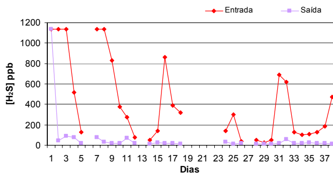
Figura 5.18: Monitoramento de \text{H}_2\text{S} no biofiltro de café - etapa II.
