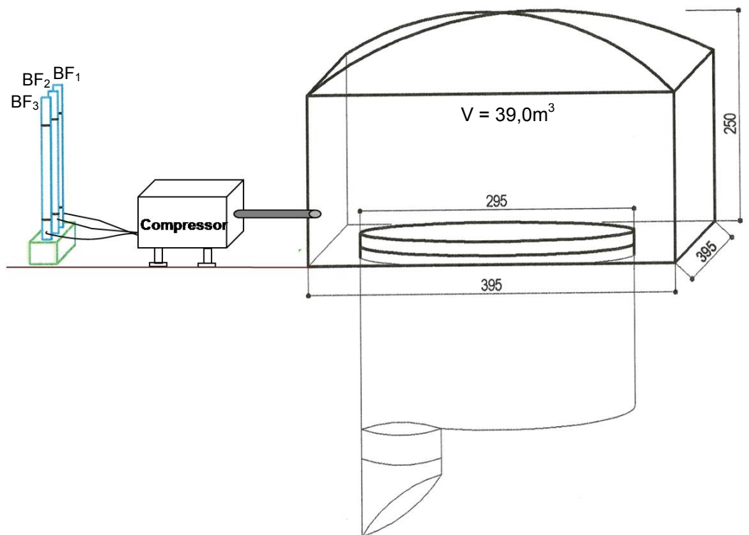
Figura 4.8: Esquema do sistema desodorizador - etapa I. Legenda: BF 1 = biofiltro de solo, BF 2 = biofiltro de cana, BF 3 = biofiltro de café.
