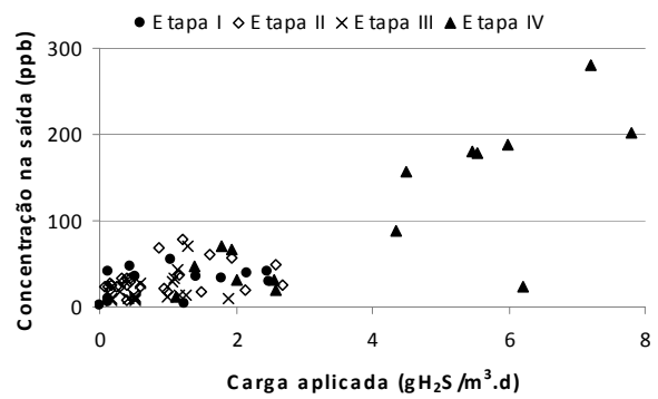
Figura 5.45: Relação da carga aplicada e da concentração de H 2 S na saída – filtro de solo.
