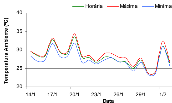
Figura 5.42: Acompanhamento da temperatura ambiente – etapa IV.
