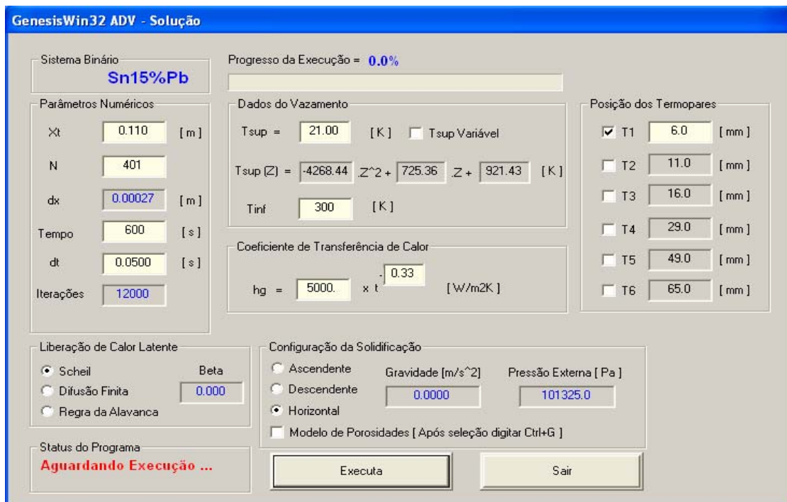
Figura 3.27: Tela de execução do programa utilizado neste trabalho com opções de escolha dos parâmetros de simulação, inserção dos dados de vazamento e valores de h_i para a liga Sn-15%Pb.
