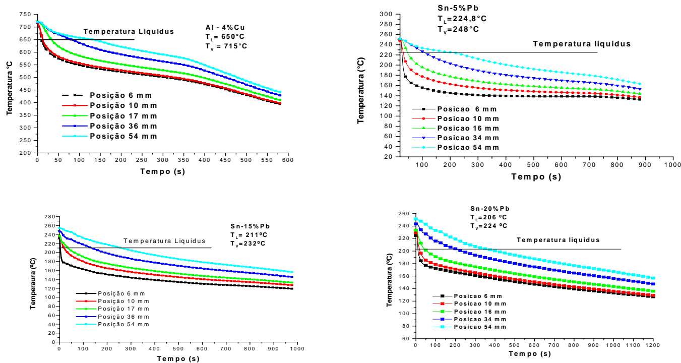
Figura 4.5: Variação da temperatura em função do tempo para cinco diferentes posições de termopares em relação à interface metal/molde das ligas estudadas neste trabalho.
