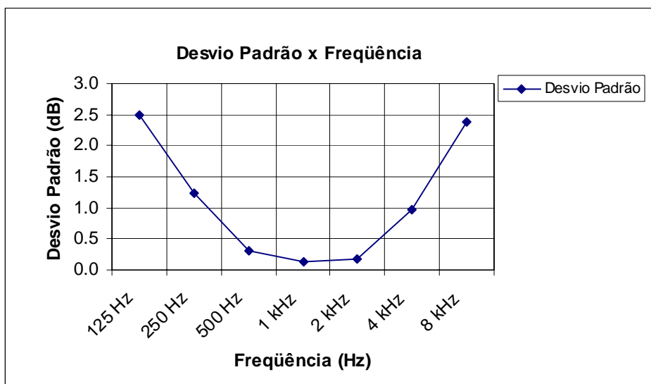
Figura 5.9 – Desvio Padrão das divisórias de fibra de aço.
