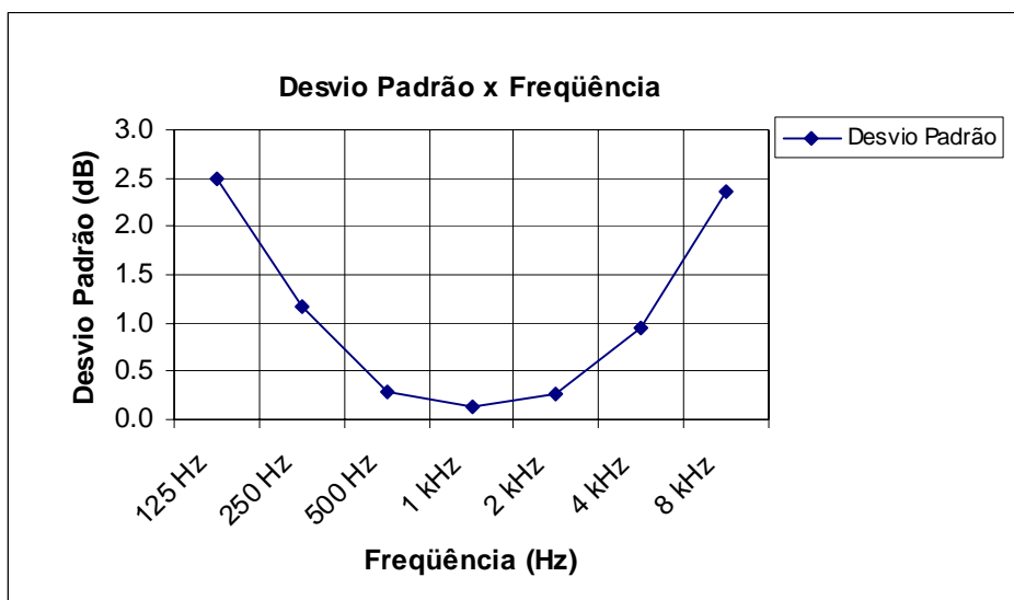
Figura 6.7 – Desvio Padrão das divisórias de fibra de aço.
