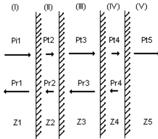
Figura 3.2: Configuração física do modelo matemático para parede dupla.
