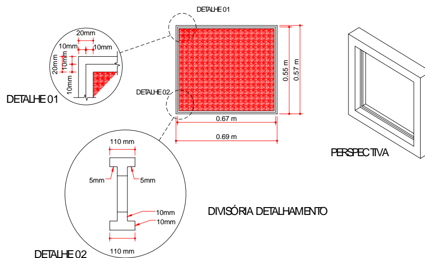
Figura 4.8 – Detalhamento da divisória.
