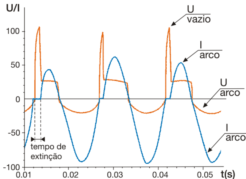
Figura 5 - Oscilogramas de tensão e corrente características de uma soldagem TIG CA do alumínio utilizando uma fonte de soldagem eletromagnética.
