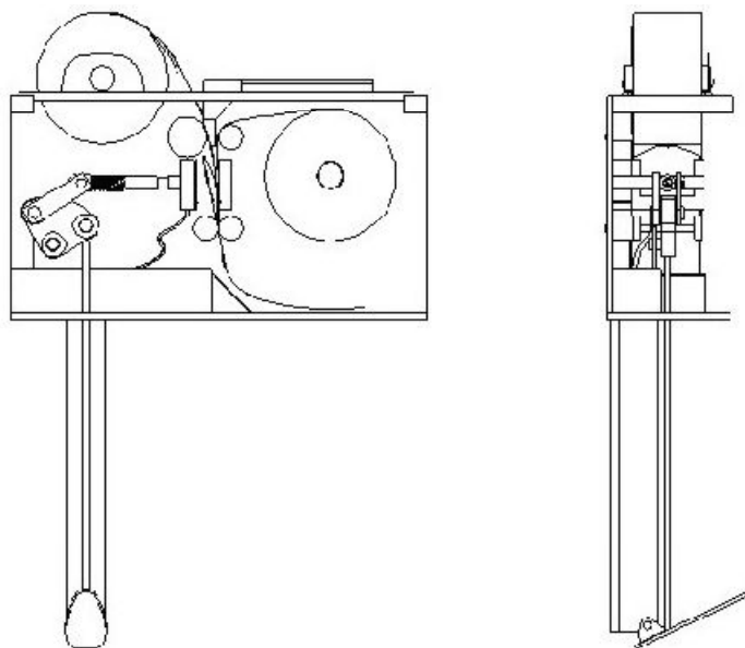
Figura 64 – Definição da arquitetura da embaladora de medicamentos
