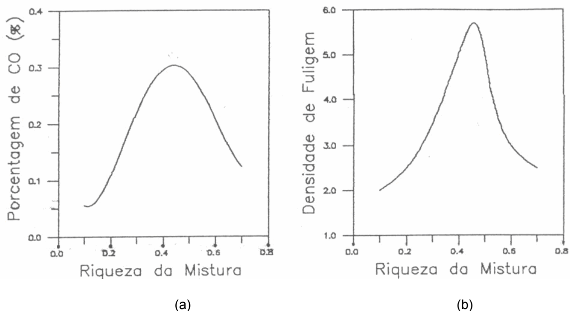
Figura 12 - Variação da composição do gás de escapamento de um motor Dual em função da riqueza global da mistura (ar-gás-diesel piloto).
