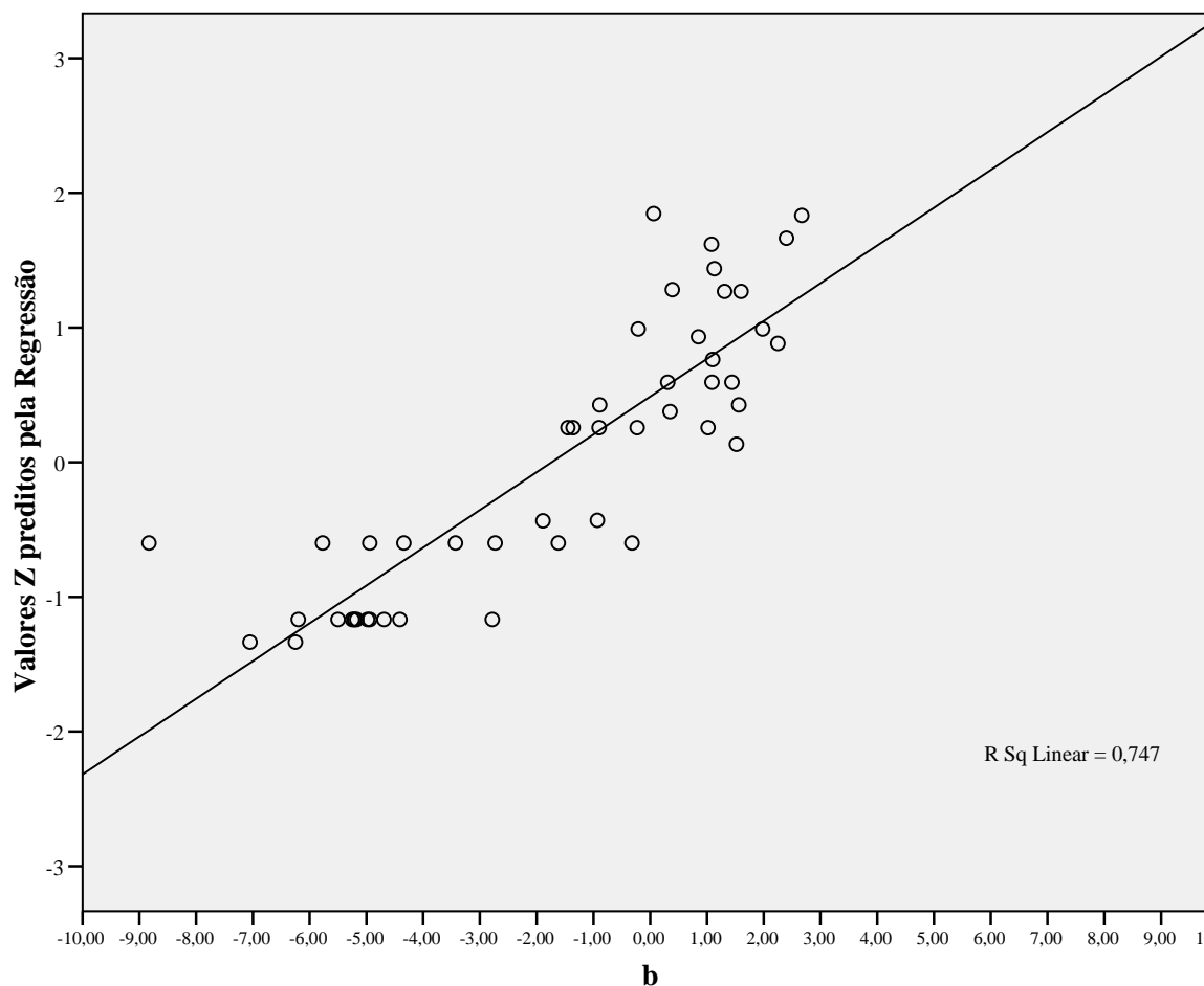
Figura 25. Gráfico de Dispersão da função de Regressão para prova RN.
