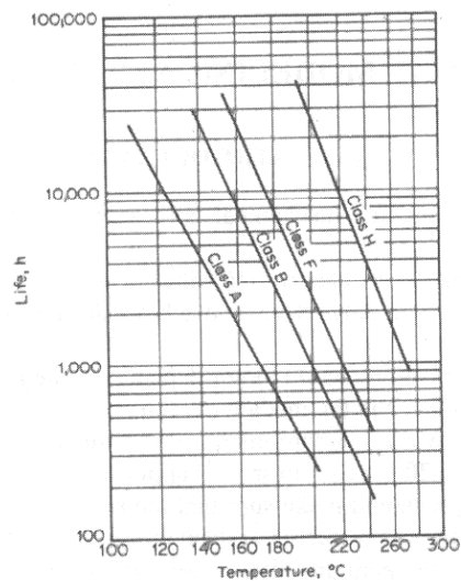
Figura 1.5 – Vida útil de um MI x Temperatura (Boldea, I., Nasar, S. A.; 2002).
