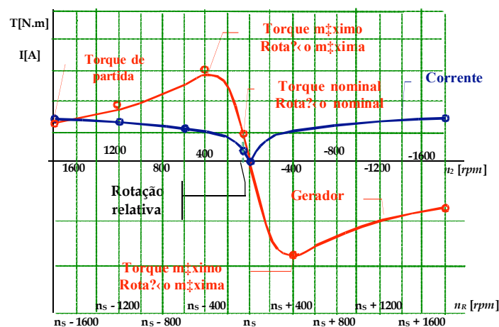
Figura 1. Comportamento do torque e da corrente para um motor de indução em relação à velocidade
