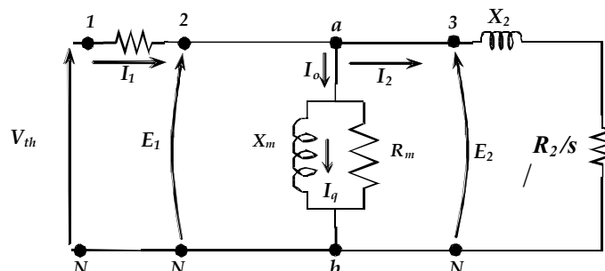
Figura 2. Circuito equivalente do motor de indução
