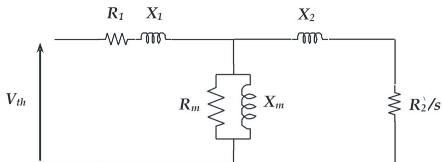
Figura 1 – Circuito equivalente de um MIT
