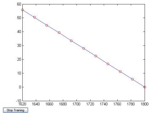
Figura 6. Resultados obtidos
