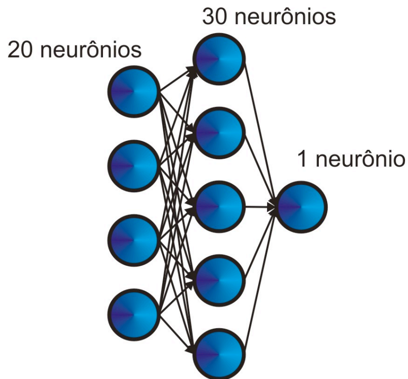
Figura 3.2 – RNA utilizada
