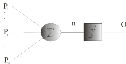
Figura 3. Neurônio artificial
