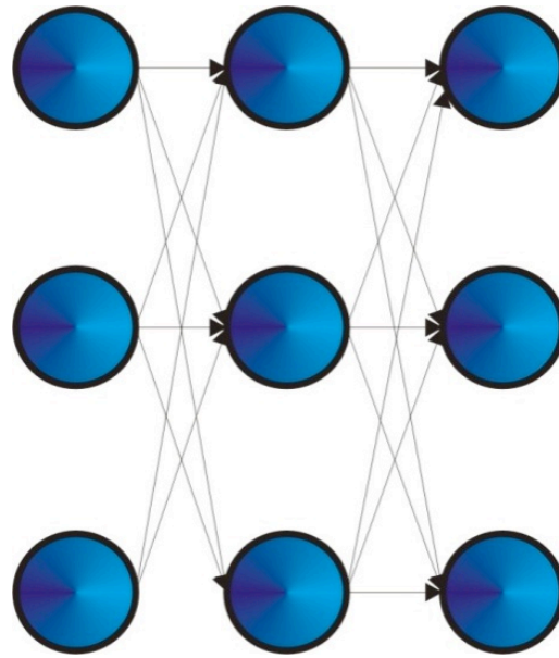
Figura 2.9 – Rede MADALINE
