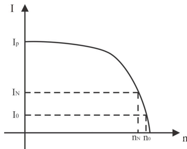
Figura 1.4 – Comportamento da corrente em relação à velocidade
