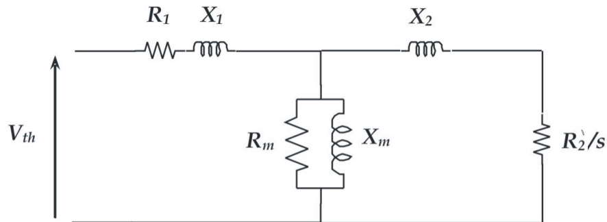
Figura 1.2 – Circuito equivalente de um motor de indução
