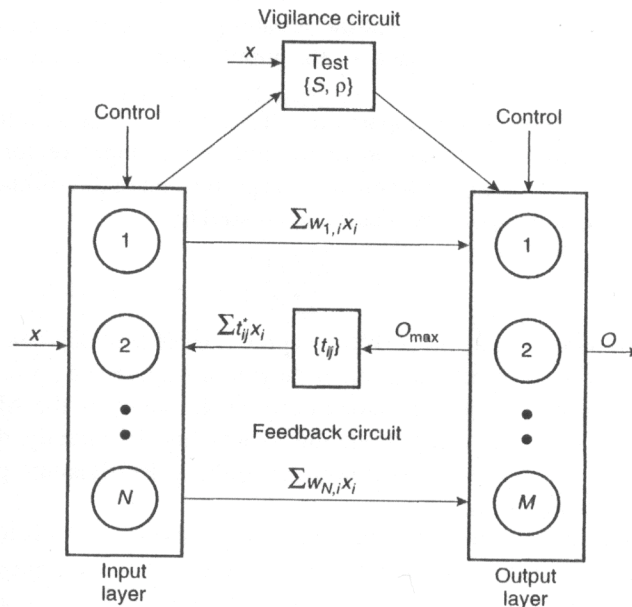
Figura 2.10 – Rede ART (Kartalopoulos, S.; 1996).
