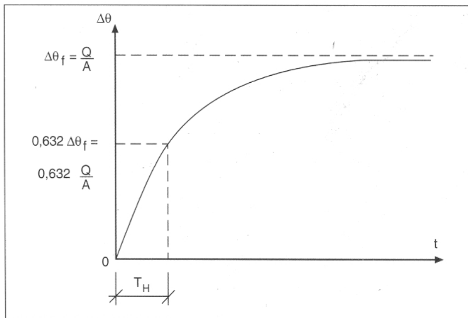
Figura 1.6 – Comportamento térmico durante a aceleração de um motor de indução (Costa, P. F., Borel, J. E. V.; 1999).
