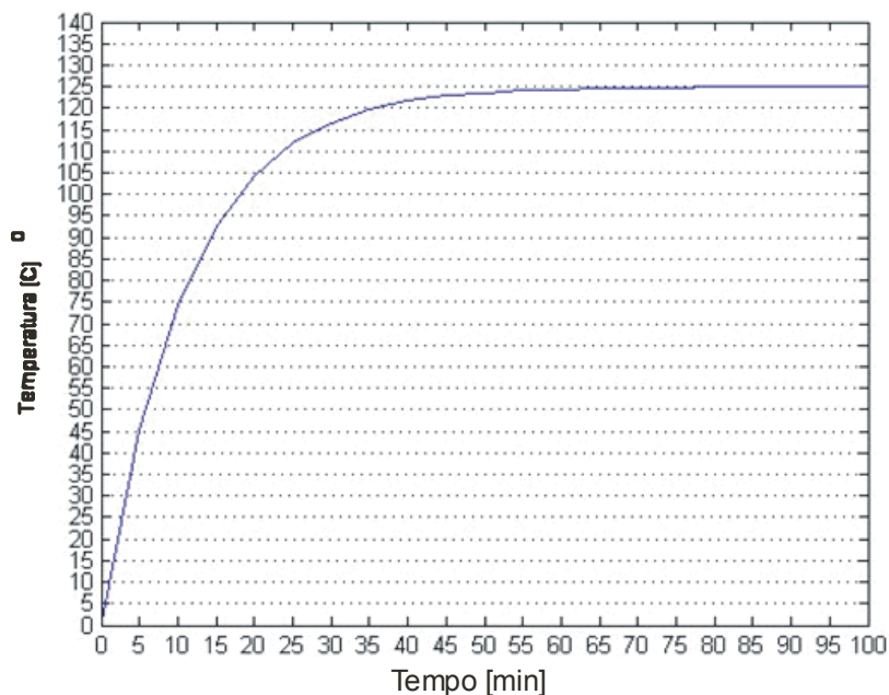
Figura 3.1 – Curva da elevação de temperatura para o motor analisado.
