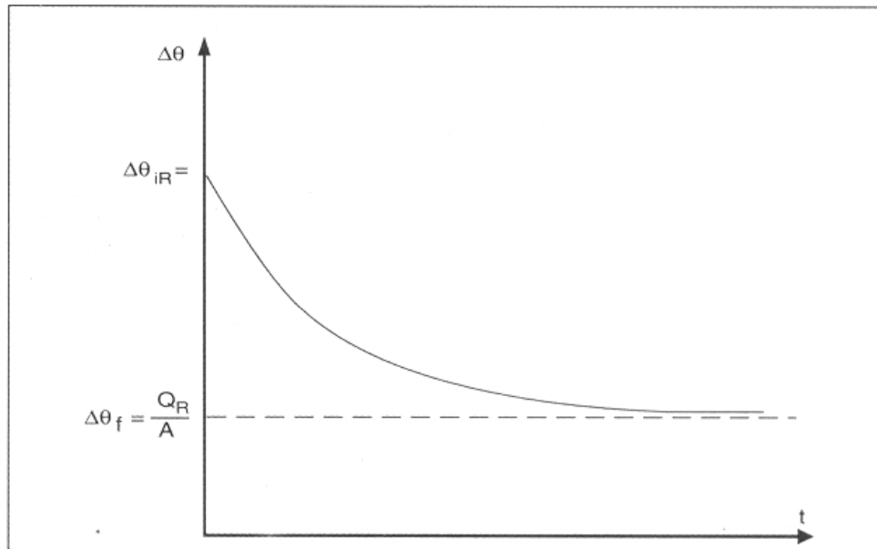
Figura 1.7 – Comportamento térmico durante a frenagem de um motor de indução (Costa, P. F., Borel, J. E. V.; 1999).
