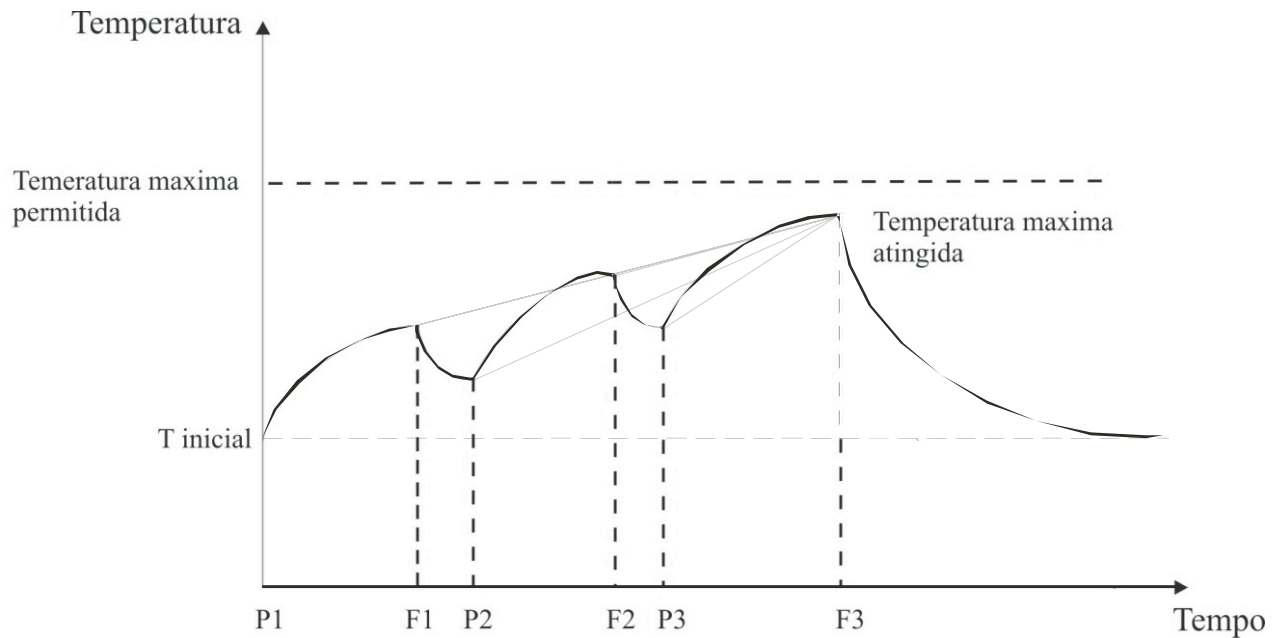
Figura 1.8 – Comportamento térmico de um motor durante um ciclo de operação.
