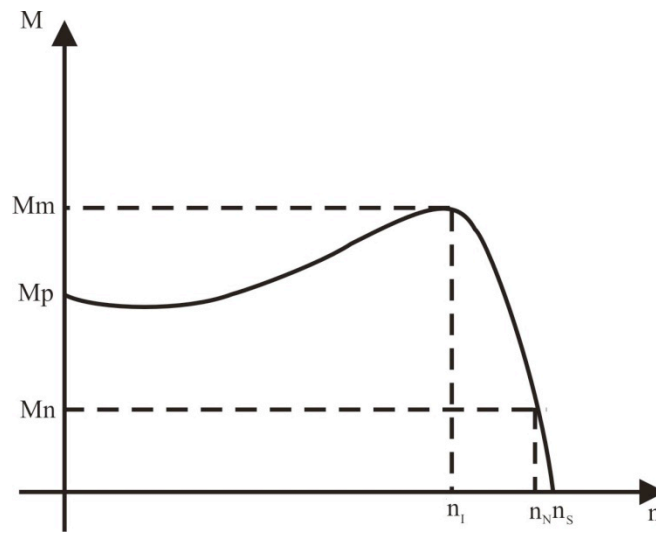
Figura 1.3 – Conjugado em relação à velocidade
