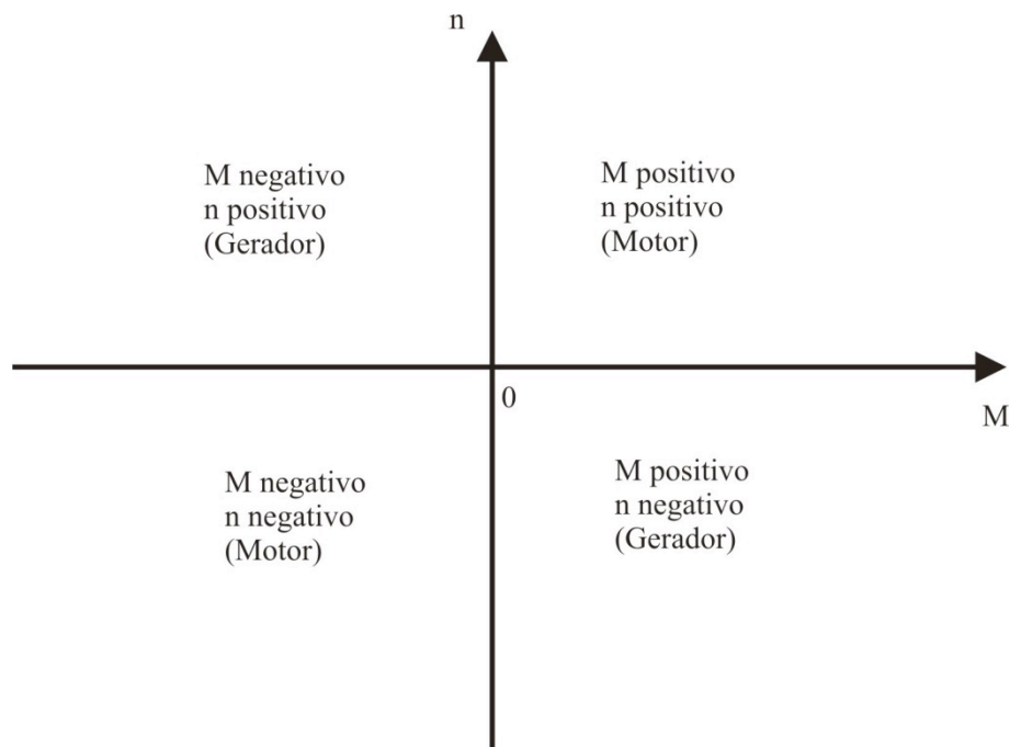
Figura 1.1 – Condições de operação nos quatro quadrantes
