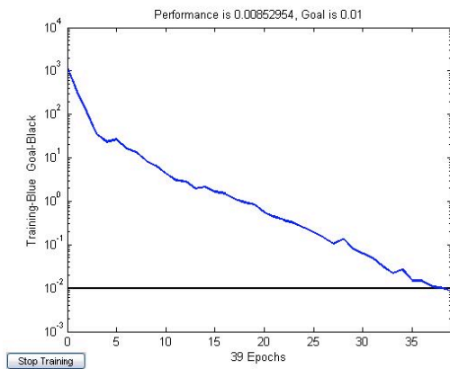
Figura 5. Desempenho da rede
