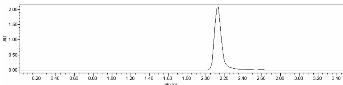
Figura 6.4.8: Cromatograma da solução de cloridrato de ciprofloxacino SQR com concentração de 100,0 \mu\text{g/mL} , utilizando ácido acético 5,0% v/v, ACN e MetOH (70:15:15, v/v/v) como fase móvel e solvente e coluna Waters.
