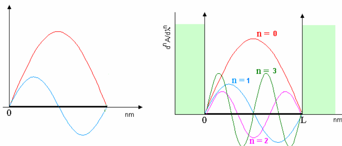
Figura 6.3.1: Representação esquemática das derivadas.
