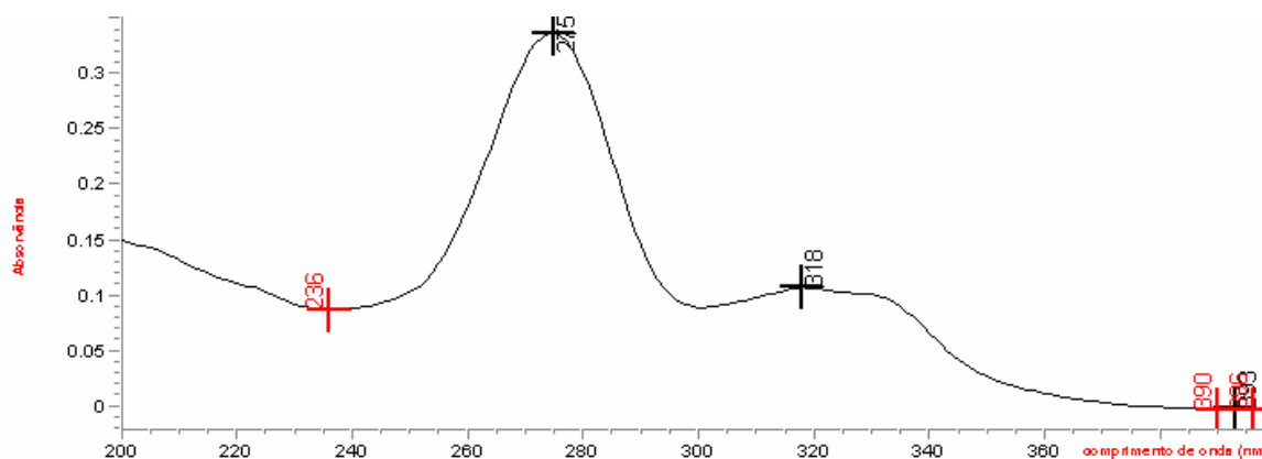
Figura 5.1.1: Espectro de absorção da solução de cloridrato de ciprofloxacino SQR com concentração de 4,0 \mu\text{g/mL} , na região do ultravioleta, utilizando água como solvente.
