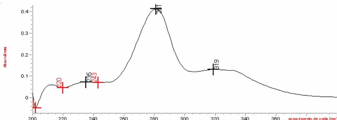
Figura 5.1.2: Espectro de absorção da solução de cloridrato de ciprofloxacino SQR com concentração de 4,0 \mu\text{g/mL} , na região do ultravioleta, utilizando metanol como solvente.
