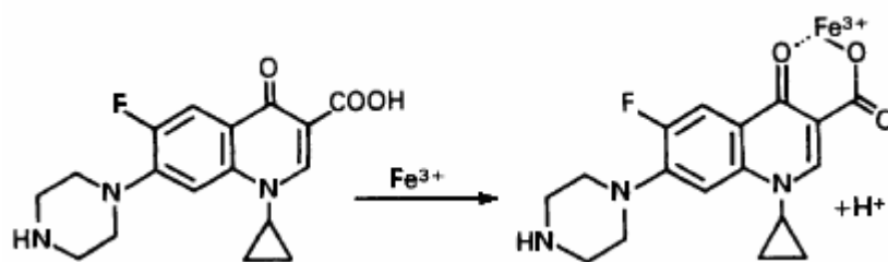
Figura 5.2.1: Reação do ferro (III) com ciprofloxacino.
