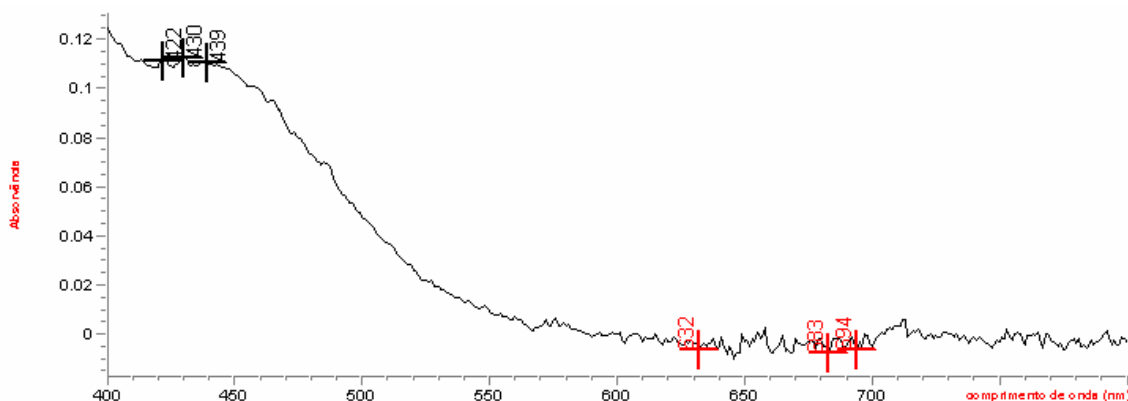
Figura 5.2.2: Espectro de absorção da solução de cloridrato de ciprofloxacino SQR com concentração de 20,0 µg/mL, na região do visível, utilizando água como solvente e cloreto férrico 1,0% como reagente.
