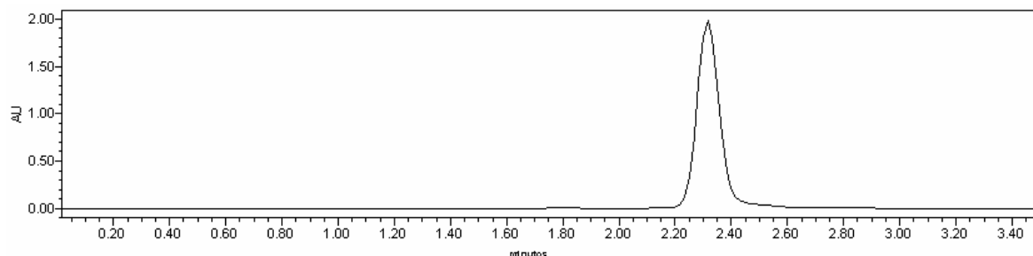
Figura 6.4.6: Cromatograma da solução de cloridrato de ciprofloxacino SQR com concentração de 100,0 \mu\text{g/mL} , utilizando ácido acético 2,5% v/v, ACN e MetOH (70:15:15, v/v/v) como fase móvel e solvente e coluna Waters.
