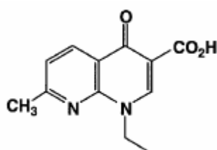
Figura 3.1.1: Estrutura química do ácido nalidíxico.
