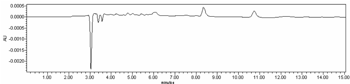
Figura 6.4.2: Cromatograma da solução de cloridrato de ciprofloxacino SQR com concentração de 100,0 \mu\text{g/mL} , utilizando ácido acético 1,0% v/v, ACN e MetOH (70:15:15, v/v/v) como fase móvel e solvente e coluna Thermo.
