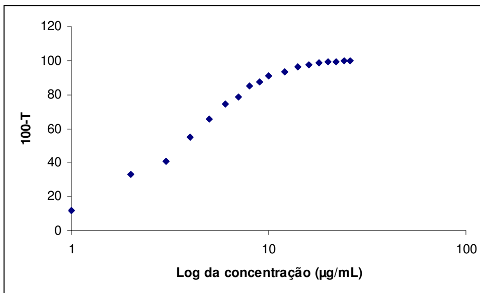
Figura 6.2.1: Curva de Ringbom obtida pelo método espectrofotométrico na região do UV para cloridrato de ciprofloxacino SQR, utilizando água como solvente no comprimento de onda de 275 nm.
