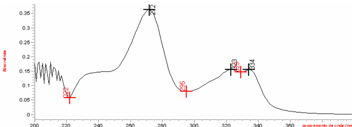
Figura 5.1.4: Espectro de absorção de solução de cloridrato de ciprofloxacino SQR com concentração de 4,0 \mu\text{g/mL} , na região do ultravioleta, utilizando hidróxido de sódio 0,1 M como solvente.
