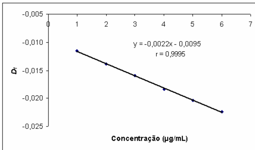
Figura 6.3.5: Curva analítica de cloridrato de ciprofloxacino SQR, obtida pelo método espectrofotométrico derivativo na região do visível, utilizando cloreto férrico 1,0% como reagente a 386,4 nm, na primeira derivada.
