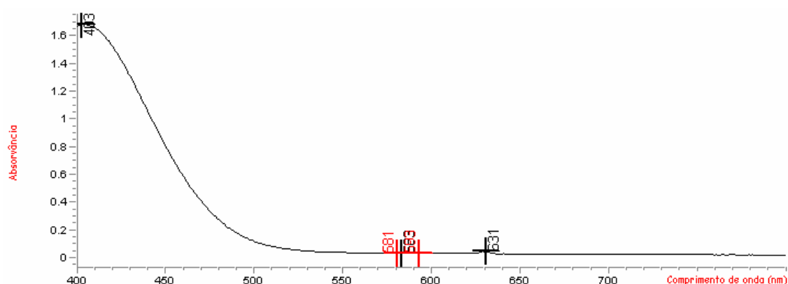
Figura 5.2.6: Espectro de absorção da solução de cloridrato de ciprofloxacino SQR com concentração de 20,0 µg/mL, na região do visível, utilizando éter etílico como solvente e azul de bromotimol como reagente.
