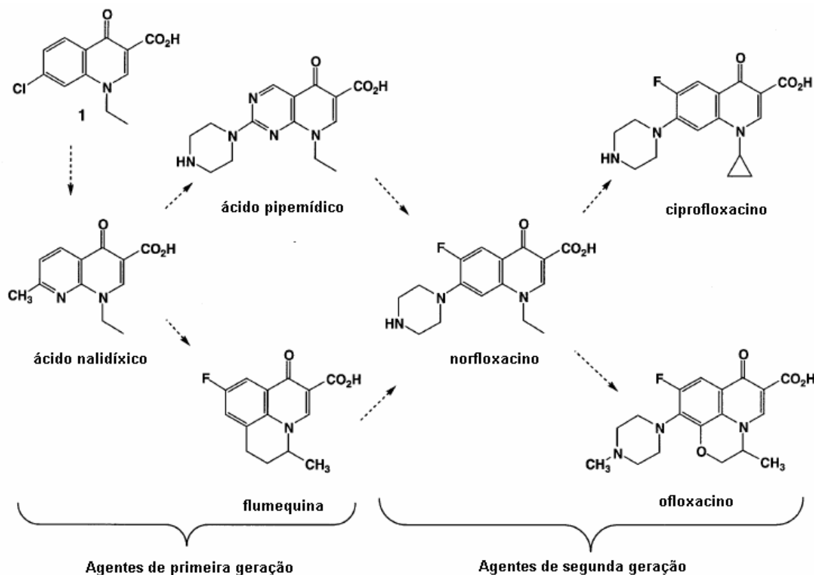
Figura 3.1.2: Evolução histórica das quinolonas.
