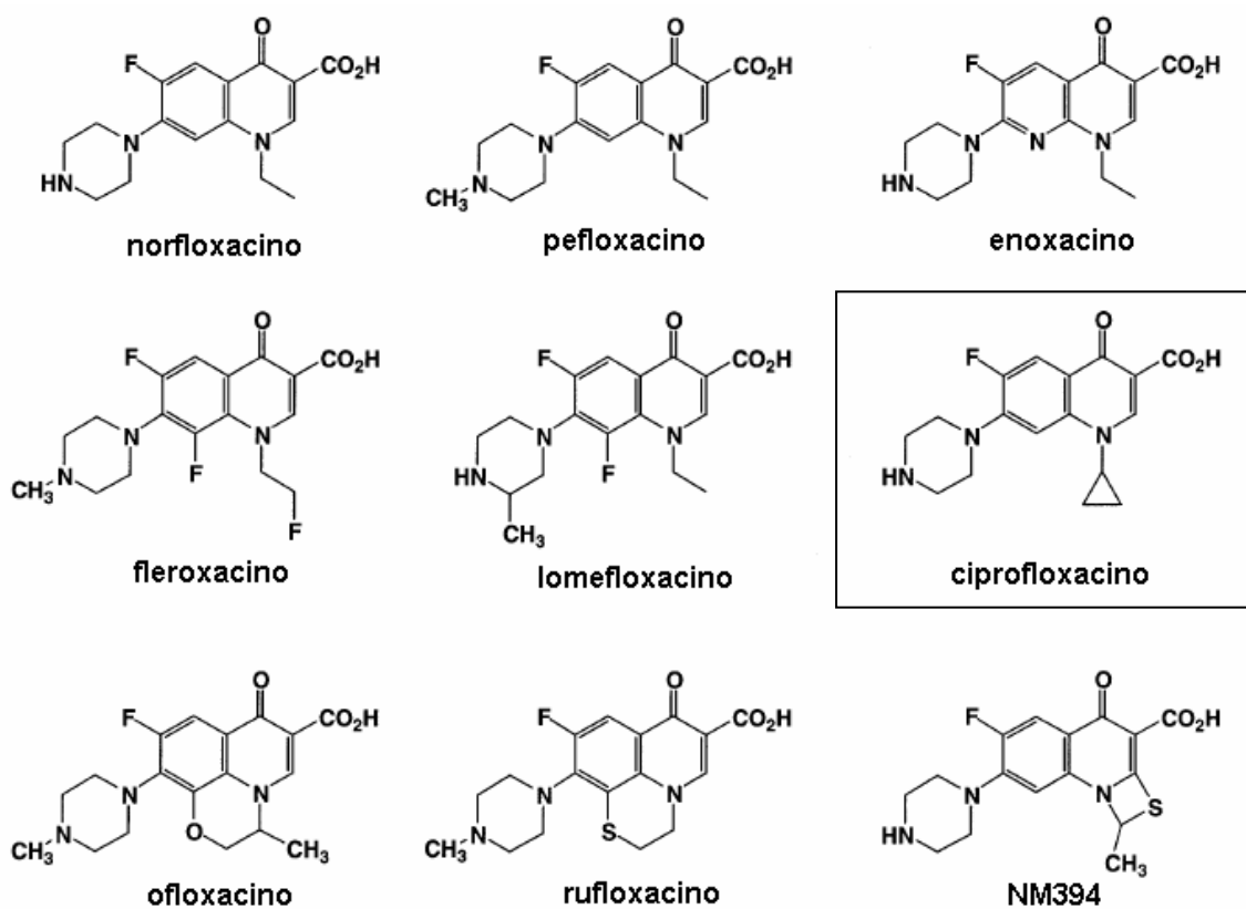
Figura 3.1.4: Quinolonas de segunda geração.
