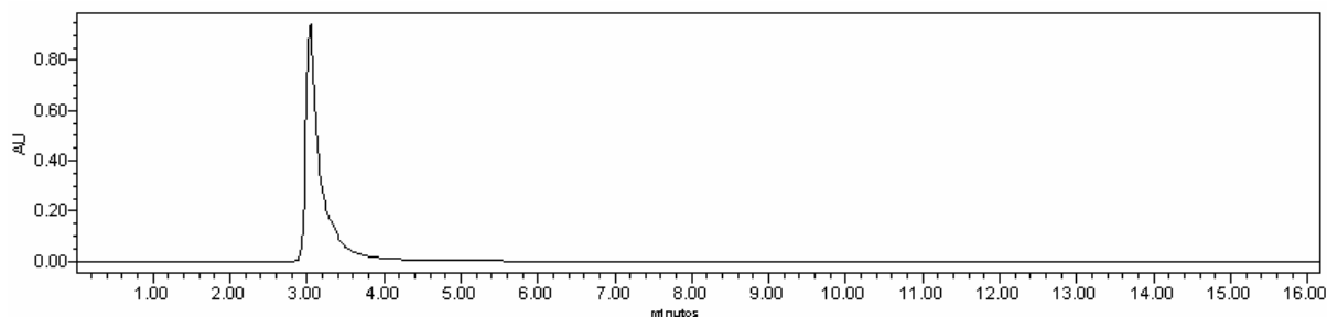
Figura 6.4.3: Cromatograma da solução de cloridrato de ciprofloxacino SQR com concentração de 100,0 \mu\text{g/mL} , utilizando água como solvente, ácido acético 1,0% v/v, ACN e MetOH (70:15:15, v/v/v) como fase móvel e coluna Waters.
