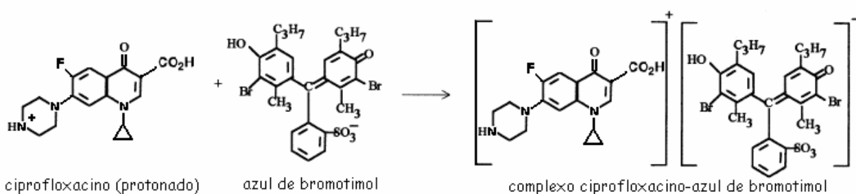
Figura 5.2.3: Esquema da reação entre o ciprofloxacino e o azul de bromotimol.
