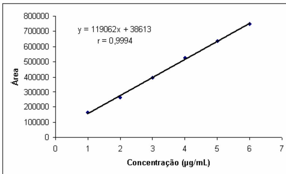
Figura 6.4.9: Curva analítica de cloridrato de ciprofloxacino SQR obtida pelo método cromatográfico, utilizando água como solvente e como fase móvel ácido acético 2,5% v/v, acetonitrila e metanol (70:15:15, v/v/v) a 275 nm.
