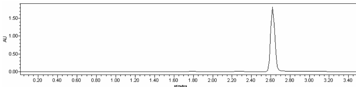
Figura 6.4.5: Cromatograma da solução de cloridrato de ciprofloxacino SQR com concentração de 100,0 \mu\text{g/mL} , utilizando água como solvente, ácido acético 2,5% v/v, ACN e MetOH (70:15:15, v/v/v) como fase móvel e coluna Waters.
