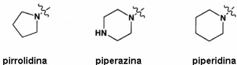
Figura 3.1.8: Substituintes comuns nas estruturas quinolônicas.
