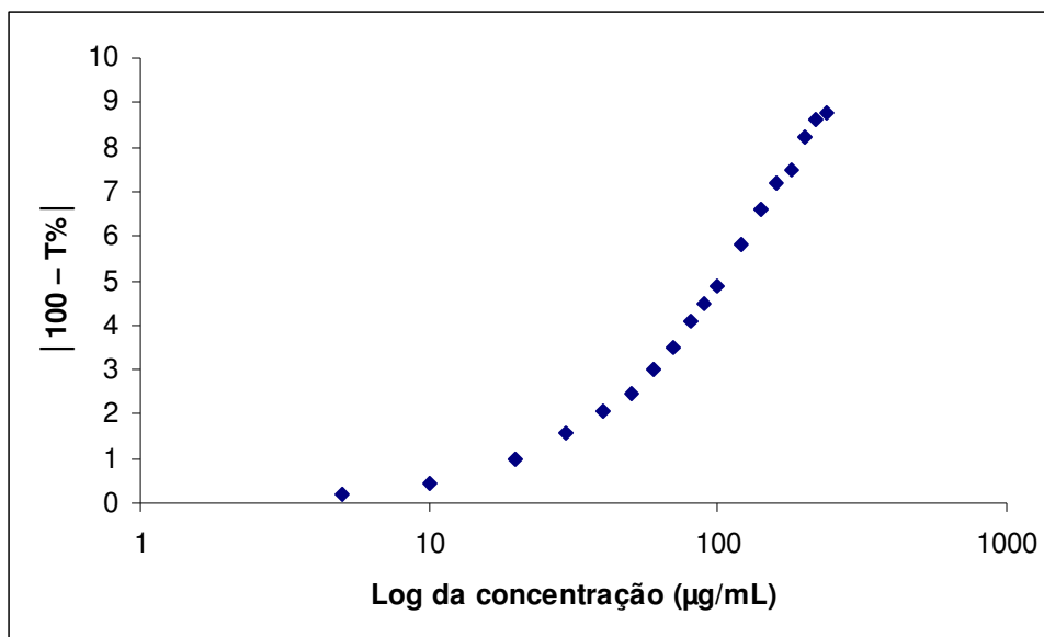
Figura 6.3.4: Curva de Ringbom obtida pelo método espectrofotométrico derivativo na região do visível para cloridrato de ciprofloxacino SQR, utilizando cloreto férrico 1,0% como reagente no comprimento de onda de 386,4 nm, na primeira derivada.
