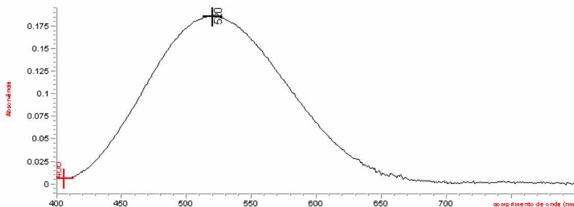
Figura 5.2.8: Espectro de absorção da solução de cloridrato de ciprofloxacino SQR com concentração de 60,0 µg/mL, na região do visível, utilizando acetonitrila como solvente e ácido cloranílico como reagente.
