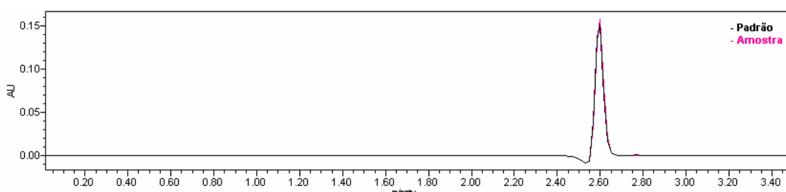
Figura 6.4.10: Sobreposição de cromatogramas de cloridrato de ciprofloxacino SQR e solução oftálmica, nas mesmas concentrações (10 µg/mL), para comprovação da especificidade do método CLAE.
