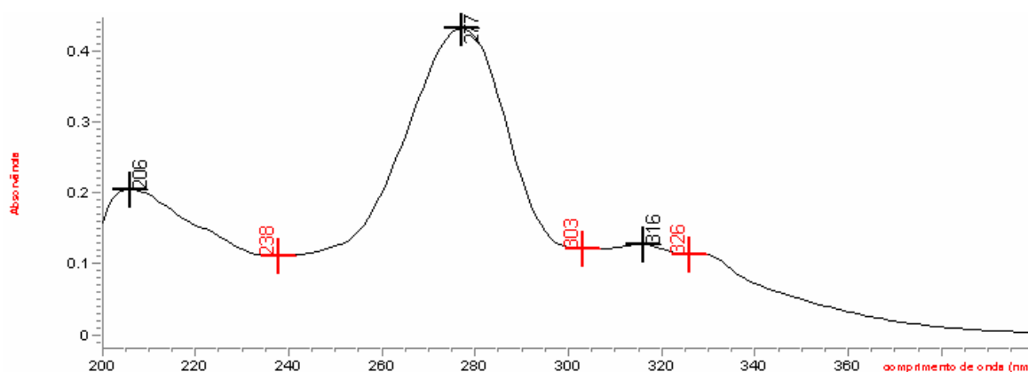
Figura 5.1.3: Espectro de absorção da solução de cloridrato de ciprofloxacino SQR com concentração de 4,0 \mu\text{g/mL} , na região do ultravioleta, utilizando ácido clorídrico 0,1 M como solvente.
