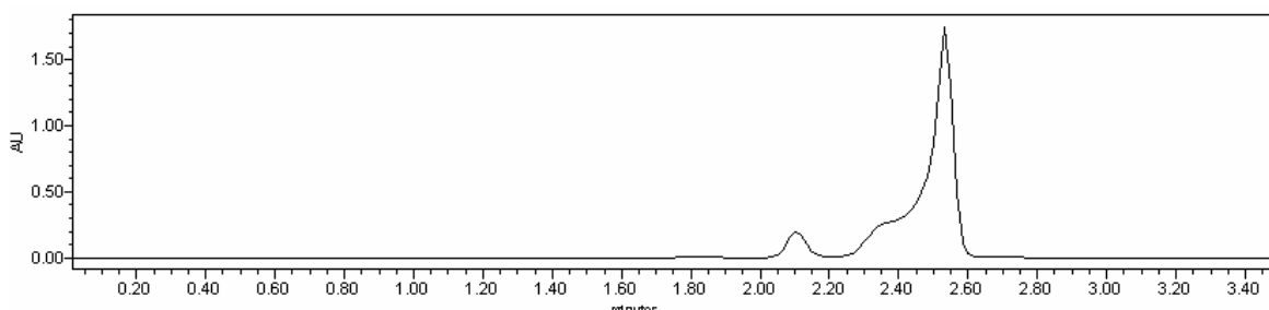
Figura 6.4.7: Cromatograma da solução de cloridrato de ciprofloxacino SQR com concentração de 100,0 \mu\text{g/mL} , utilizando água como solvente, ácido acético 5,0% v/v, ACN e MetOH (70:15:15, v/v/v) como fase móvel e coluna Waters.
