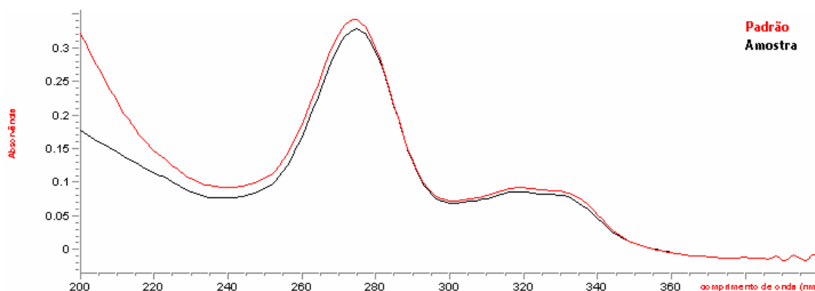
Figura 6.2.3: Sobreposição dos espectros de cloridrato de ciprofloxacino SQR e solução oftálmica, nas mesmas concentrações (4µg/mL), para determinação da especificidade do método espectrofotométrico na região do UV.
