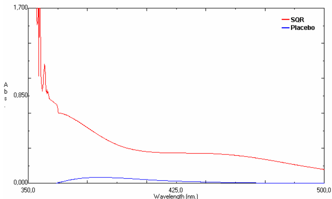
Figura 6.3.2: Espectro de ordem zero da solução de cloridrato de ciprofloxacino SQR (50,0 \mu\text{g/mL} ) e da solução placebo da solução oftálmica reagindo com cloreto férrico 1,0%.
