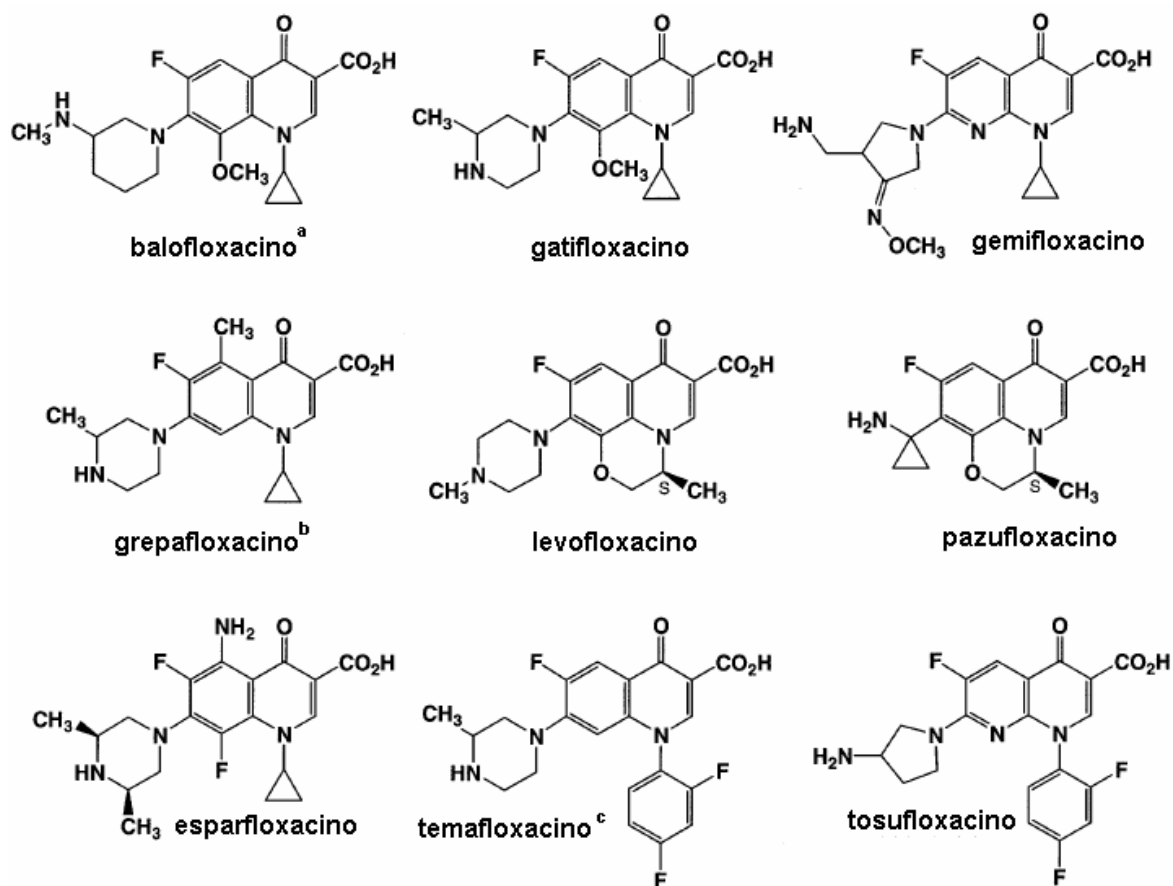
Figura 3.1.5: Quinolonas de terceira geração.
