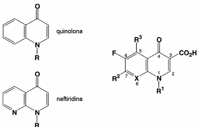
Figura 3.1.7: Núcleo quinolona e naftiridina: características da estrutura geral requerida para atividade antibacteriana.
