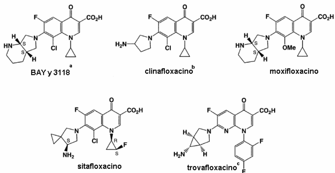
Figura 3.1.6: Quinolonas de quarta geração.
