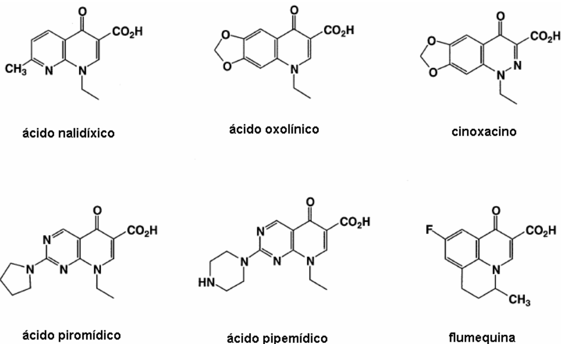
Figura 3.1.3: Quinolonas de primeira geração.
