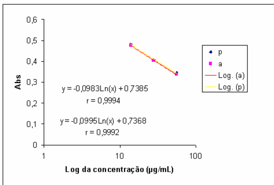
Figura 6.1.1: Curvas analíticas de soluções de cloridrato de ciprofloxacino SQR e amostra, em concentrações de 14,0; 28,0 e 56,0 µg/mL, obtidas pelo método turbidimétrico.
