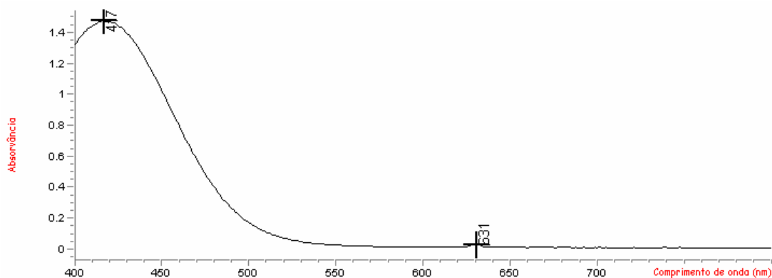
Figura 5.2.5: Espectro de absorção da solução de cloridrato de ciprofloxacino SQR com concentração de 20,0 µg/mL, na região do visível, utilizando clorofórmio como solvente e azul de bromotimol como reagente.
