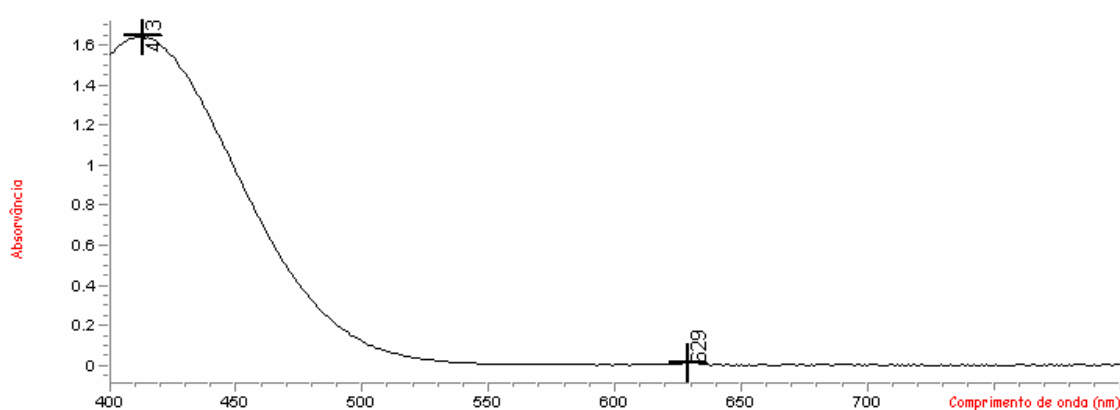
Figura 5.2.4: Espectro de absorção da solução de cloridrato de ciprofloxacino SQR com concentração de 20,0 µg/mL, na região do visível, utilizando diclorometano como solvente e azul de bromotimol como reagente.
