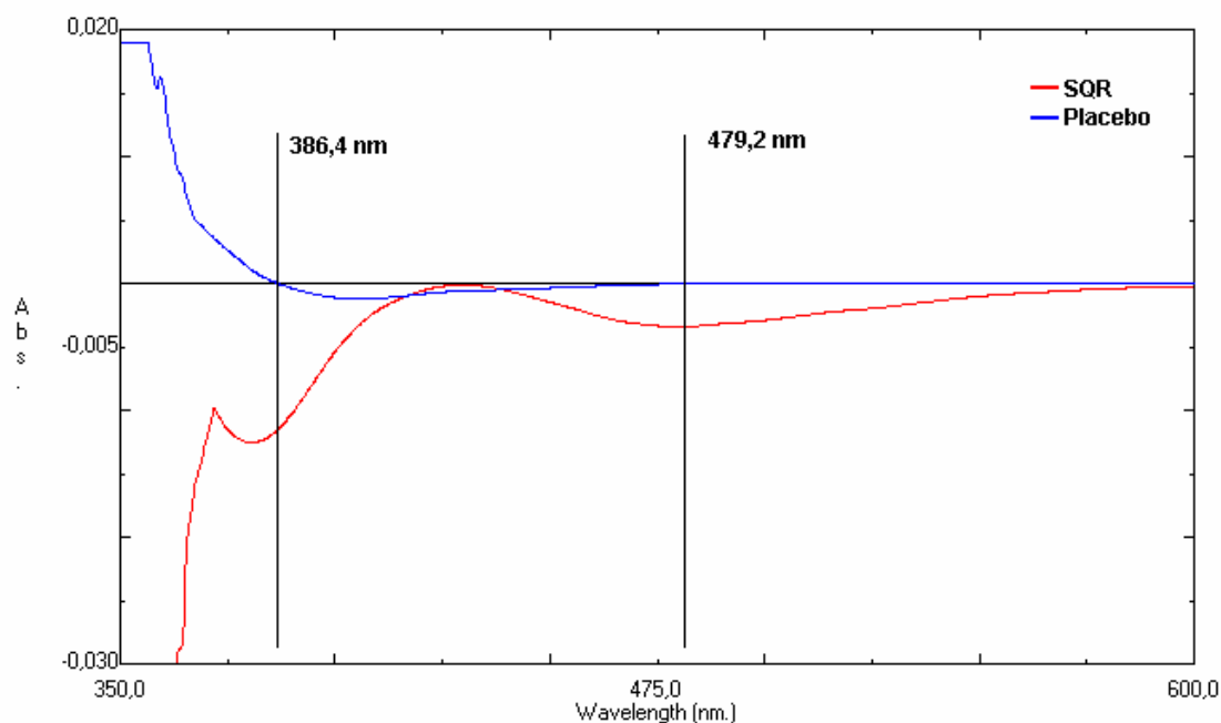
Figura 6.3.3: Espectro de primeira ordem da solução de cloridrato de ciprofloxacino SQR (50,0 µg/mL) e da solução placebo da solução oftálmica reagindo com cloreto férrico 1,0%.
