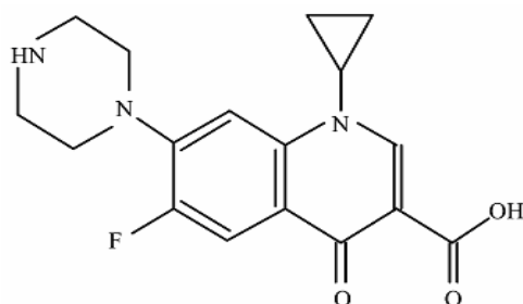
Figura 4.1.1: Estrutura química do ciprofloxacino.
