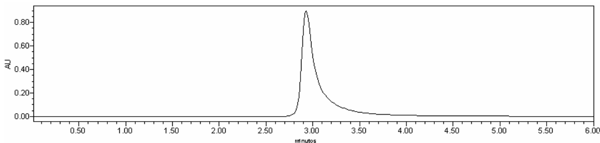
Figura 6.4.4: Cromatograma da solução de cloridrato de ciprofloxacino SQR com concentração de 100,0 \mu\text{g/mL} , utilizando ácido acético 1,0% v/v, ACN e MetOH (70:15:15, v/v/v) como fase móvel e solvente e coluna Waters.
