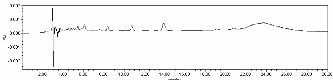
Figura 6.4.1: Cromatograma da solução de cloridrato de ciprofloxacino SQR com concentração de 100,0 \mu\text{g/mL} , utilizando água como solvente, ácido acético 1,0% v/v, ACN e MetOH (70:15:15, v/v/v) como fase móvel e coluna Thermo.
