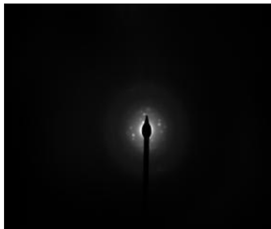
Figura 33: Padrão de difração de elétrons do suporte HBC
