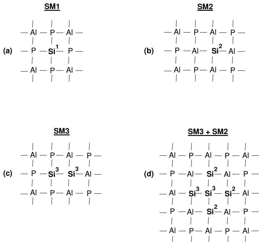
Figura 12: Princípio da introdução de silício na estrutura de um \text{ALPO}_4
