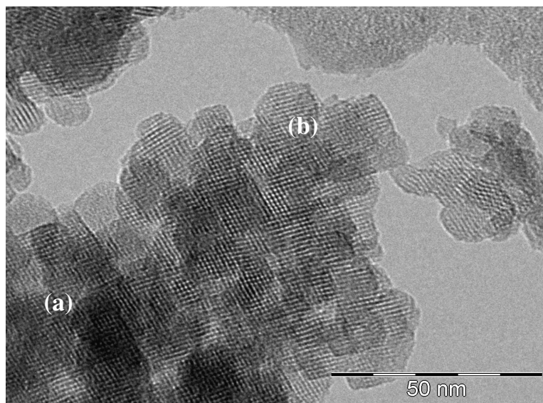
Figura 59: Microscopia eletrônica transmissão do catalisador HBC NM02
