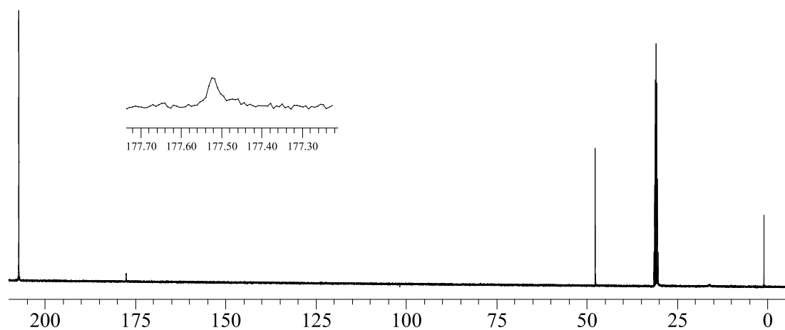
Figura 20. Espectro de RMN de ^{13}\text{C} em \text{acetona-}d_6 do composto \text{Br}_3\text{InCH}_2\text{Et} , 6.
