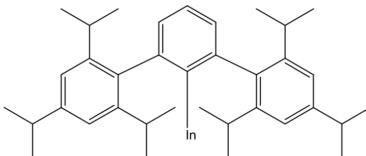
Figura 1. Estrutura do composto \text{In}(\text{C}_6\text{H}_3\text{-2,6-Trip}_2) .
