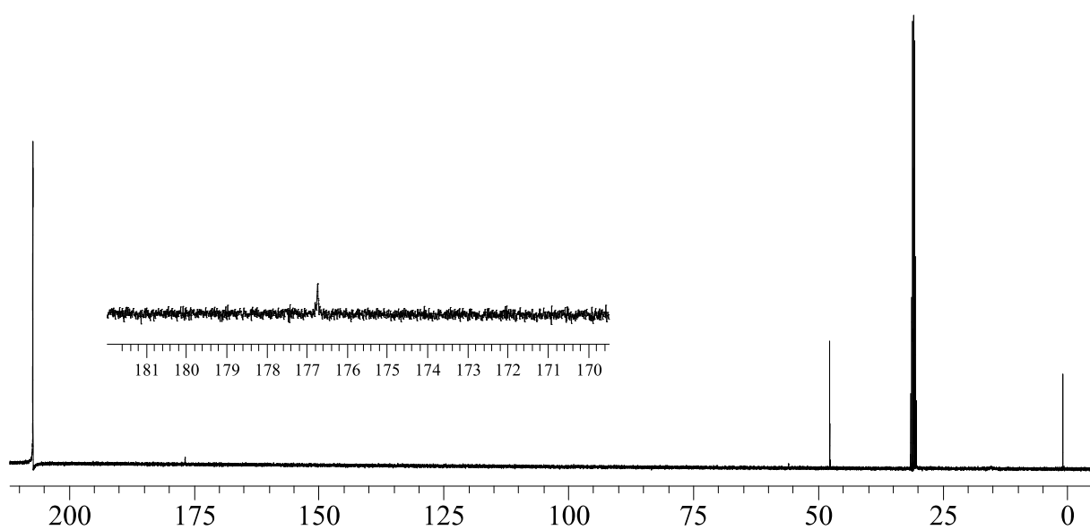
Figura 22. Espectro de RMN de ^{13}C em acetona- d_6 do composto I_3InCH_2Et , 5.
