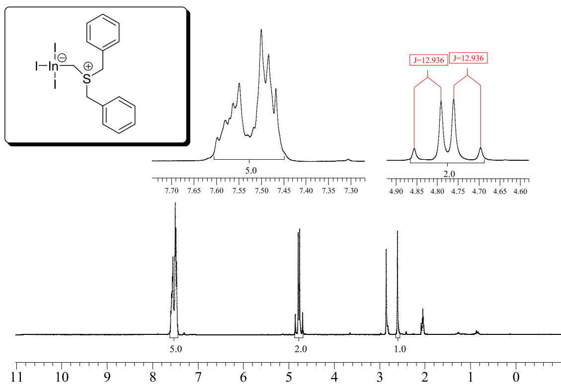
Figura 17. Espectro de RMN de ^1H em acetona- d_6 do composto I_3InCH_2S(CH_2Ph)_2 , 3.
