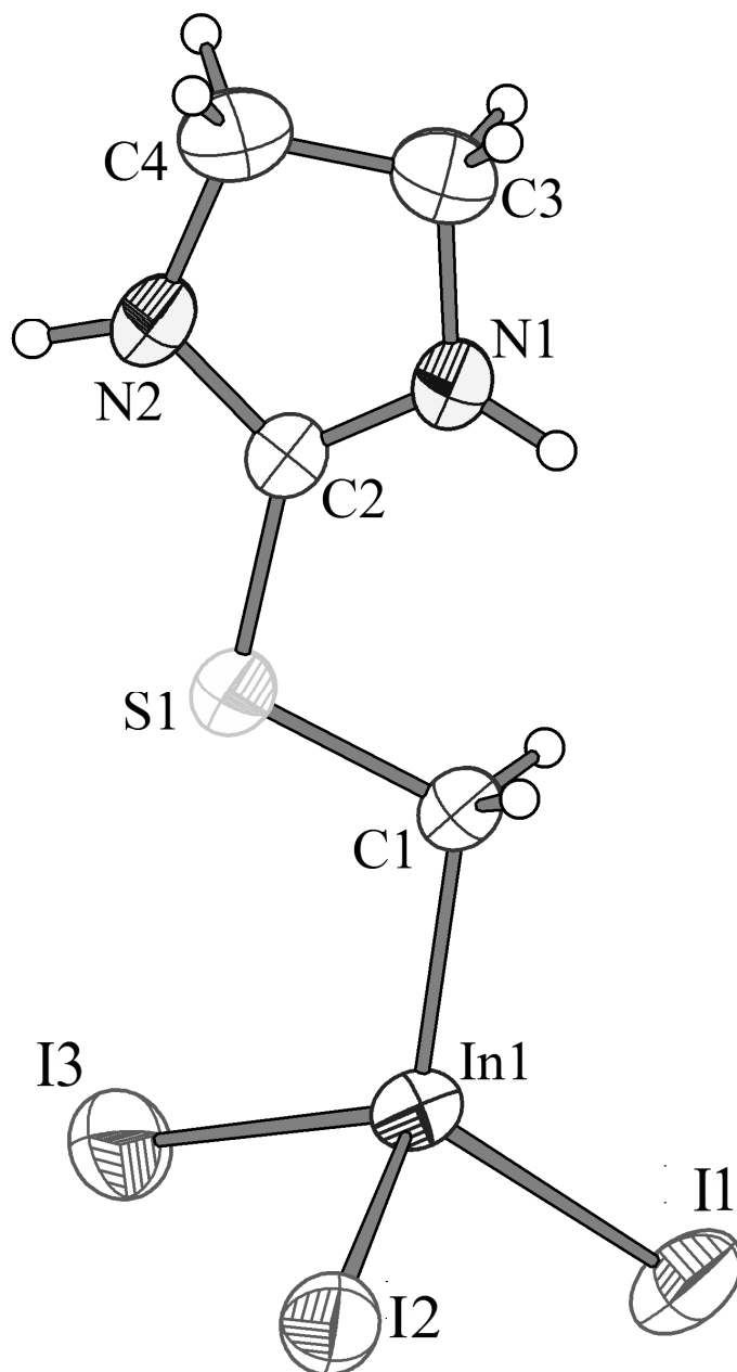
Figura 11. Estrutura molecular do Metilto de etilenotiorônio-triiodo-índio(III), 7. As elipsóides termais foram desenhadas com nível de probabilidade de 50%.
