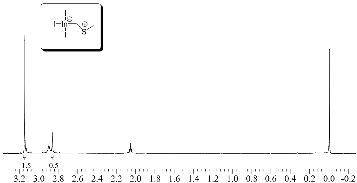
Figura 15. Espectro de RMN de ^1H em acetona- d_6 do composto I_3InCH_2S(CH_3)_2 , 2 .
