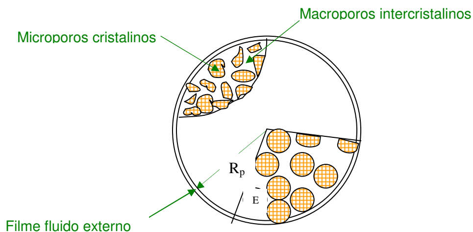
Figura 3 – Diagrama esquemático de pellet adsorvente (representação ideal, cristaltos esféricos uniformes), mostrando os três tipos principais de resistência à transferência de massa. (RUTHVEN, 1984)
