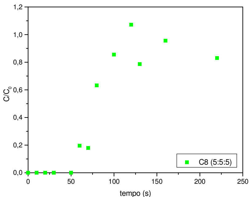
Figura 65 - Curva de ruptura para o iso-octano a partir da dispersão Água/hidrocarbonetos com concentração total 15%, sendo 5% de hexano, 5% de heptano e 5% de iso-octano. Q = 2,9 mL/s e H=23,6 cm.
