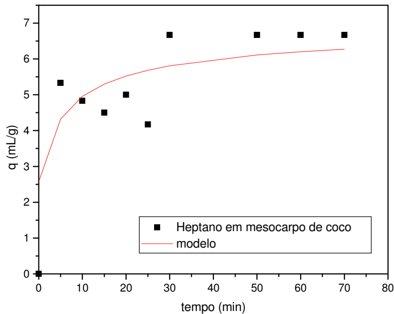
Figura 31 – Cinética de adsorção de heptano em mesocarpo de coco, R_{HCB} = 10
