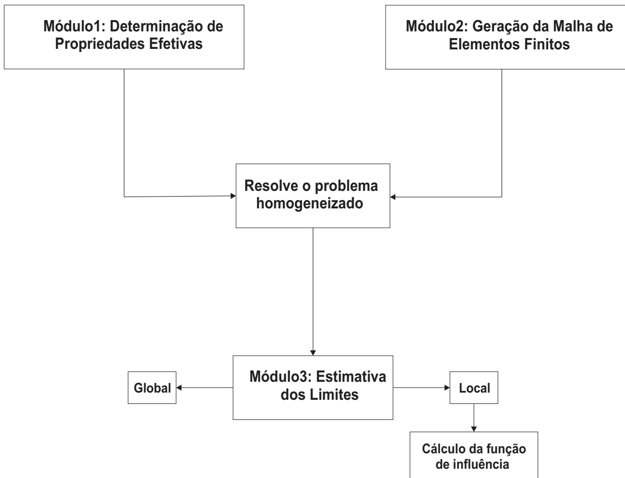
Figura 4.2: Representação da interação entre os módulos do MODERE.
