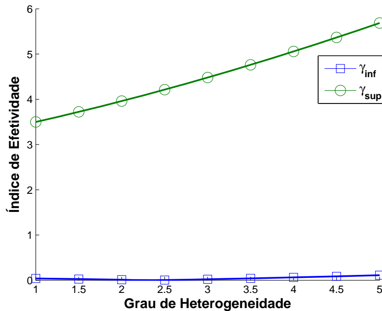
Figura 5.9: Estimativas do erro de modelagem global em função do grau de heterogeneidade para o caso de pressão externa.
