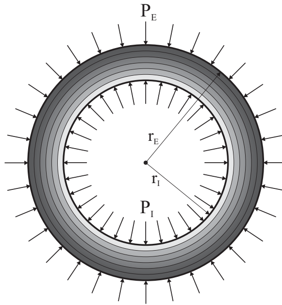
Figura 5.5: Tubo laminado.
