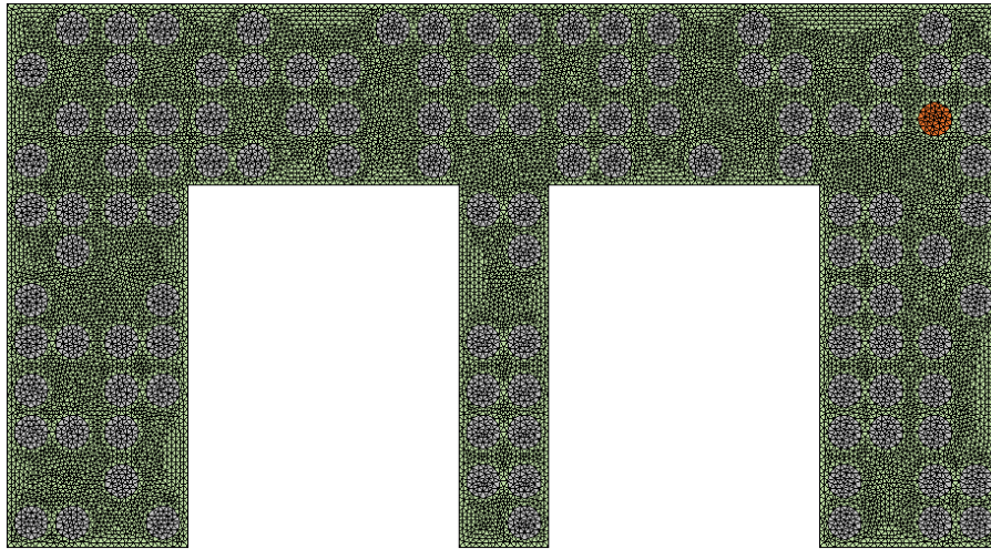
Figura 5.17: Malha de elementos finitos T6 utilizada nas análises.
