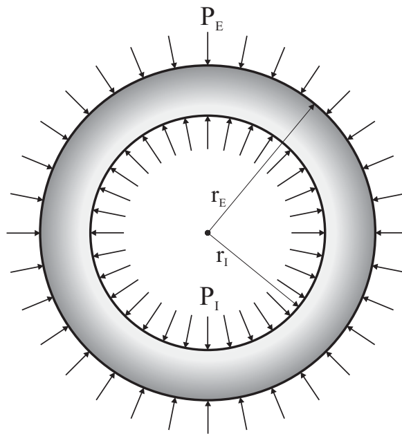
Figura 5.4: Tubo de FGM.
