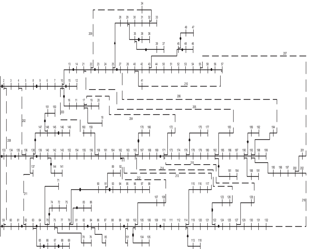
Figura 30: Sistema de 202 barras.
