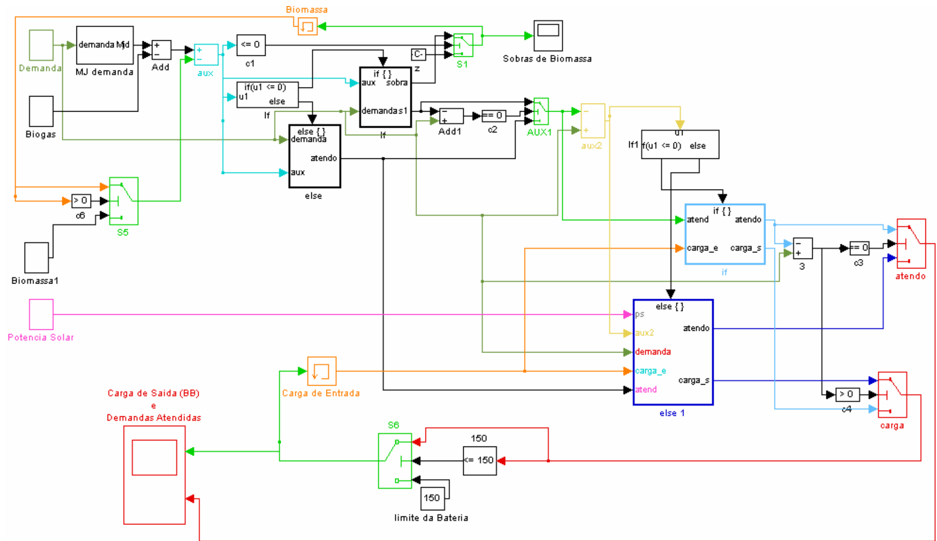
Figura 5.11: Sistema Especialista de Supervisão e Gerenciamento.
