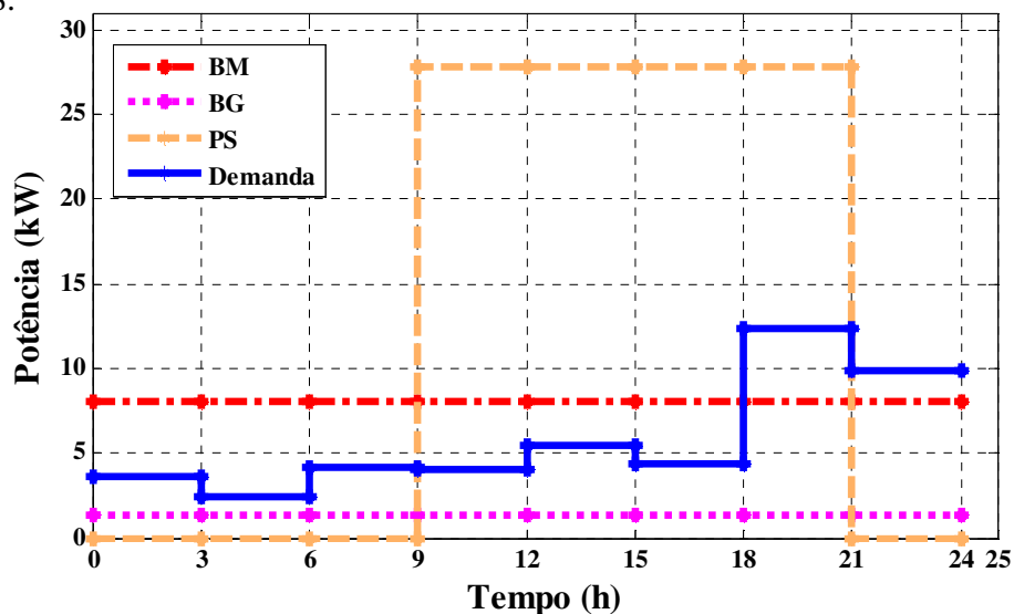
Figura 5.8: Cenário 5 – Dia Típico de Inverno com 27 visitantes.
