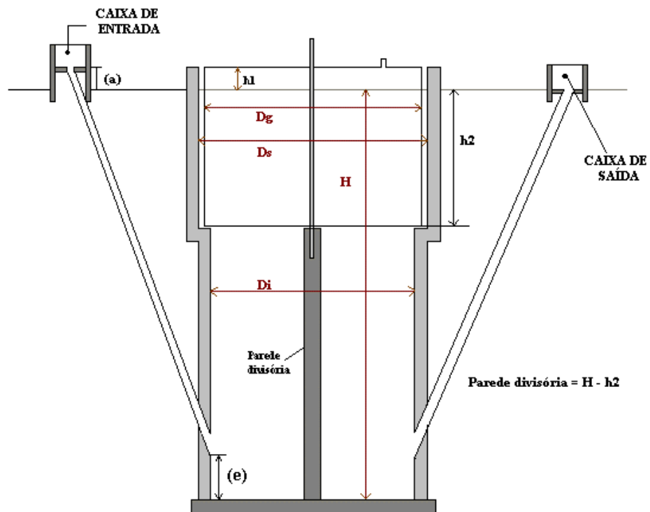
Figura 2.3: Biodigestor Modelo Indiano.
