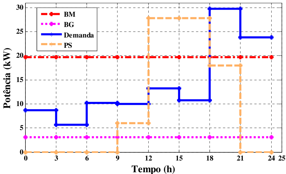
Figura 5.4: Cenário 1 – Dia Típico de Inverno com 65 Visitantes.
