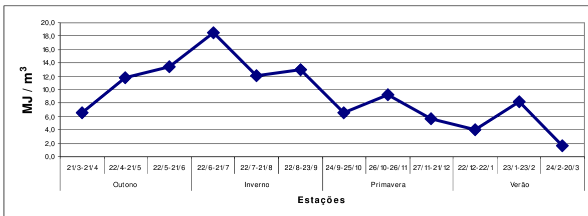
Figura 5.15: Produção Média de biogás por Estação.
