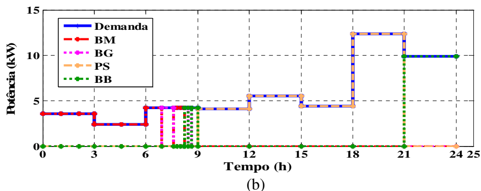
Figura 6.5: Resultado do Cenário 5.
