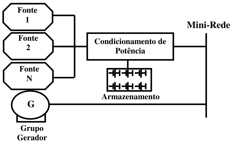
Figura 3.2: Configuração básica do sistema híbrido isolado.
