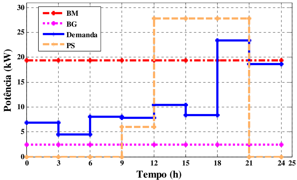
Figura 5.7: Cenário 4 – Dia Típico de Outono com 51 visitantes.
