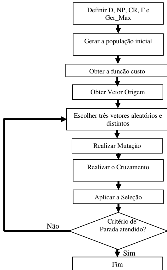
Figura 4.1: Fluxograma da Evolução Diferencial.
