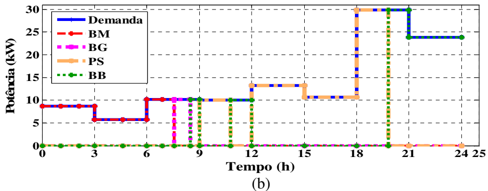
Figura 6.1: Resultado do Cenário 1.
