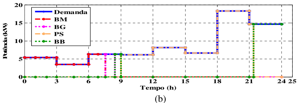
Figura 6.2 Resultado do Cenário 2.
