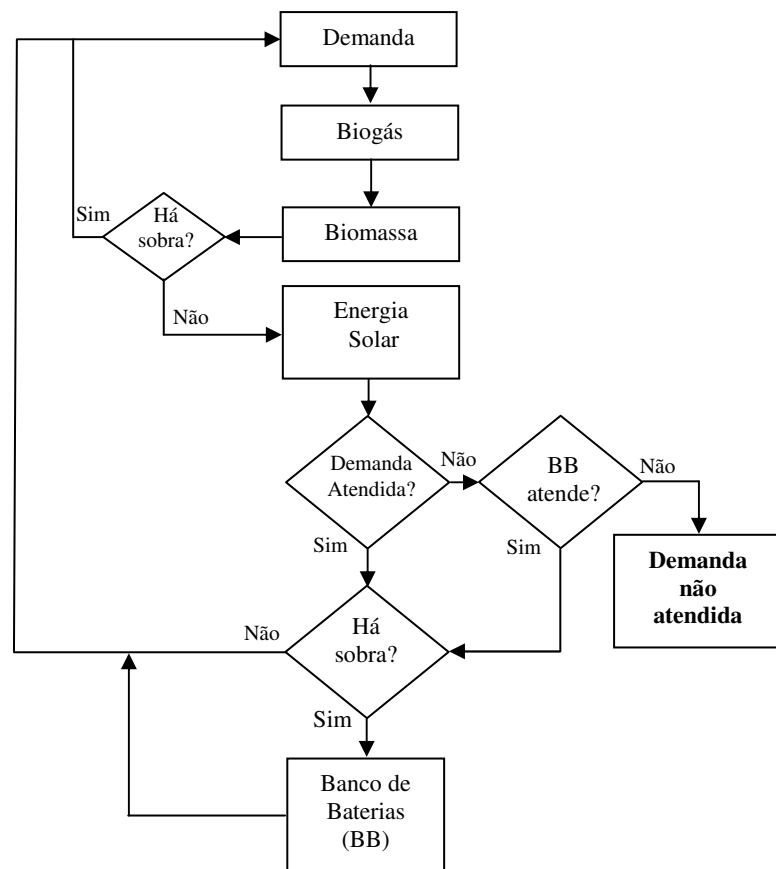
Figura 5.10: Fluxograma do sistema especialista de supervisão e gerenciamento.
