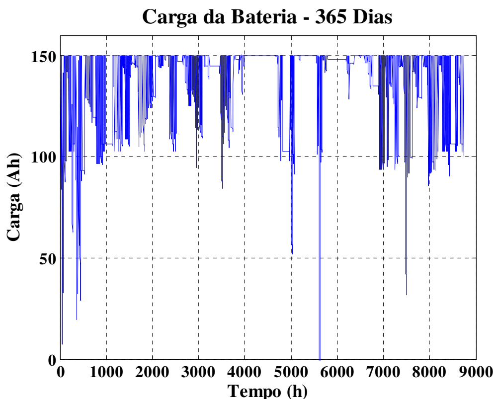
Figura 6.6: Resultado do Cenário Anual. Carga do Banco de Baterias.
