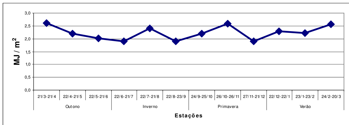
Figura 5.16: Média da Irradiação solar por Estação.
