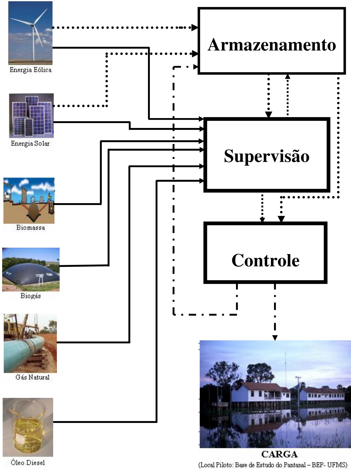
Figura 5.1: Detalhamento da idéia principal do projeto.
