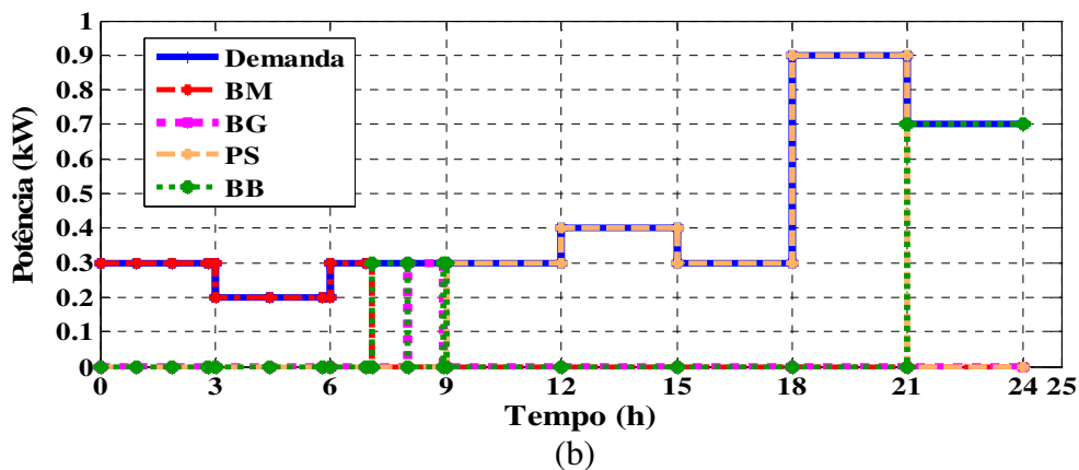
Figura 6.3: Resultado do Cenário 31.
