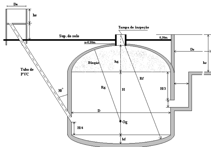
Figura 2.4: Biodigestor Modelo Chinês. Fonte: DEGANUTTI et al. [18].
