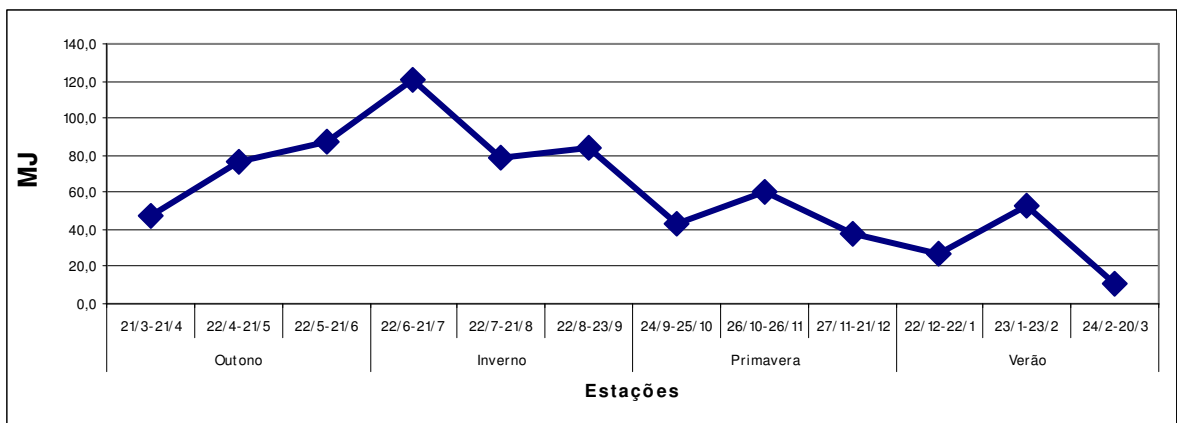
Figura 5.13: Produção Média de biomassa por Estação.
