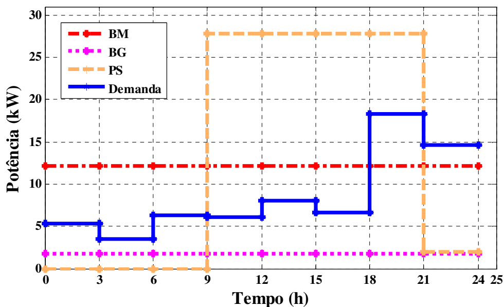
Figura 5.5: Cenário 2 – Dia Típico de Primavera com 40 Visitantes.
