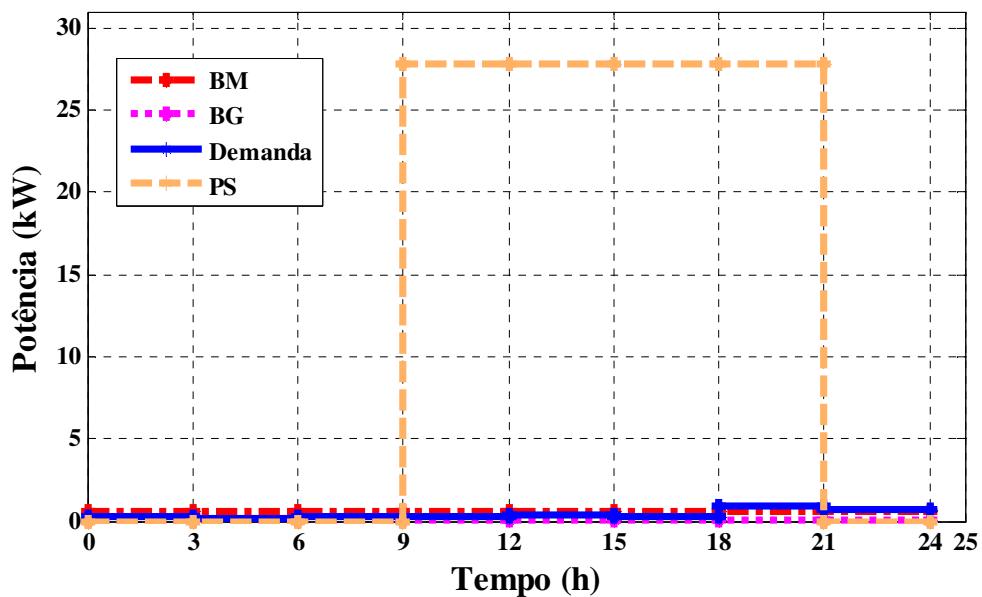
Figura 5.6: Cenário 3 – Dia Típico de Verão com 2 visitantes.
