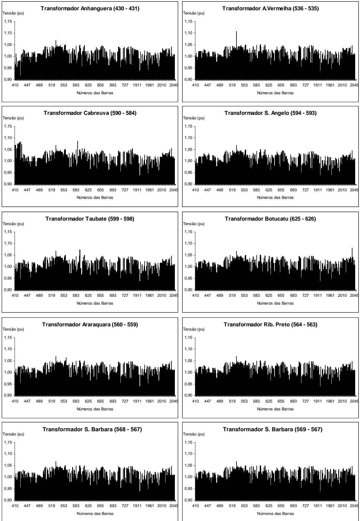
Figura 4.23.1 - Perfis de tensão com problemas após as alterações dos taps de transformadores para a eliminação da sobrecarga no transformador de S. Bárbara 440/138 kV no caso de julho de 2005.
