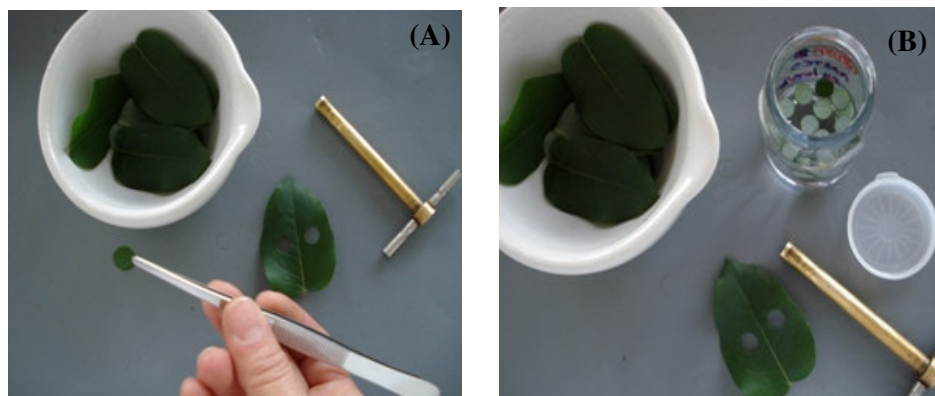
Figura 1 – Corte dos discos foliares de Eucalyptus dunnii com perfurador de rolha (A), para posterior determinação de condutividade elétrica (B).
