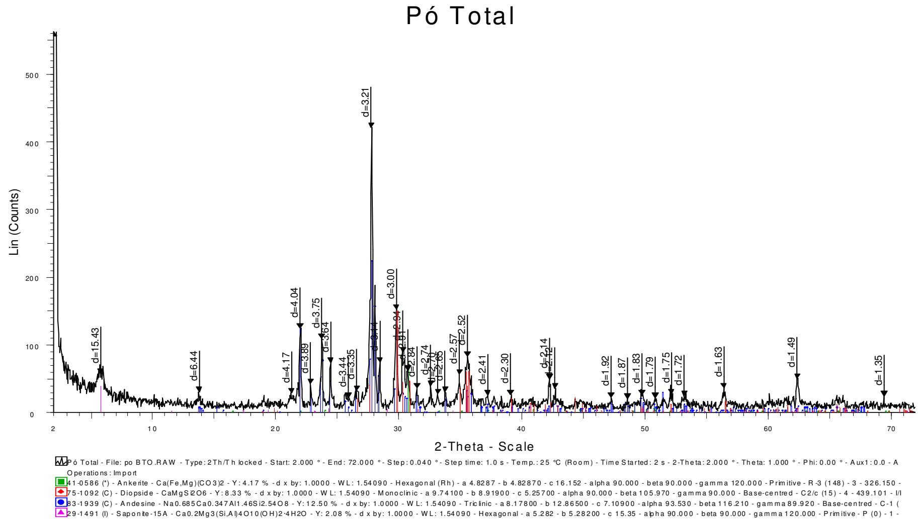
Figura 16: Difratograma de pó total da rocha basáltica.
