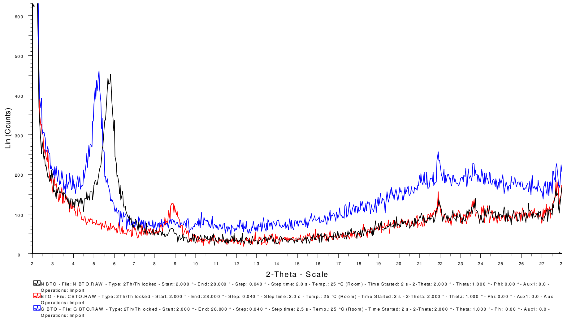
Figura 14: Difratoograma de rocha basáltica (natural, calcinada e glicolada) – Todos sobrepostos..
