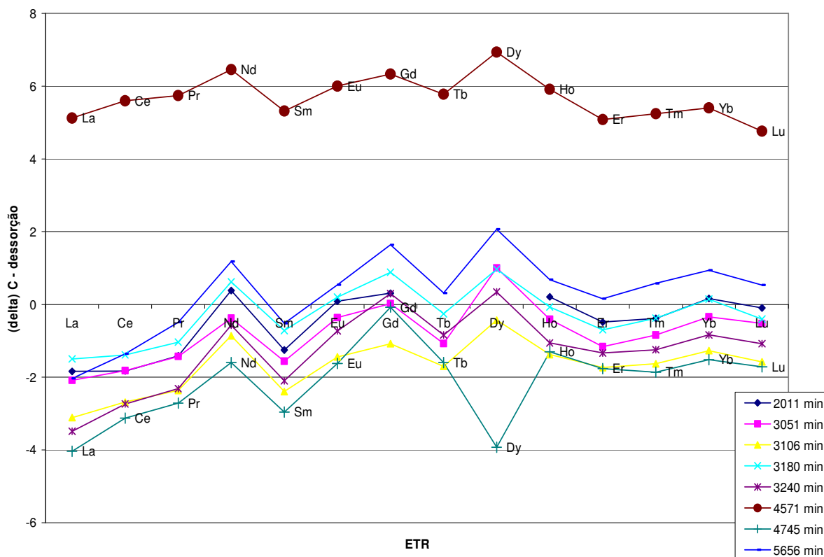
Gráfico 14: (Dessorção) Concentração em função do tempo. ( I=0,500M NaCl )
