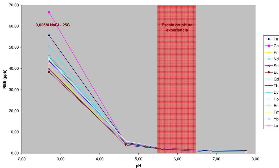
Gráfico3: Batch Test . Concentração (ppb) versus pH, em baixa força iônica ( I = 0,025 \text{ M} )
