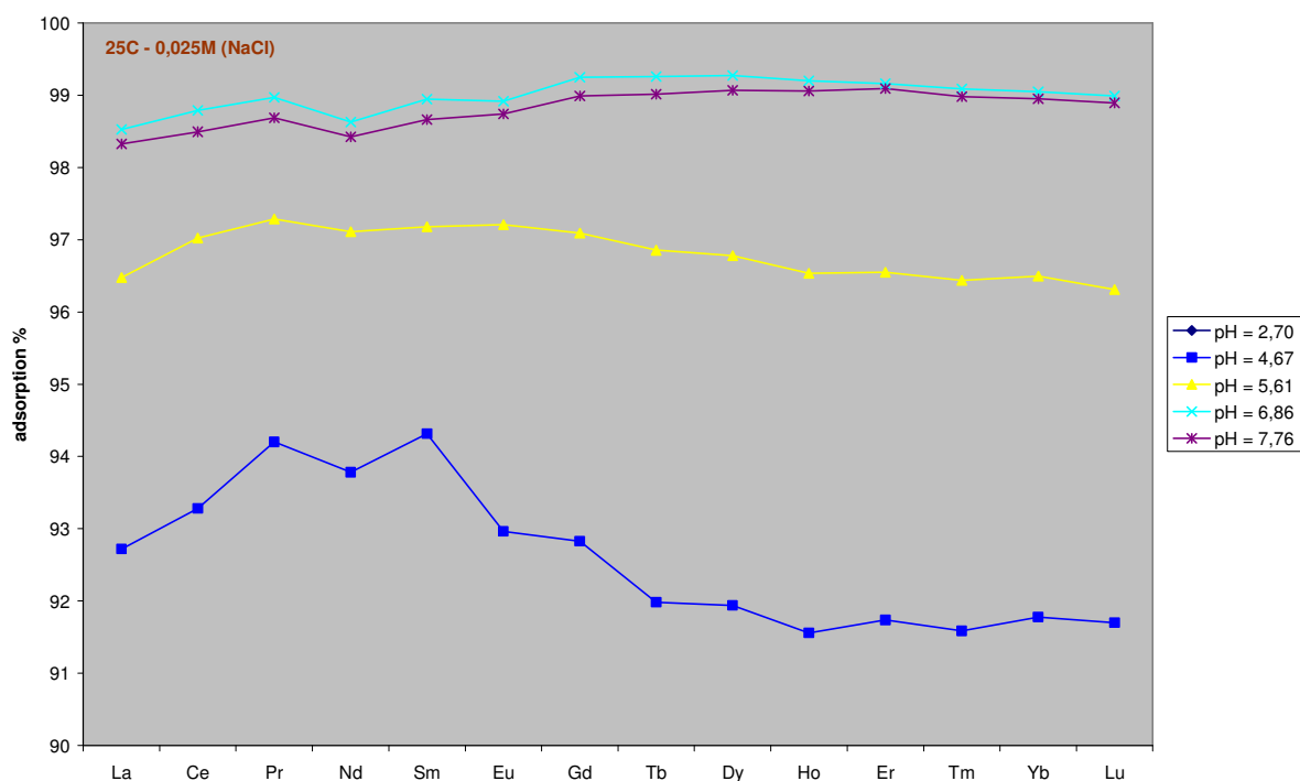
Gráfico 8: percentual de adsorção dos ETR(Z) em função do pH. (I=0,025M)
