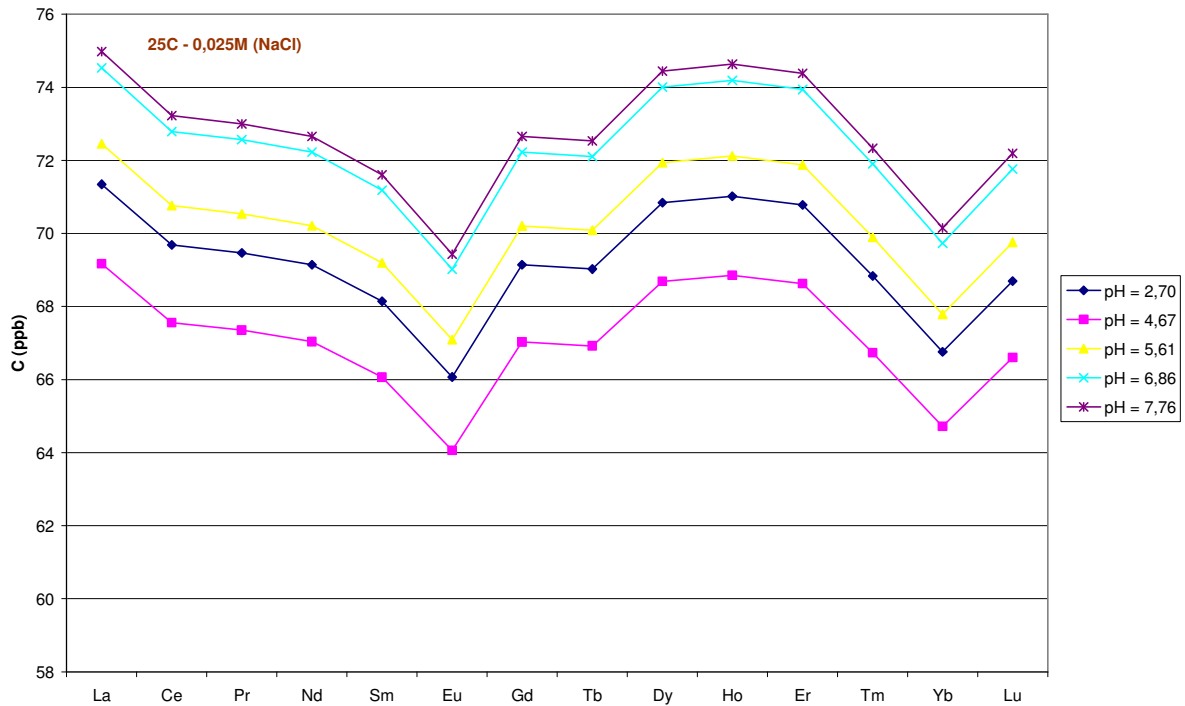
Gráfico 1: Concentração dos ETR, em solução inicial, sem interação com o basalto. I=0,025M
