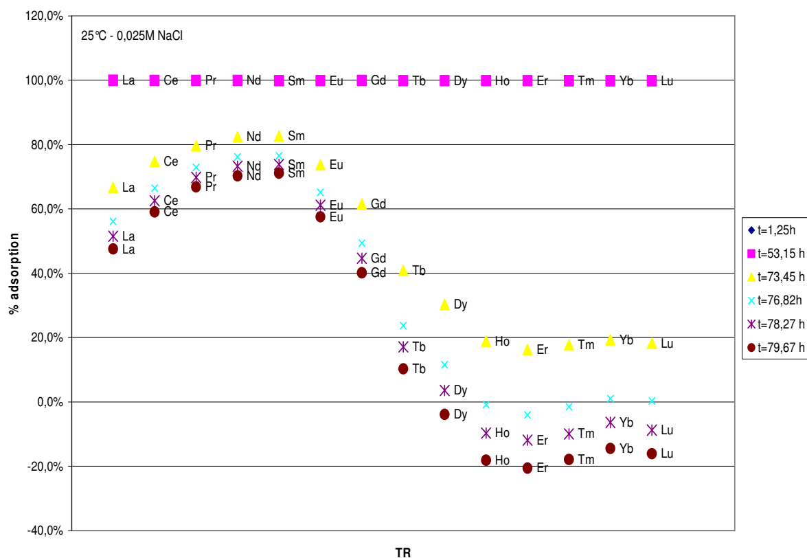
Gráfico 11: Percentual de adsorção dos ETR, em função do tempo. Escala de tempo maior. Força iônica I=0,025M (NaCl)
