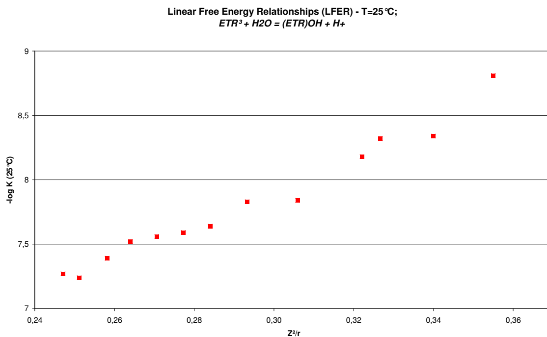
Gráfico 17: Linearização da energia livre para ETR^{3+} + H_2O .
