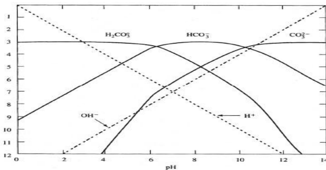
Figura 11: Controle dos carbonatos em solução
