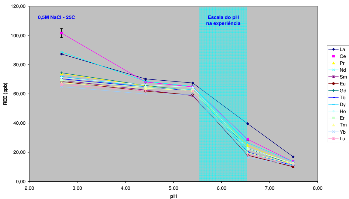
Gráfico4: Batch Test . Concentração (ppb) versus pH, em alta força iônica ( I = 0,500 \text{ M} )
