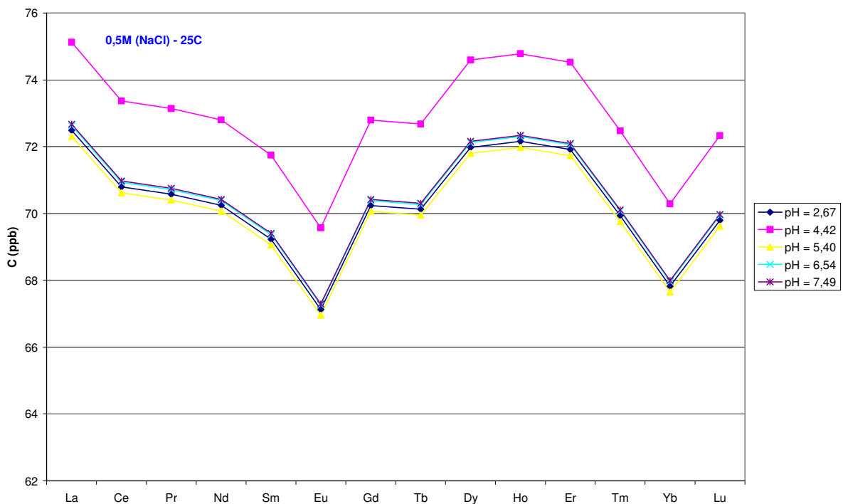
Gráfico 2: Concentração dos ETR, em solução inicial, sem interação com o basalto. I=0,500M
