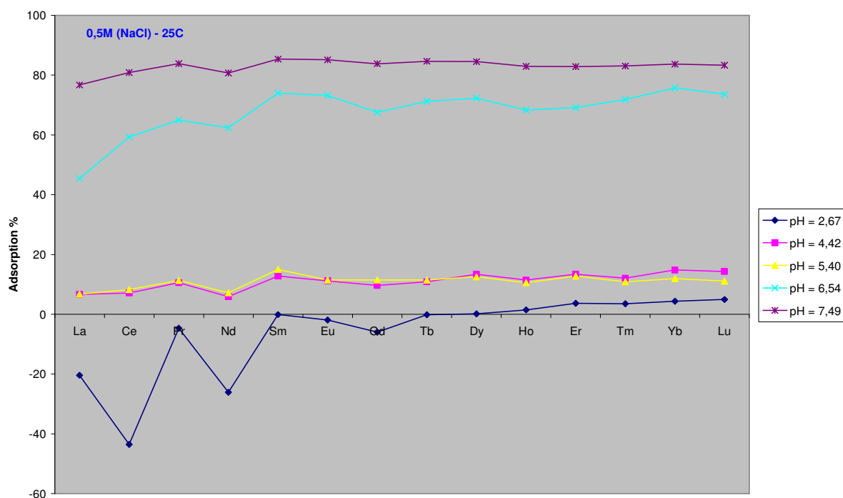
Gráfico 9: percentual de adsorção dos ETR(Z) em função do pH. (I=0,500M)
