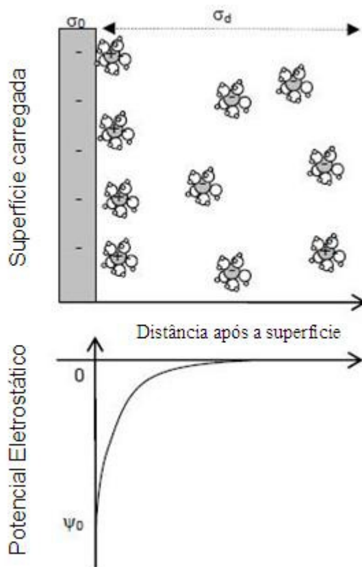
Figura 7: Representação gráfica do modelo da camada dupla difusa e a relação do potencial eletrostático ( \Psi ) em função da distância a superfície.
