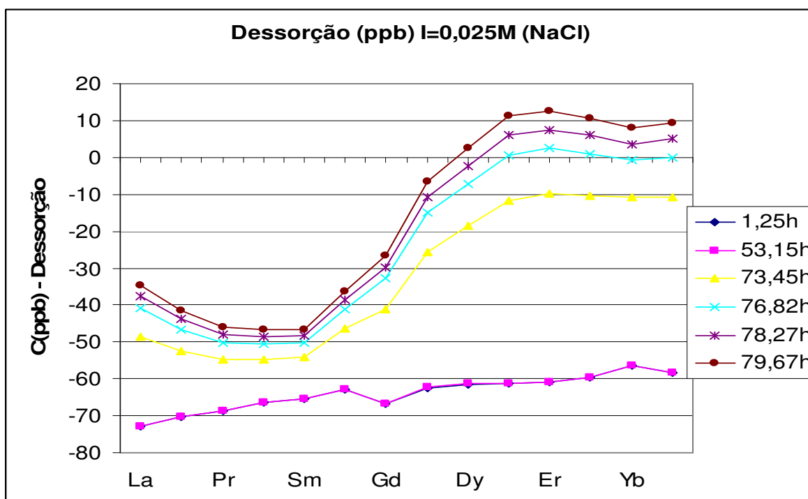
Gráfico 15: (Dessorção) Concentração em função do tempo. ( I=0,025M )
