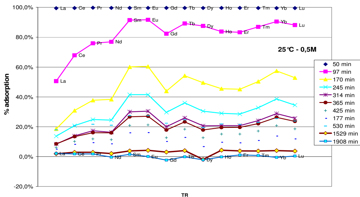
Gráfico 12: Percentual de adsorção dos ETR, em função do tempo. Escala de tempo maior.
