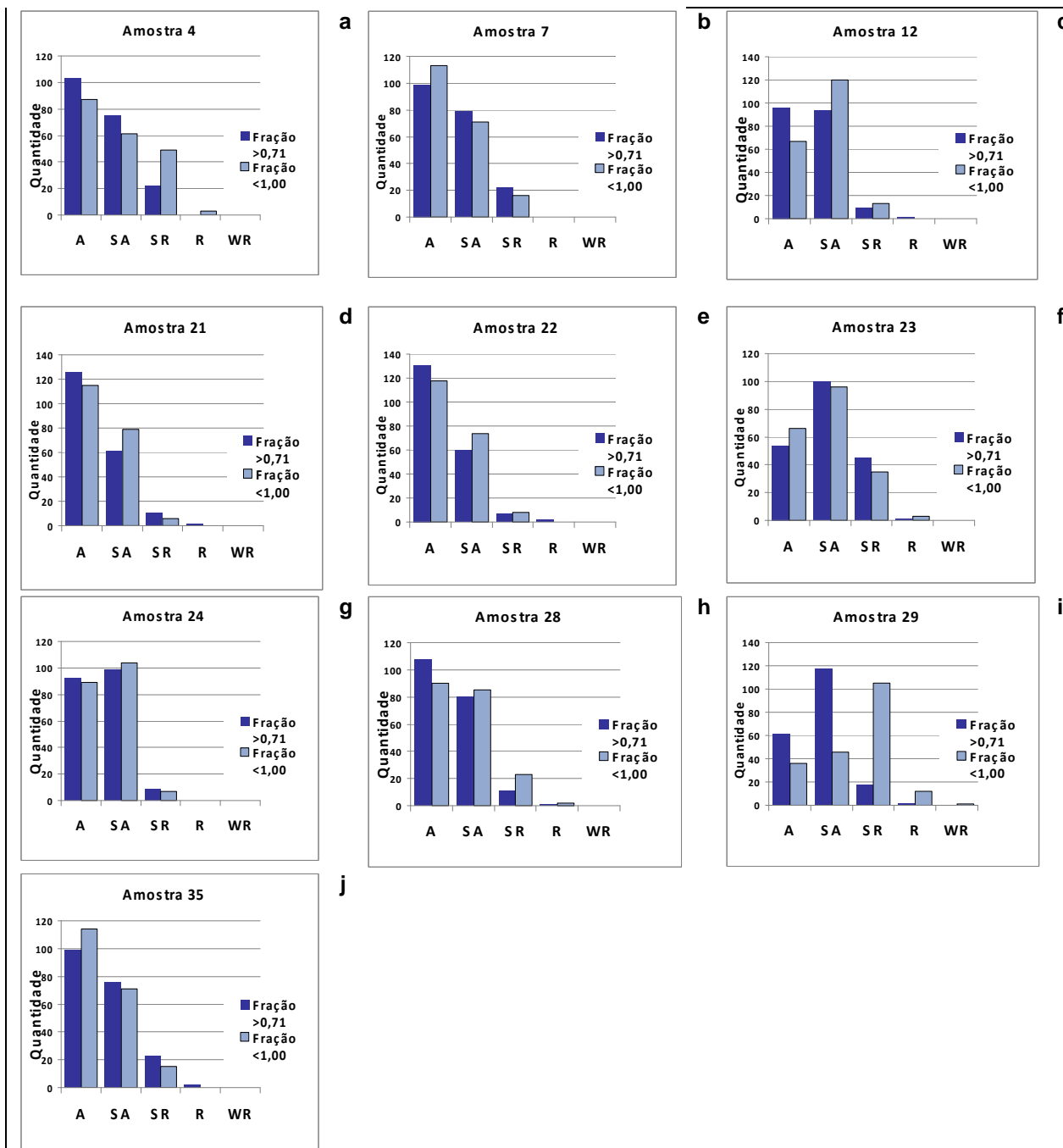
Figura 25 – Graus de arredondamento de cada depósito conforme análise de amostras de 100 g.
