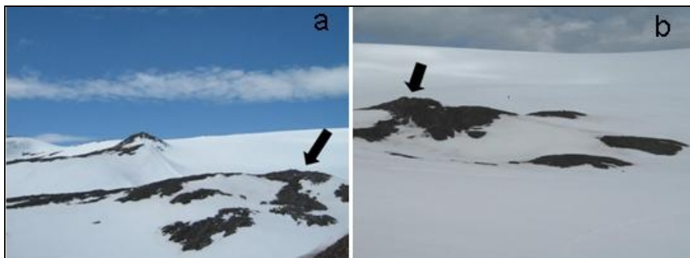
Figura 51 – Fotografia a mostra o bloco rochoso subglacial (amostra 5) localizado no setor elevado da moraina oriental a 101 metros de altitude. Fotografia b mostra o depósito subglacial (amostra 8) sob a moraina lateral (Fotografias de Rosa, 2007).
