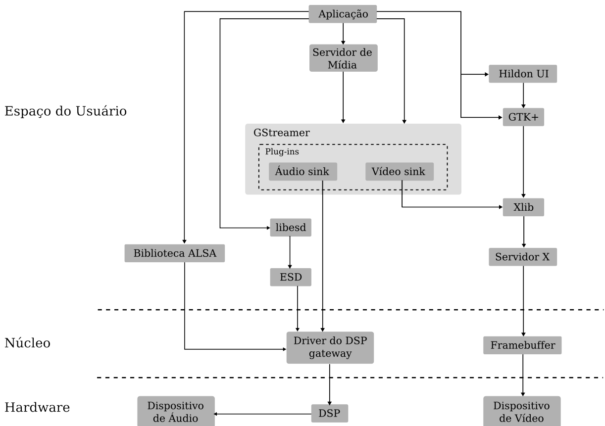
Figura 7.1: Principais elementos do módulo de multimídia da plataforma maemo.
