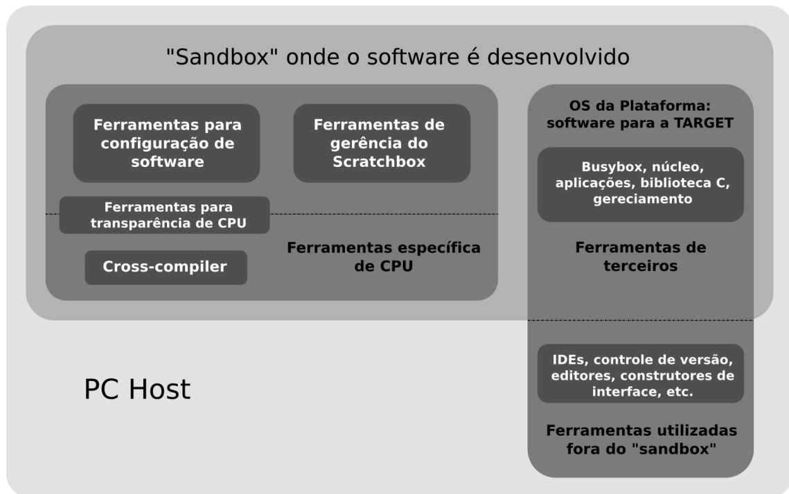
Figura 11.1: Funcionamento do Ambiente Scratchbox.
