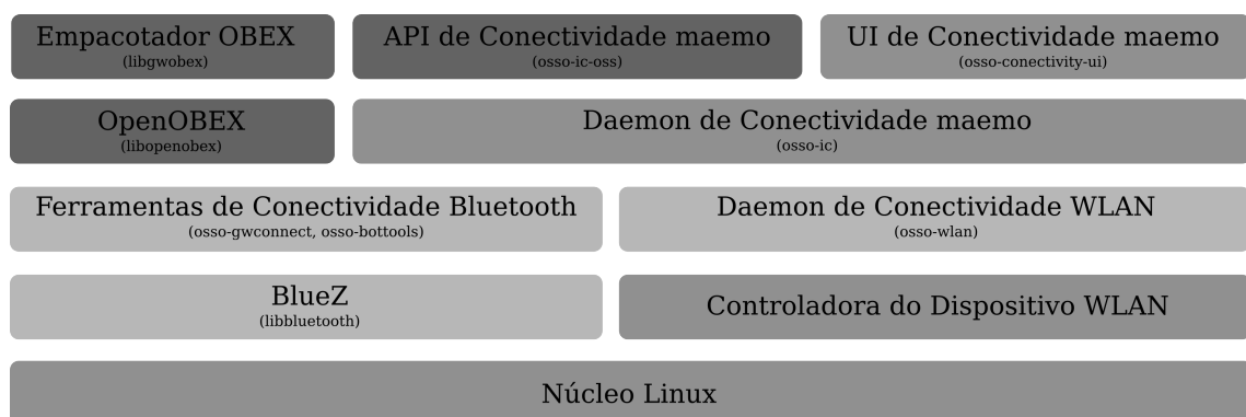
Figura 8.1: Elementos do subsistema de conectividade da plataforma maemo.
