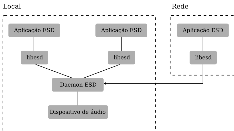
Figura 7.2: Comunicação entre aplicativos ESD.
