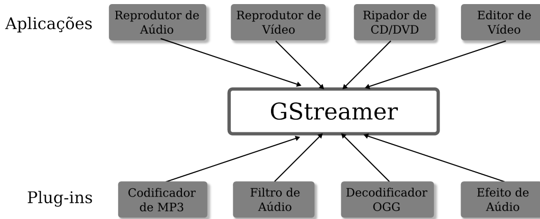
Figura 7.4: Arquitetura do framework GStreamer.
