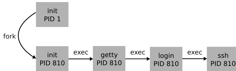
Figura 2.4: Mecanismo de criação de processos.
