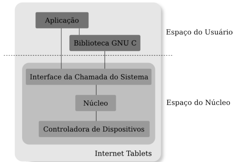
Figura 2.2: Espaços de memória.
