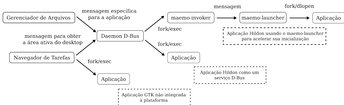
Figura 3.4: Métodos para ativação de aplicações.
