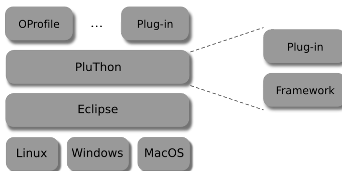
Figura 12.4: Arquitetura de ferramenta PluThon.
