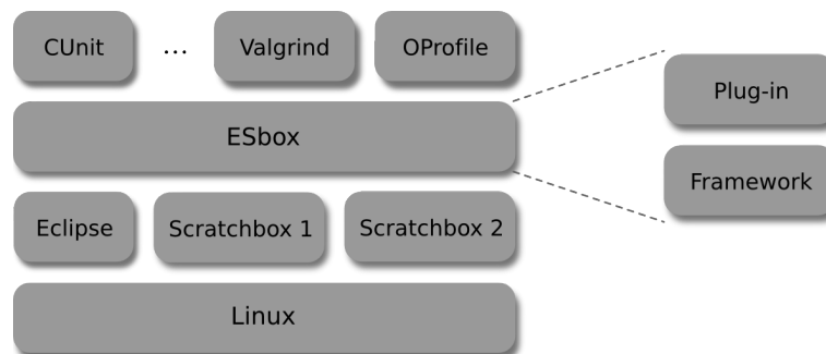
Figura 12.2: Arquitetura da ferramenta ESbox.
