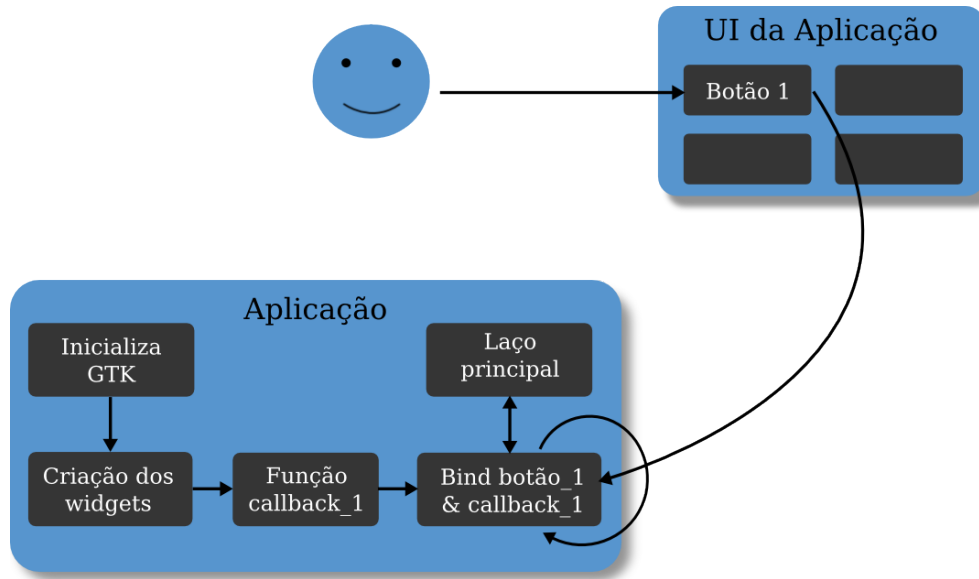
Figura 6.7: Notificação de um evento gerado pela interação do usuário com a interface gráfica.
