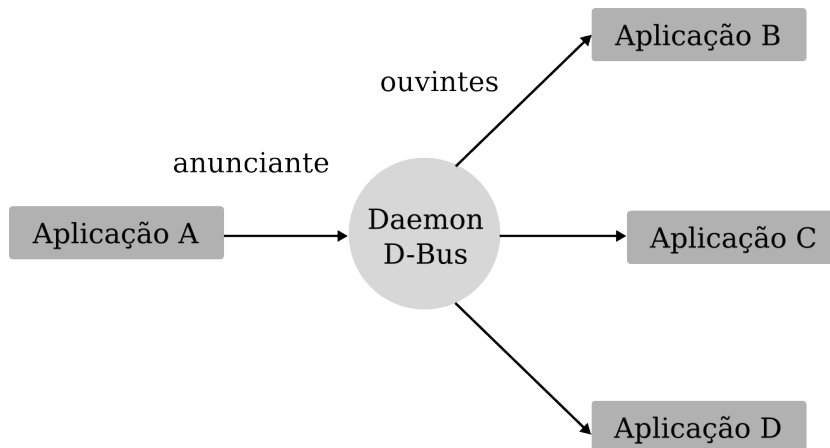
Figura 5.2: Envio de sinais por uma aplicação via D-Bus.
