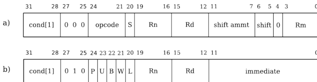
Figura 13.4: Exemplo de formatos de instrução do ARM.
