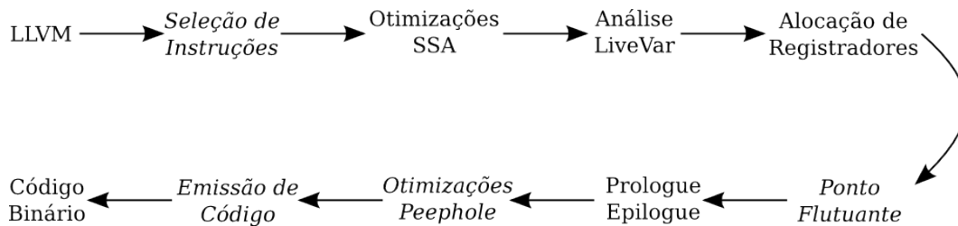
Figura 13.3: Fases de geração de código.
