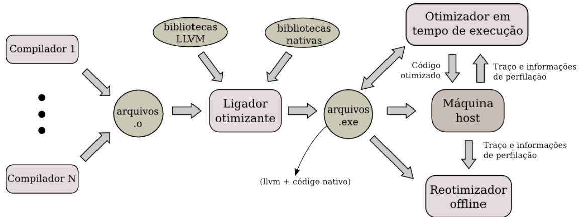
Figura 13.2: Estratégia de compilação do LLVM.
