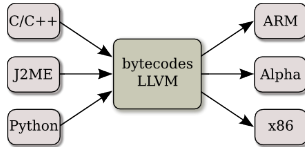
Figura 13.1: Cenário de utilização.
