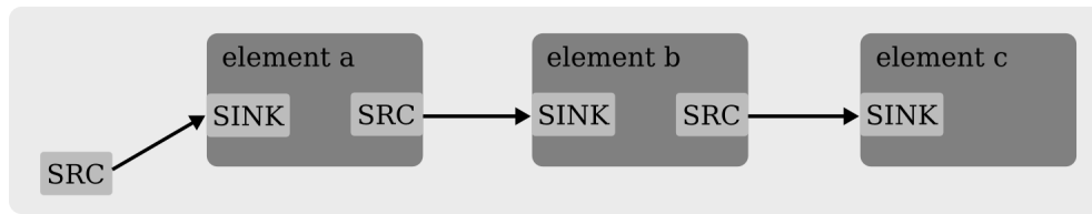
Figura 7.6: Elements contidos em um bin.
