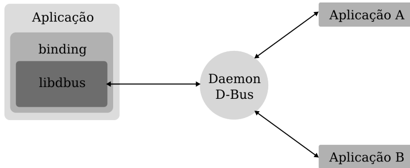
Figura 5.1: Comunicação ponto-a-ponto entre aplicações via D-Bus.
