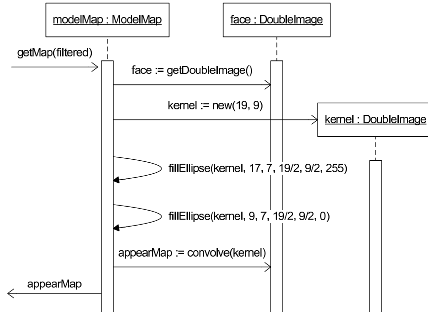
Figura 4.9: Diagrama de seqüência da geração de mapa de evidência baseado em modelos.
