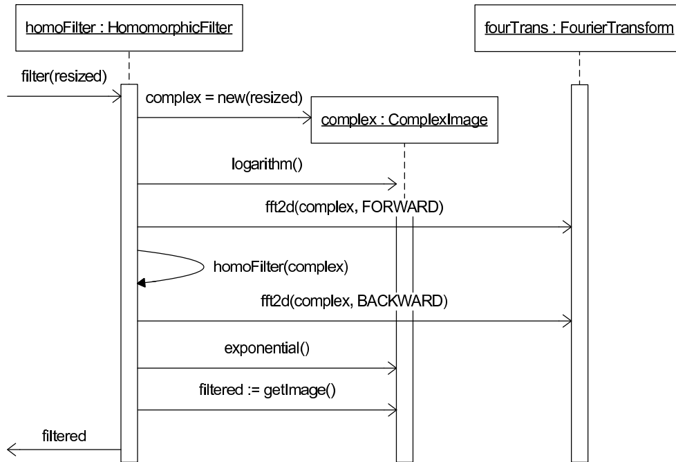
Figura 4.5: Diagrama de sequência da filtragem homomórfica.
