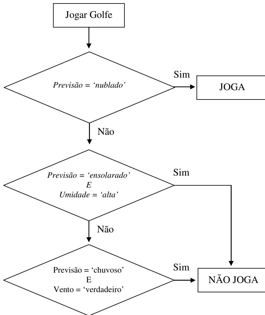
Figura 2.1: Árvore de decisão que descreve o problema "Jogar Golfe"
