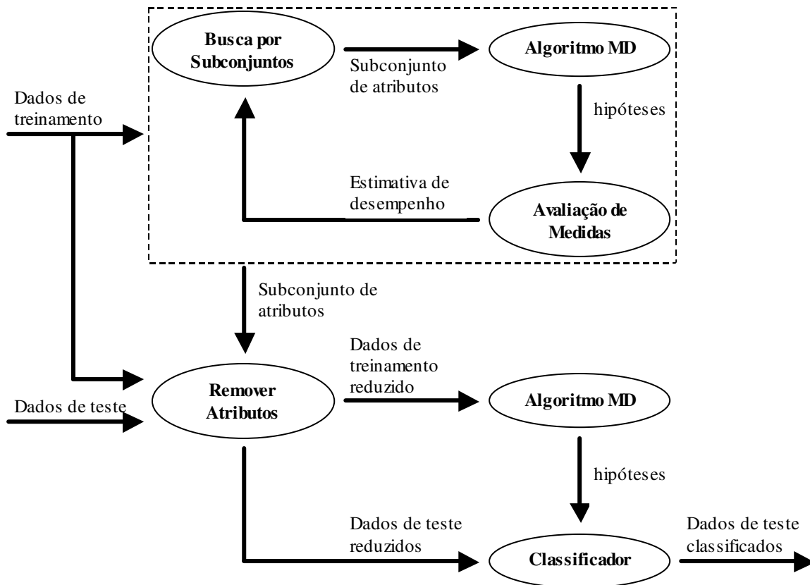
Figura 3.4: Esquema de abordagem para SA: Abordagem Wrapper
