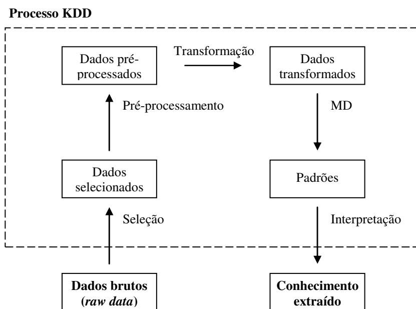
Figura 1.2: Diagramação do Processo KDD
