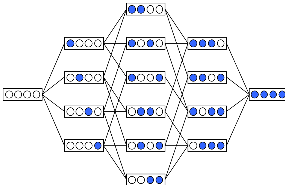
Figura 3.1: Exemplo de espaço de busca de subconjunto atributos [Langley, 1994]
