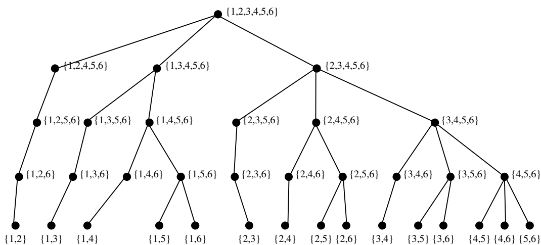
Figura 5.6: Árvore de busca da ferramenta Branch and Bound
