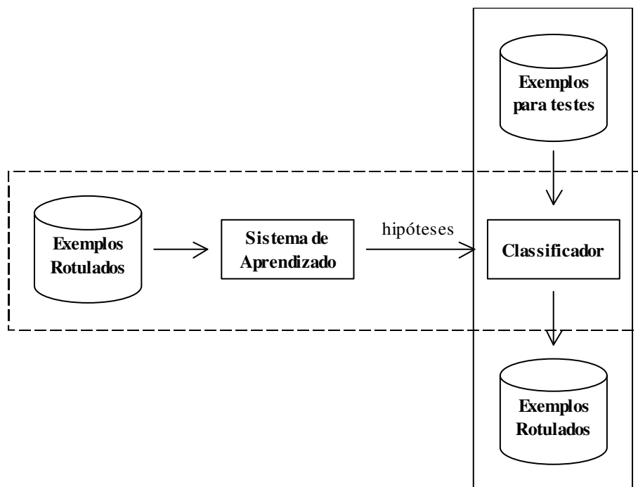
Figura 1.1: Sistema de AM para Classificação [Pila, 2001]
