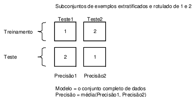
Figura 4.2: Esquema de validação cruzada
