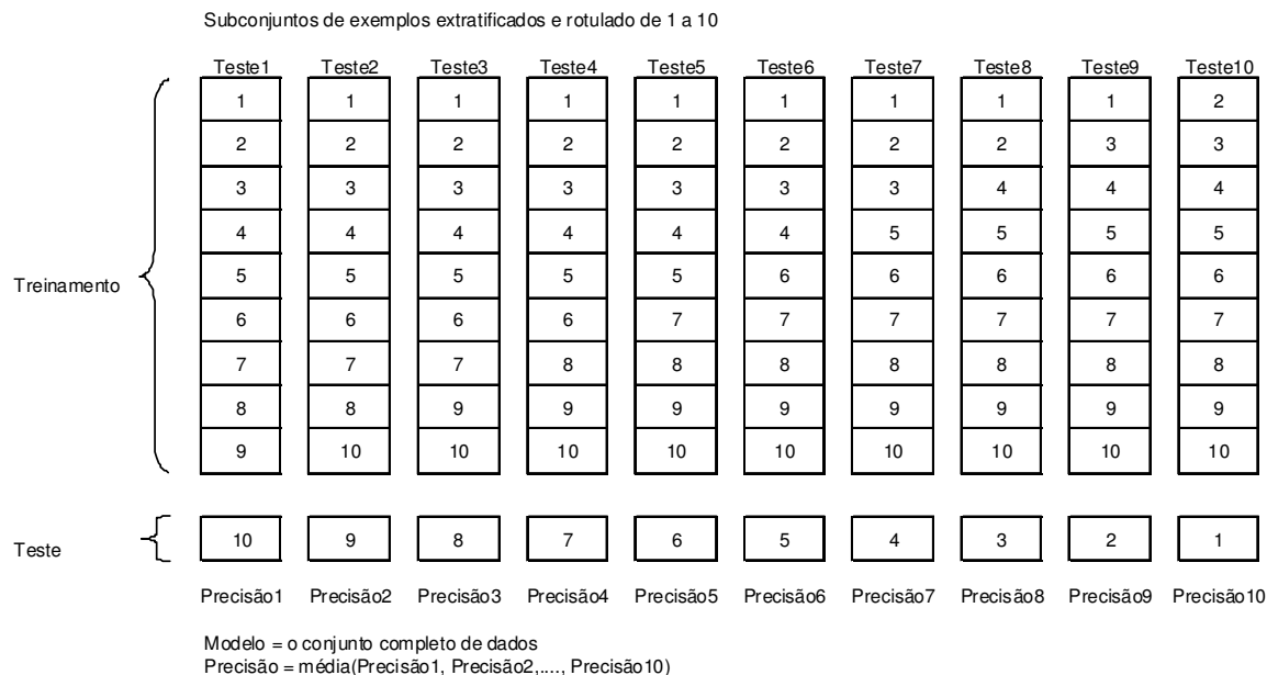
Figura 4.3: Esquema de validação cruzada com 10-partições estratificadas
