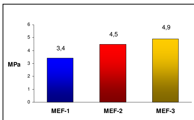
Fig. 13: Gráfico de valores (MPa) dos pontos de tensão lateral
