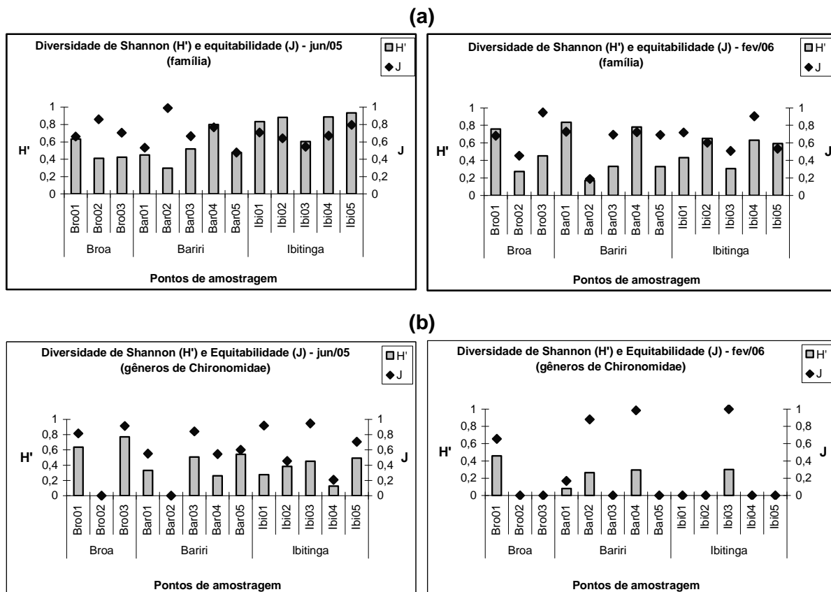
Figura 42 – Índice de Diversidade de Shannon (H') e Equitabilidade (J) tirados para as famílias de macroinvertebrados (a) e para os gêneros de Chironomidae (b) no período de junho de 2005 (seca) e fevereiro de 2006 (chuva).
