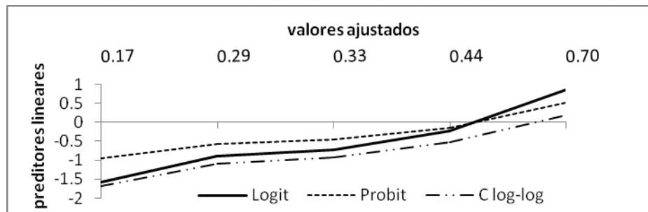
FIGURA 7: Valores ajustados das proporções do modelo binomial usando funções de ligação logit, probit e complemento log-log utilizado para modelar a proporção de ovos parasitados, a cada passo efetuado do método de inspeção com a estratégia não-proporcional.
