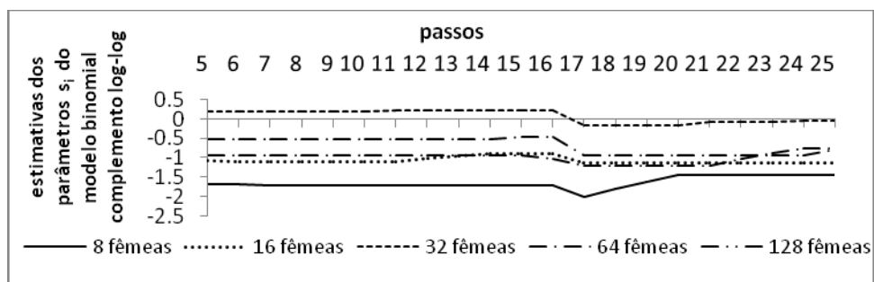
FIGURA 4 Inspeção das estimativas dos parâmetros s_i do modelo binomial sem o intercepto c , com funções de ligação logit (a), probit (b) e complemento log-log (c), utilizado para modelar a proporção de ovos parasitados a cada passo efetuado do método de inspeção com a estratégia não-proporcional.
