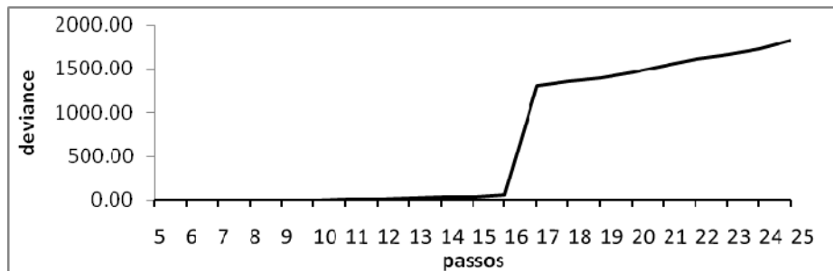
FIGURA 6 Inspeção dos valores da deviance do modelo binomial considerando as funções de ligação logit, probit complemento log-log para modelar a proporção de ovos parasitados a cada passo efetuado do método de inspeção com a estratégia não-proporcional.
