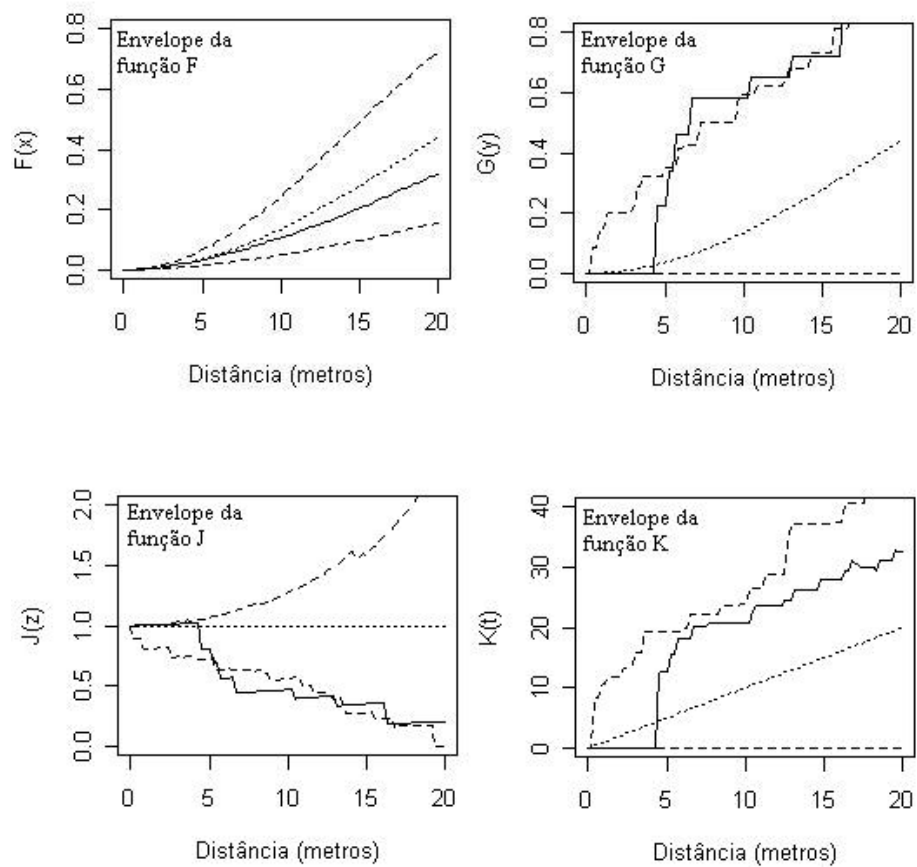
FIGURA 15: Envelope de simulação das funções: F , G , J , K ; limite superior (linha tracejada); limite inferior (linha tracejada); função teórica (linha pontilhada); função estimada (linha contínua).
