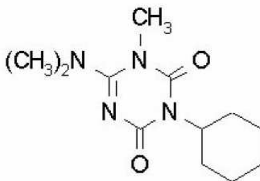
FIGURA 2 – Fórmula Estrutural do herbicida Hexazinona
