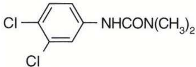
FIGURA 1 – Fórmula Estrutural do herbicida Diuron
