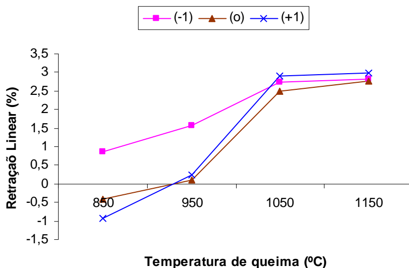
Figura 5.8. Variação da Retração Linear com a Temperatura de queima.
