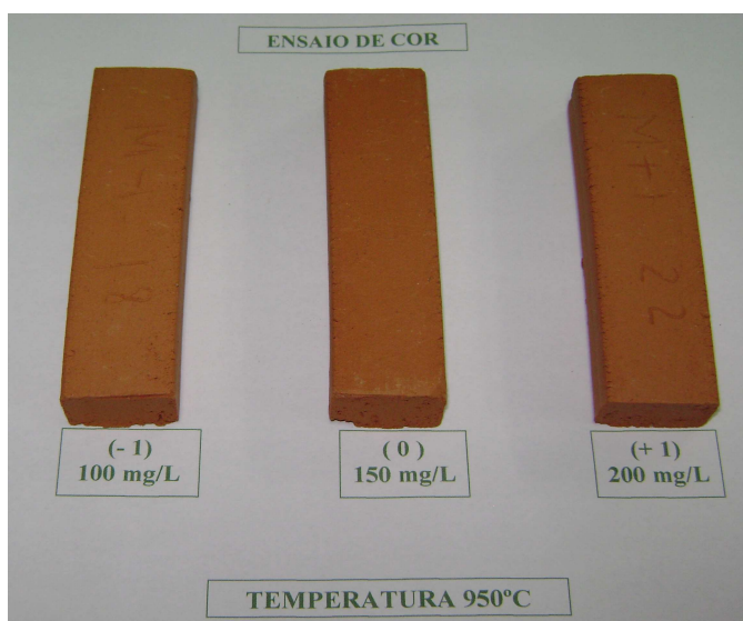
Figura 4.10. Corpos cerâmicos queimados a 950 °C.
