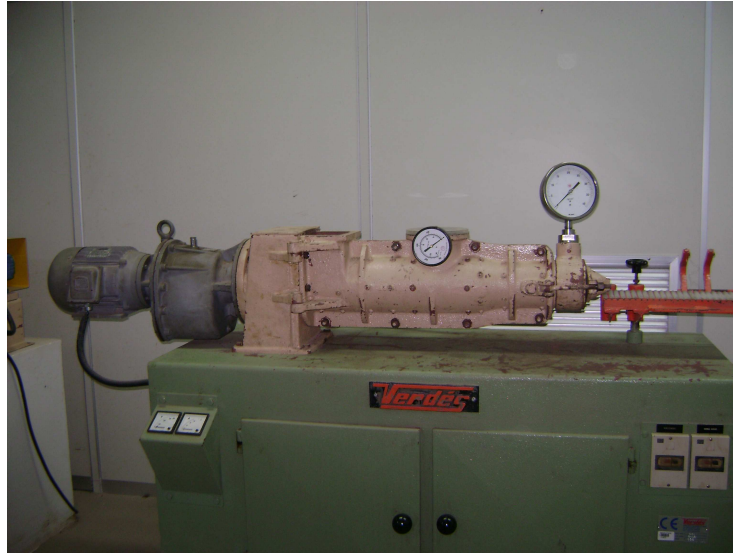
Figura 4.5. Extrusora Verdes modelo 051 e série 035.
