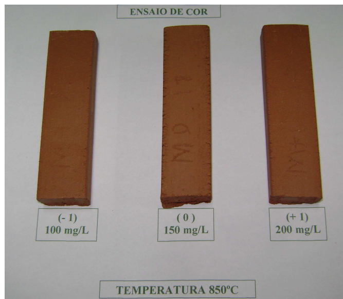
Figura 4.9. Corpos cerâmicos queimados a 850 °C.
