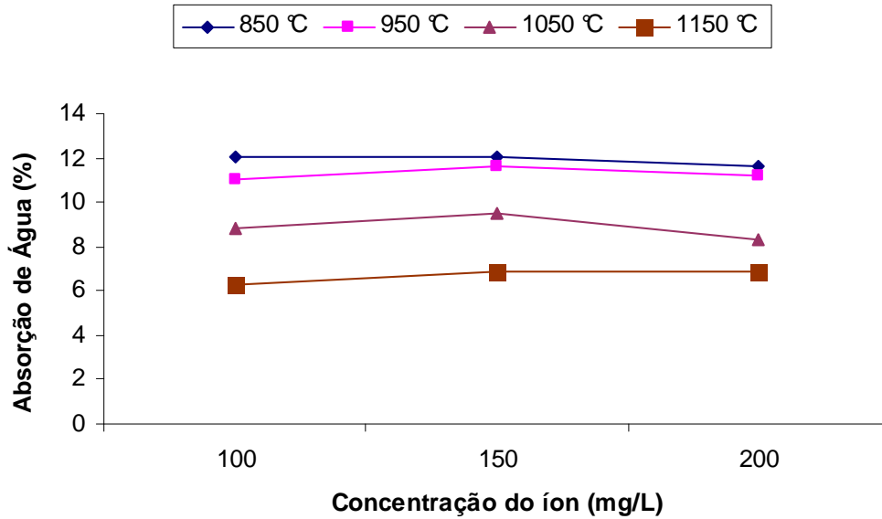
Figura 5.11. Variação da Absorção de Água com a Concentração do íon
