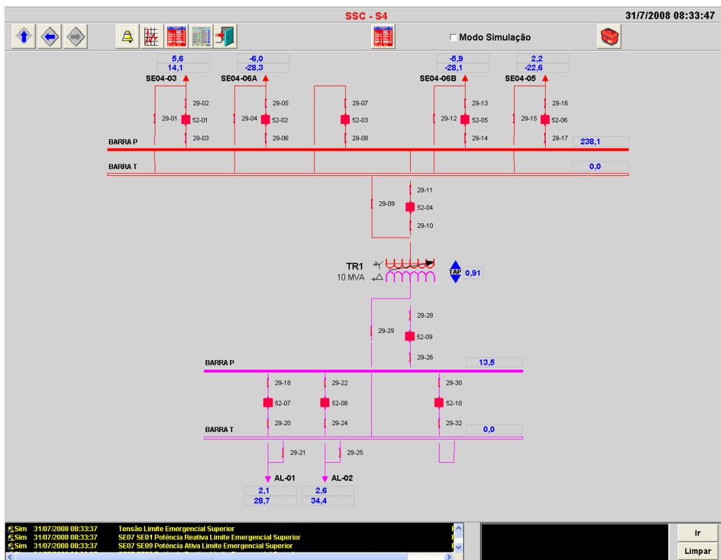
Figura 23: Diagrama de operação de uma subestação monitorada por uma UTR.
