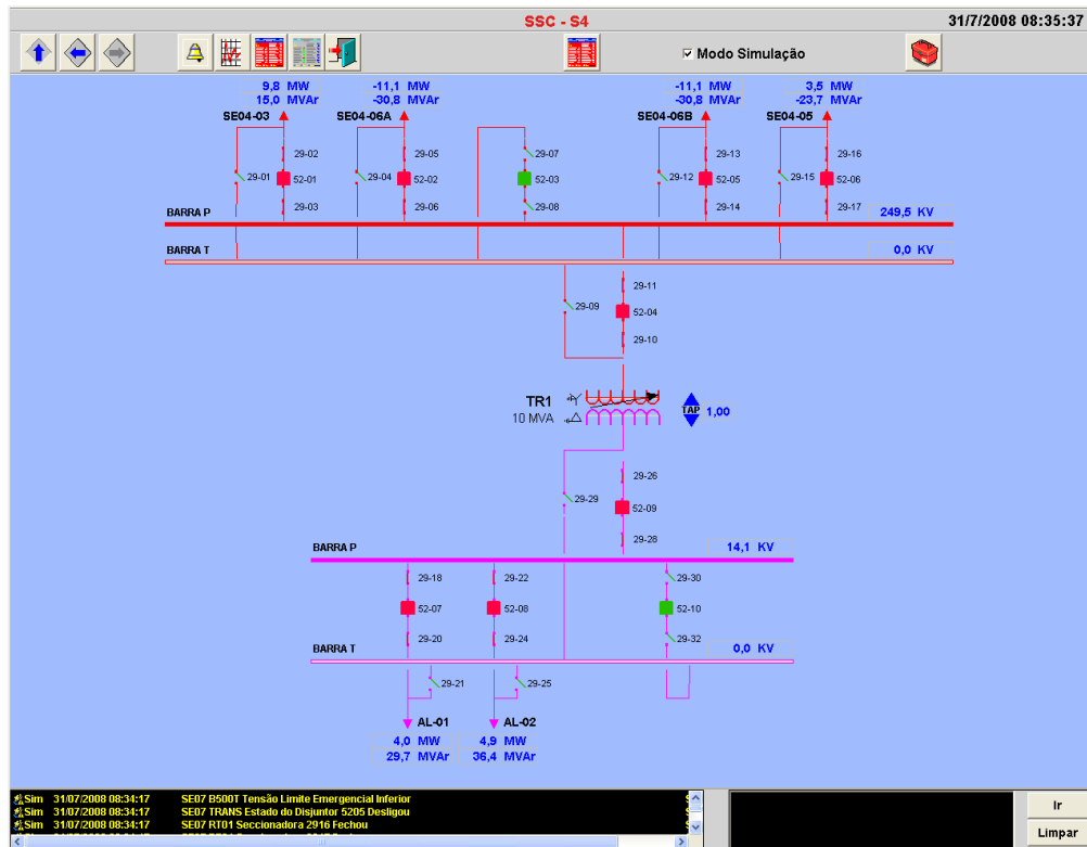
Figura 24: Diagrama de operação de uma subestação simulada pelo módulo PSM e acessada via CCM.
