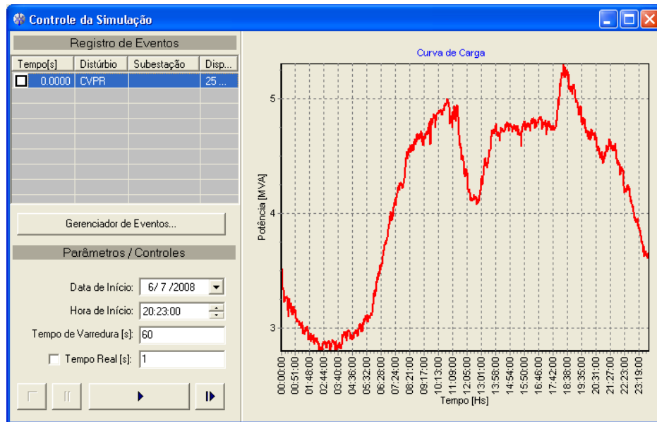
Figura 7: Curva de carga criada através do módulo ES do PSL ® -SDK.
