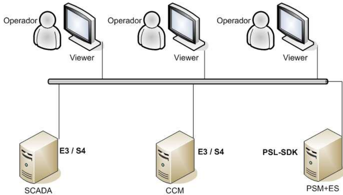
Figura 27: Plataforma configurada para trabalhar distribuída em três servidores.
