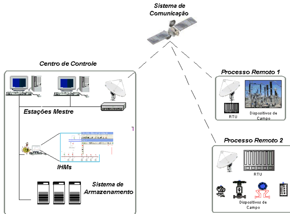
Figura 13: Diagrama esquemático de um sistema SCADA.
