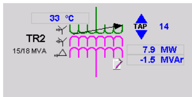
Figura 16: Representação Gráfica de um transformador no S4.
