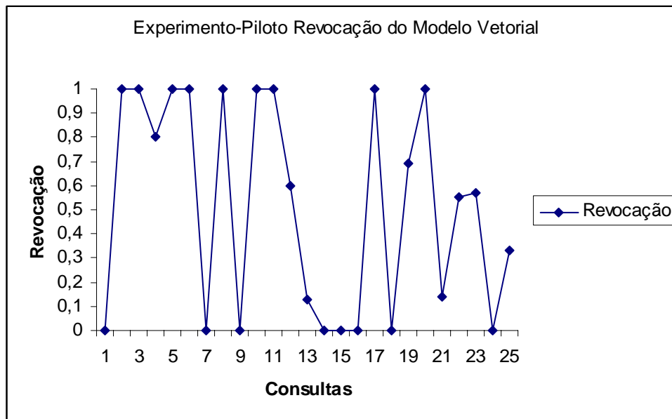
Figura 4.9.: Resultado de Revocação do Experimento-Piloto utilizando o Modelo Vetorial
