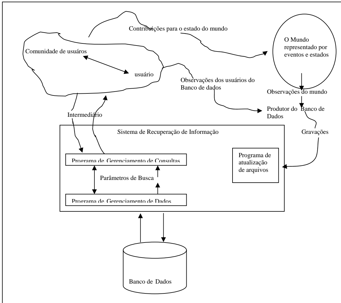
Figura 2.1. Visão Geral do cenário de um Sistema de Recuperação de Informação, adaptado de MEADOW 1992.
