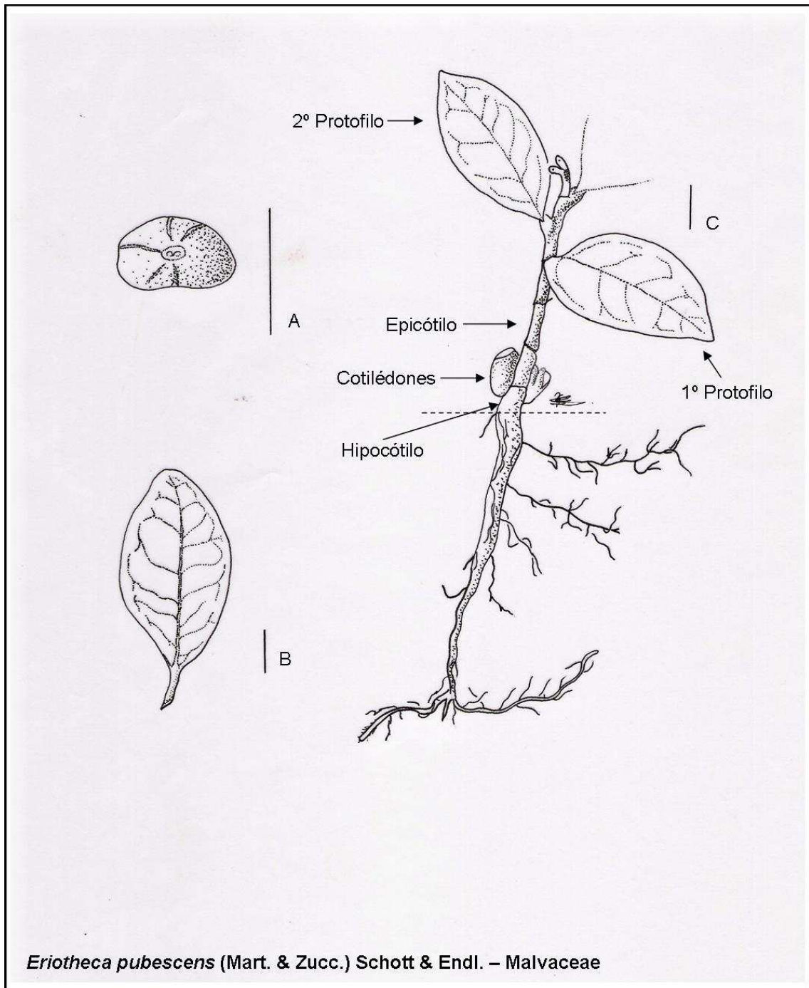
Figura 25. Eriothecha pubescens . A. Semente com estrias; B. Protofilo simples e com pecíolo; C. Plântula FER-III com 70 dias e \pm 17 cm de comprimento (tracejado representa a região do colo). Escala: 1 cm.
