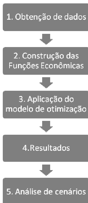
Figura 3.1: Fluxograma Metodológico
