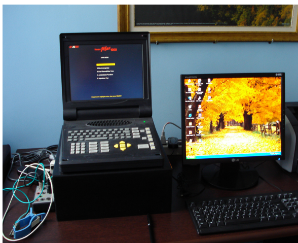
Figura 4 – Equipamento Neuromax 1000;
