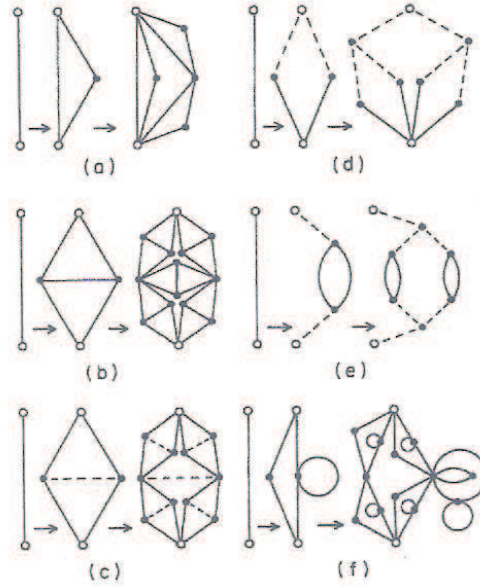
Figura 2.6: Exemplos de gerações de redes hierárquicas (figura retirada da referência [36]).
