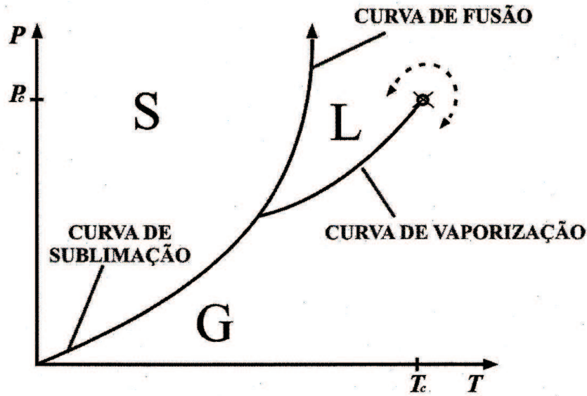
Figura 2.1: Diagrama de fases para sistemas fluidos representado pelo gráfico PT , com as fases sólida ( S ), líquida ( L ) e gasosa ( G ) (figura retirada da referência [21]).
