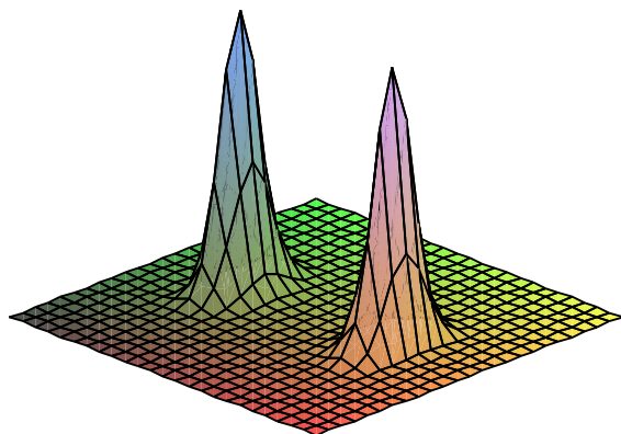
Figura 5.10: Gráfico descrito em [21] quando o valor do bombeio se encontra acima do limiar. Podemos notar que não há semelhança entre ele e a figura 5.7
