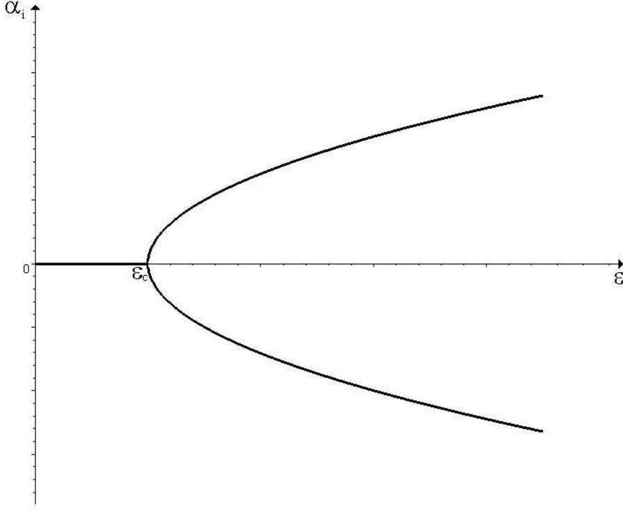
Figura 4.2: Amplitude dos modos amplificados, intacavidade, em função do bombeamento. Abaixo do limiar \epsilon_c apenas flutuações quânticas estão presentes na cavidade e acima de \epsilon_c vemos a presença de campos macroscópicos. Os dois ramos indicam as duas possíveis fases de \alpha .
