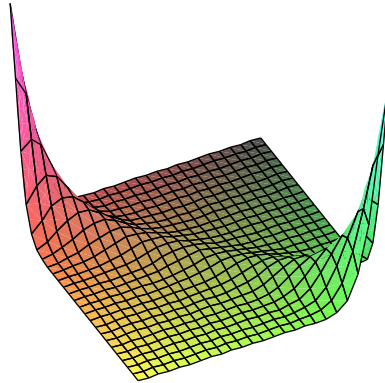
Figura 5.7: Curva de nível para a função linearizada (equação 5.21) quando \mu = 1.1 , e y_1 = y_2 = 0 . Acima do limiar a divergência é total pelo mesmo motivo acima. O termo de correção tem um papel fundamental na descrição do fenômeno: sem ele, a função de Wigner linearizada não consegue representar a realidade encontrada nos laboratórios)
