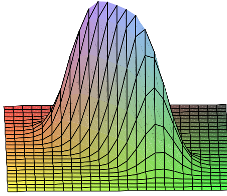
Figura 5.12: Gráfico das curva de nível da função de Wigner completa (equação 5.16) para \mu = 1.0 , e y_1 = y_2 = 0 . Com o termo de correção não-linear presente na expressão, não há mais o aparecimento da divergência mesmo no limiar. O gráfico obtido está de acordo com o relatado em [21] e assemelha-se com a figura 5.9
