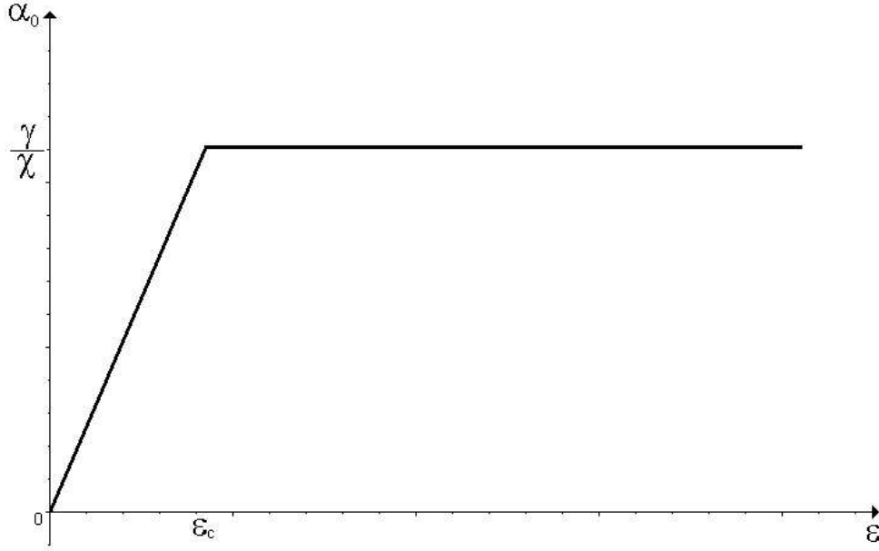
Figura 4.1: Gráfico da amplitude do modo bombeado no OPO em função do bombeamento. Acima do limiar a amplitude fica fixada em \frac{\gamma}{\kappa} , independentemente de \epsilon .
