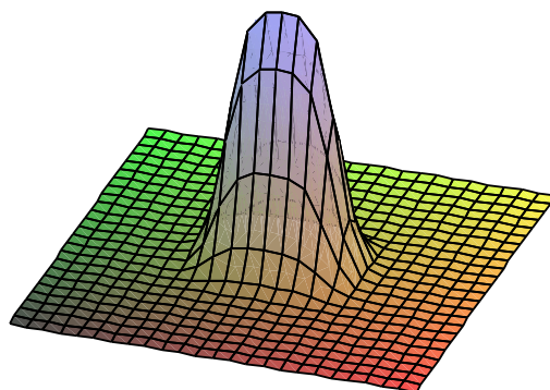
Figura 5.9: Gráfico reportado em [21] quando o valor do bombeio se encontra no limiar. Verifica-se que não há semelhança entre ele e a figura 5.6
