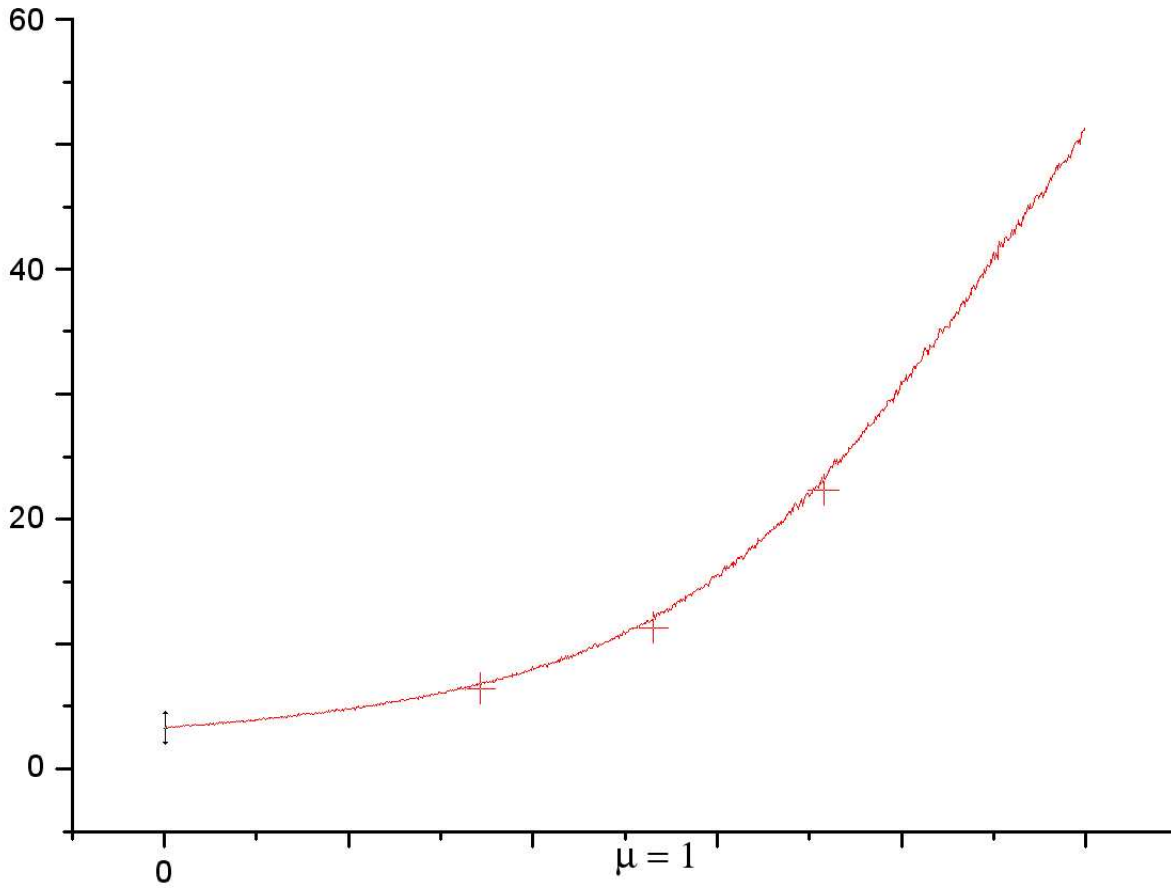
Figura 5.15: Gráfico revelando como o valor esperado de \langle (x_1 + x_2)^2 \rangle e \langle (y_1 - y_2)^2 \rangle variam com a intensidade do bombeamento.
