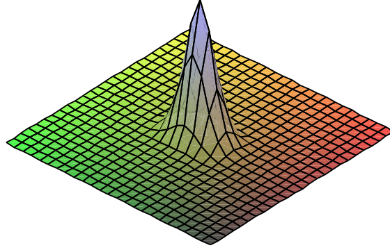
Figura 5.8: Gráfico relatado em [21] quando o valor do bombeio se encontra abaixo do limar. Podemos observar a semelhança entre ele e a figura 5.5
