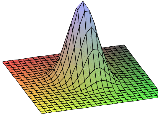
Figura 5.11: Gráfico das curva de nível da função de Wigner completa (equação 5.16) para \mu = 0.5 , e y_1 = y_2 = 0 . Abaixo do limiar, essa figura é similar com a figura 5.5 e 5.8, demonstrando um estado levemente comprimido numa quadratura.
