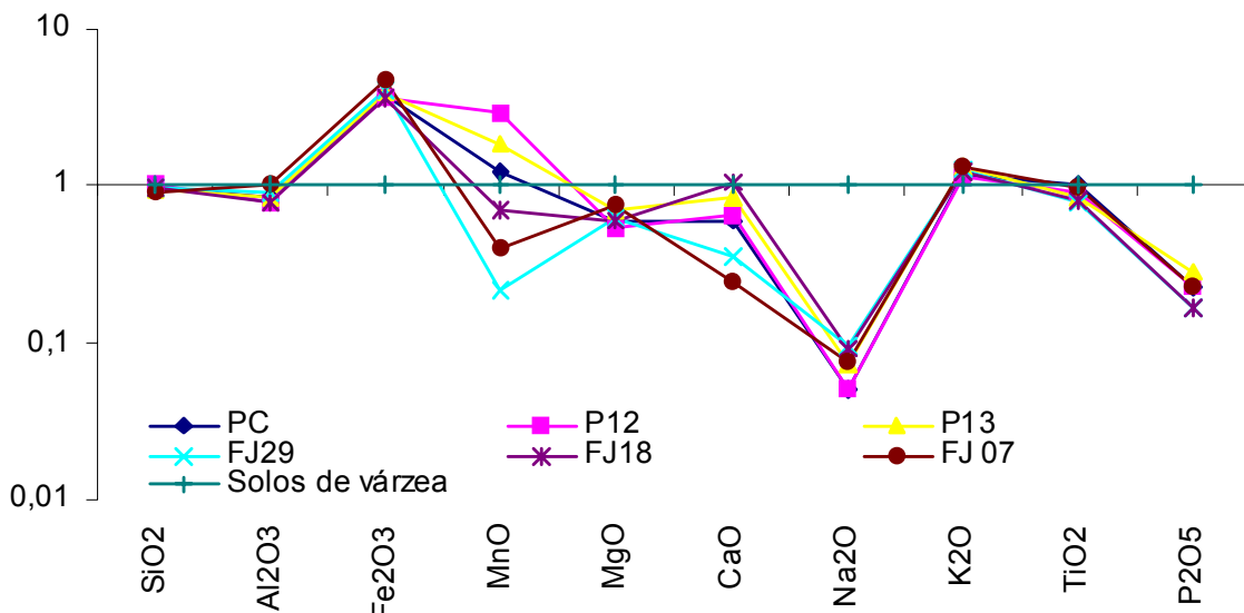
Figura 42 - Normalização das concentrações dos elementos analisados nos solos da região Feijó-Tarauacá com média dos solos de Várzea da região central da Amazônia. Dados dos solos de várzea: Konhauser, Fyfe e Kronberg (1994).
