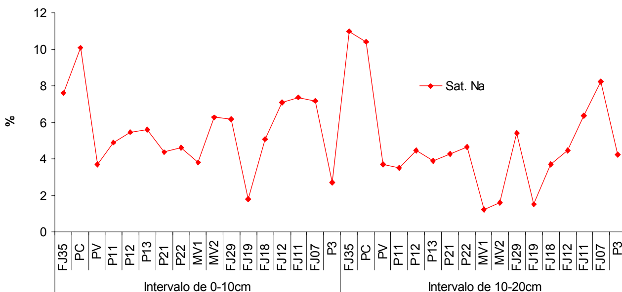
Figura 64 - Distribuição das porcentagens de Saturação de Na (Sat. Na) nos solos da região Feijó-Tarauacá nos intervalos de 0-10 e 10-20cm de profundidades.
