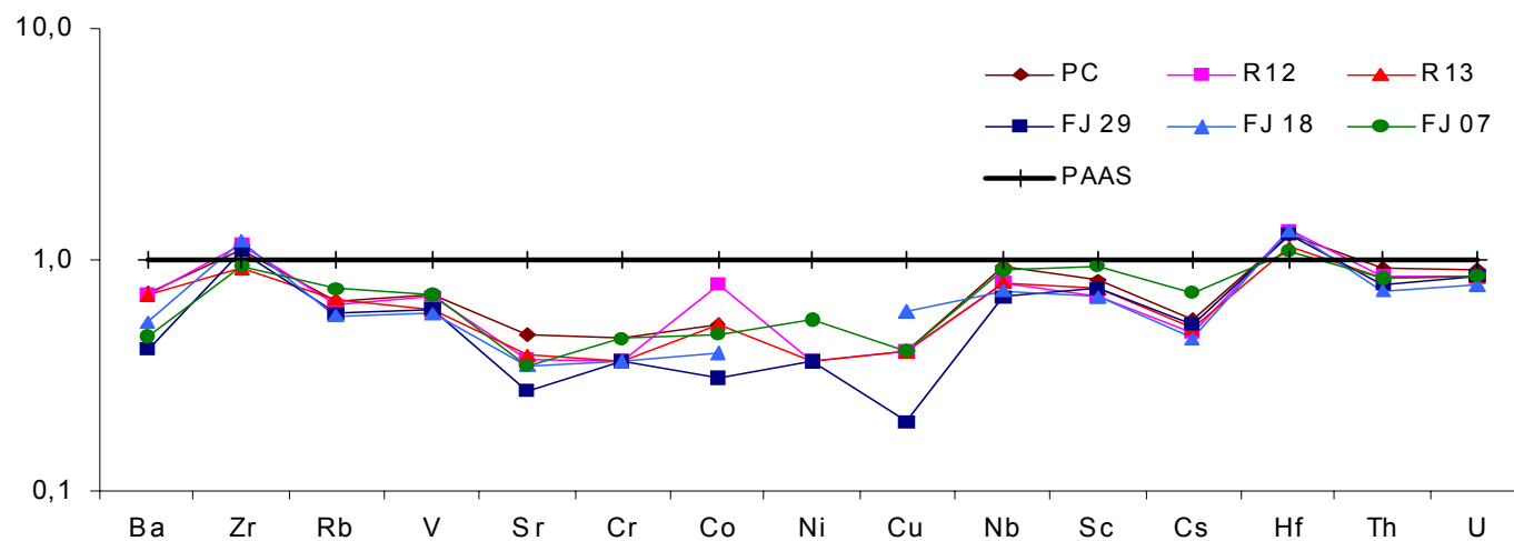
Figura 48 - Normalização das concentrações dos elementos traço dos solos da região Feijó-Tarauacá no intervalo de 0-10cm com os folhelhos pós-arqueanos australianos (PAAS). Dados do PAAS: Taylor e McLennan (1985)
