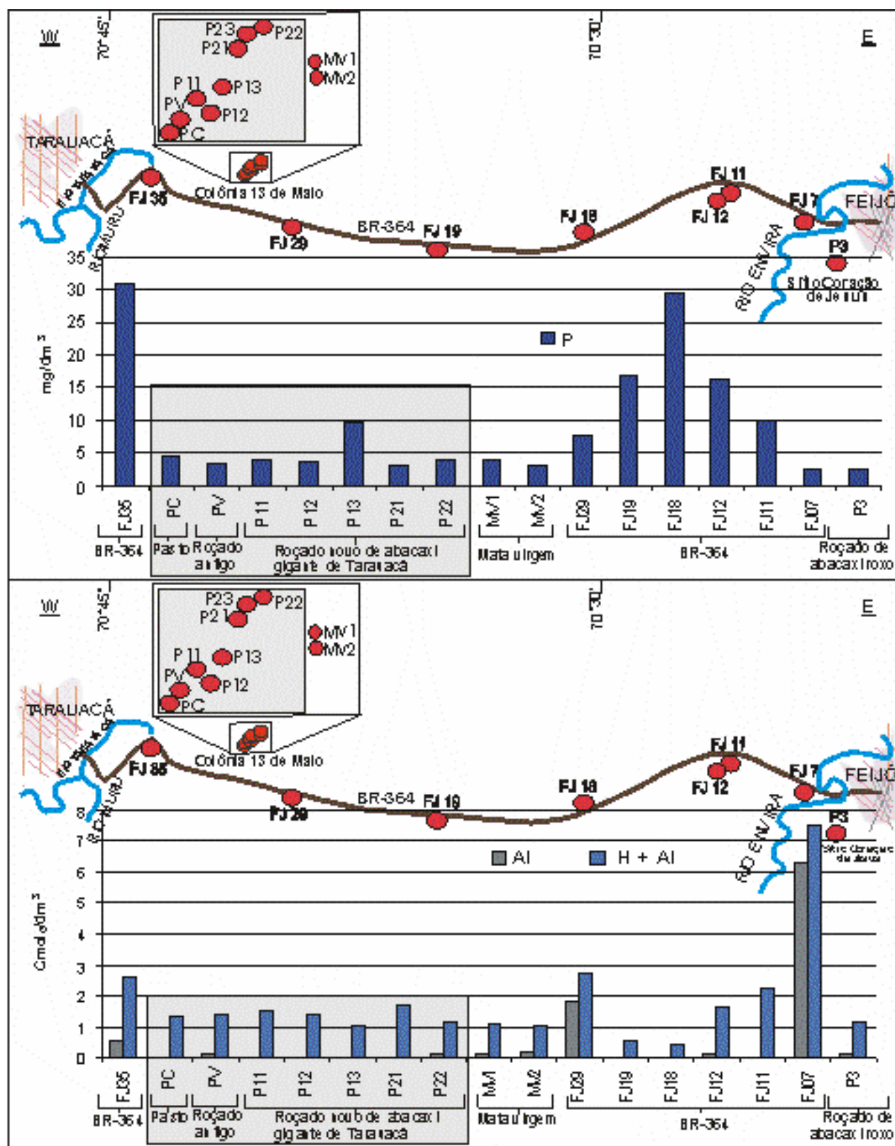
Figura 60 - Distribuição das concentrações de fósforo disponível, alumínio e acidez potencial (Al + H) nos solos da região Feijó-Tarauacá na profundidade de 0-10cm, com destaque para os solos de plantação de abacaxi "Gigante de Tarauacá".
