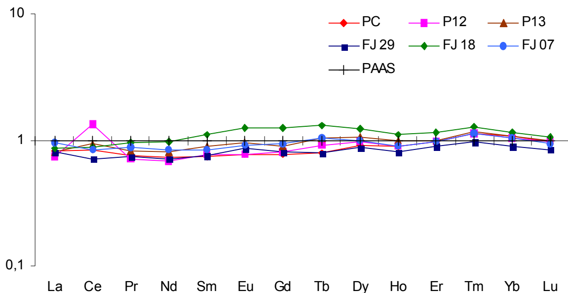
Figura 52 - Normalização dos teores dos elementos terras raras dos solos-sedimentos da região Feijó-Tarauacá no intervalo de 0-10cm com os do PAAS. Dados do PAAS: Taylor e McLennan (1985).
