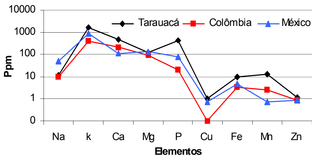
Figura 75 - Distribuição de alguns elementos químicos determinados na polpa do abacaxi gigante de Tarauacá e de abacaxis consumidos em alguns países
