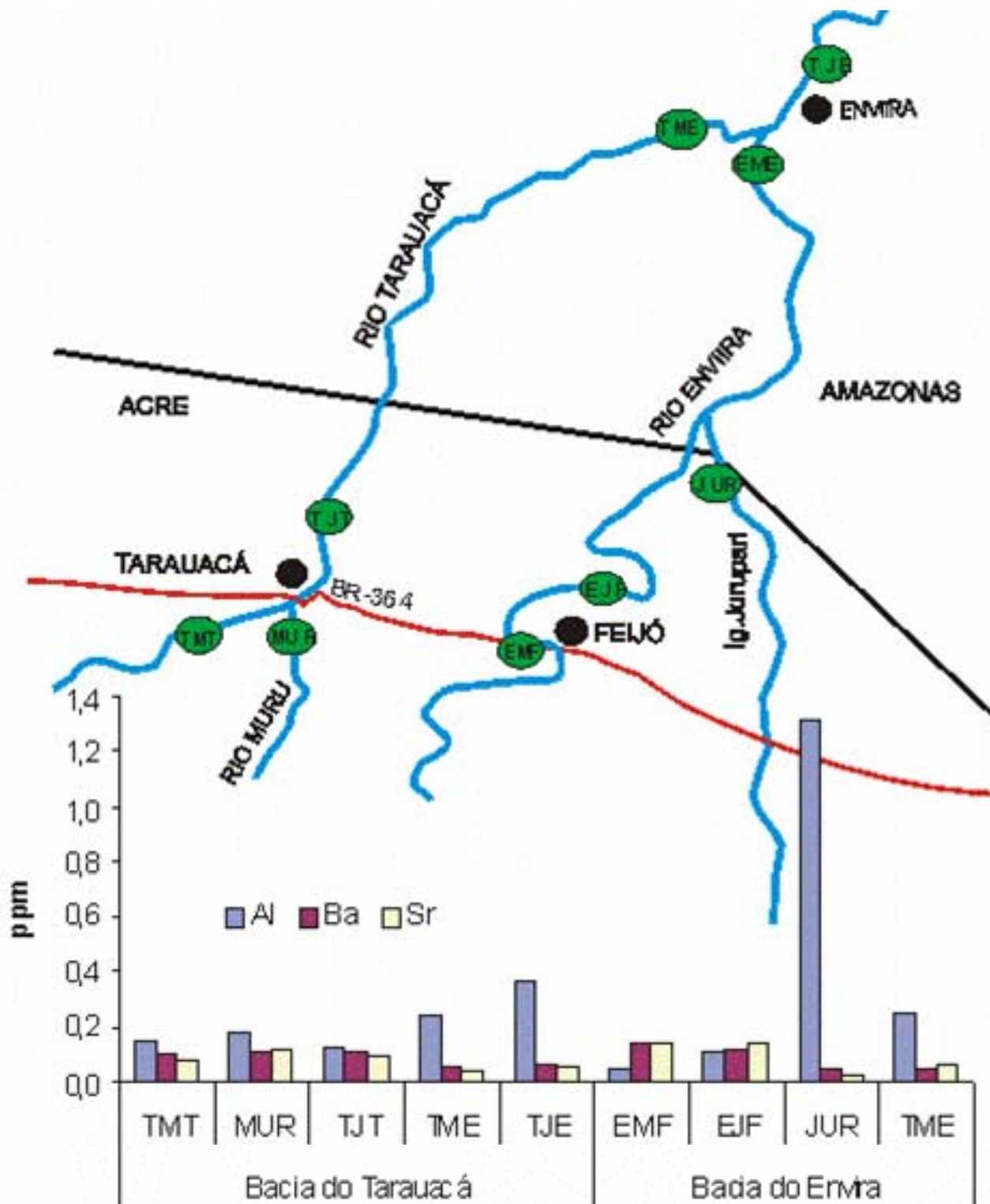
Figura 92 - Distribuição das concentrações de Al, Ba e Sr das águas dos rios da bacia do Tarauacá e do Envira no período de inverno (cheia).
