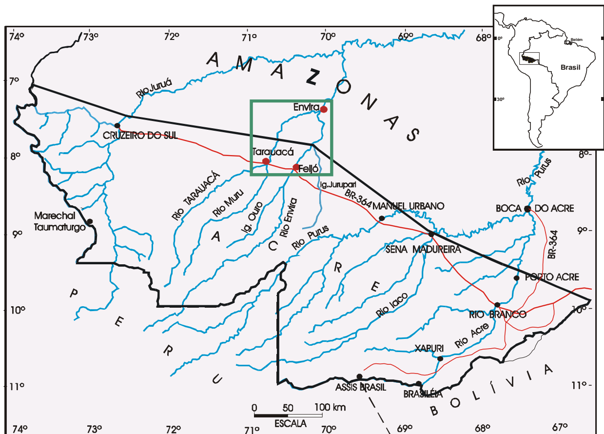
Figura 1 - Localização do Estado do Acre com destaque para a região de estudo Feijó-Tarauacá-Envira, compreendendo a área entre as cidades de Tarauacá, Feijó e Envira.
