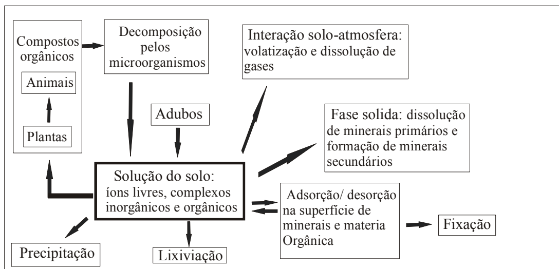
Figura 7 - Dinâmica do solo envolvendo a solução do solo e os nutrientes. Adaptado de Tomé Jr. (1997) e Cotter-Howells e Paterson (2000).
