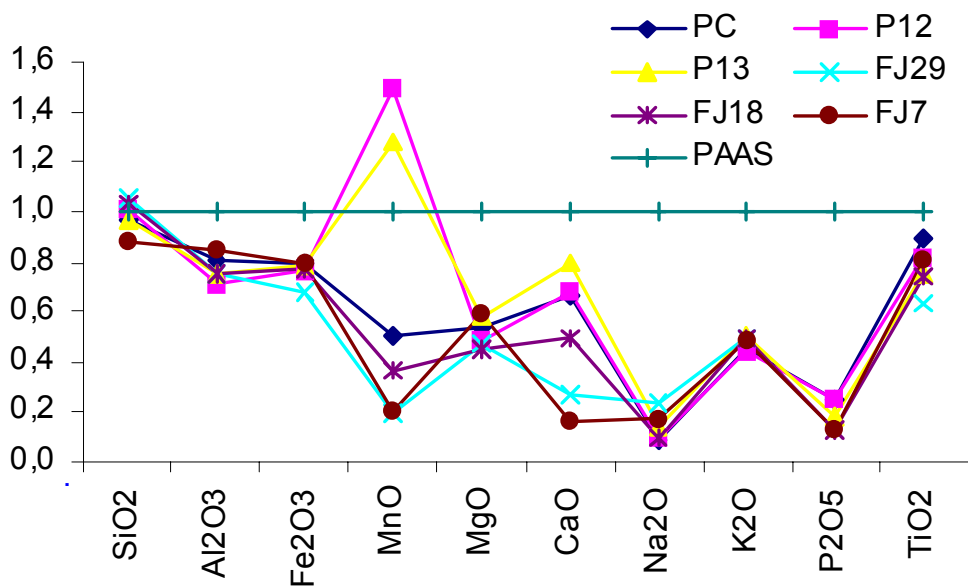
Figura 39 - Normalização das concentrações dos elementos analisados nos solos da região Feijó-Tarauacá na profundidade de 10-20cm com a dos folhelhos australianos pós-arqueanos-PAAS. Os dados para PAAS são de Taylor e McLennam (1985).
