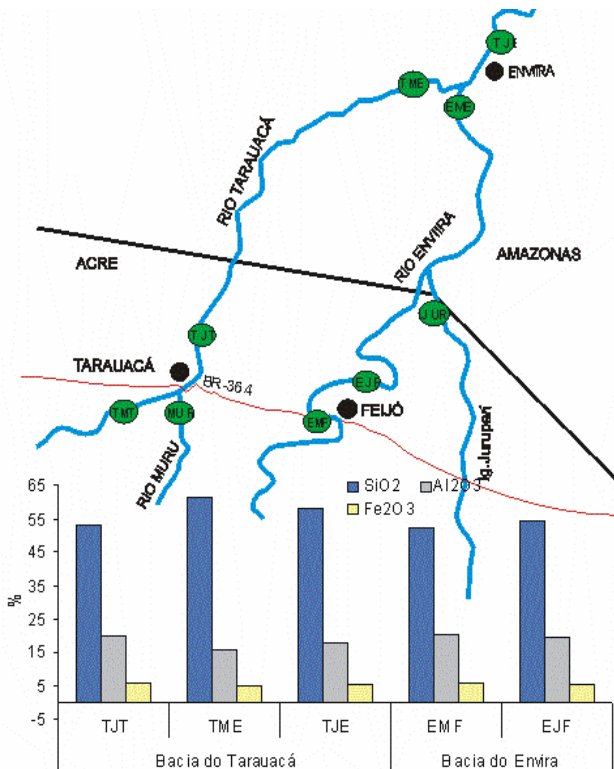
Figura 93 - Distribuição das concentrações de SiO 2 , Al 2 O 3 e Fe 2 O 3 nos suspensos dos rios da bacia do Tarauacá e do Envira no período de inverno (cheia).
