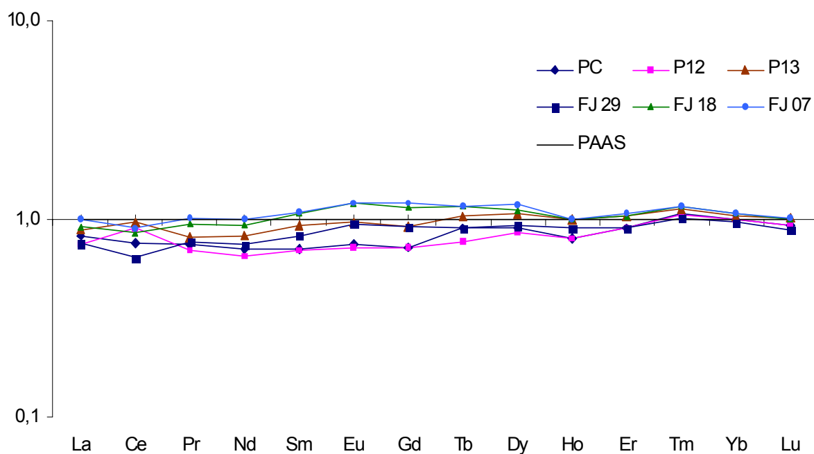
Figura 53 - Normalização dos teores dos elementos terras raras dos solos-sedimentos da região Feijó-Tarauacá no intervalo de 10-20cm com os do PAAS. Dados do PAAS: Taylor e McLennan (1985).
