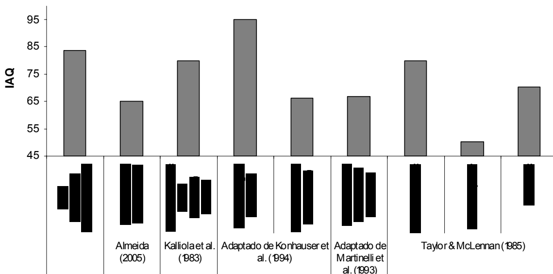
Figura 45 - Índice de alteração química (IAQ) para a média dos solos-sedimentos estudados na região Feijó-Tarauacá comparados a outros materiais de referência.
