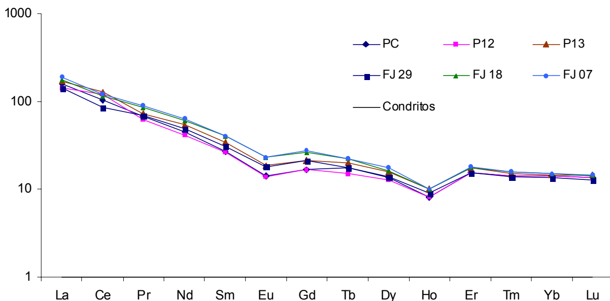
Figura 55 - Normalização dos teores dos elementos terras raras dos solos-sedimentos da região Feijó-Tarauacá no intervalo de 10-20cm aos condritos. Dados para condritos: Evensen, Hamilton e O'nions (1978).
