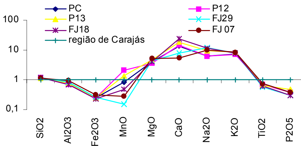
Figura 41 - Normalização das concentrações dos elementos analisados nos solos da região Feijó-Tarauacá com média dos solos da região de Carajás, estado do Pará. Dados da região de Carajás: Konhauser, Fyfe e Kronberg (1994).
