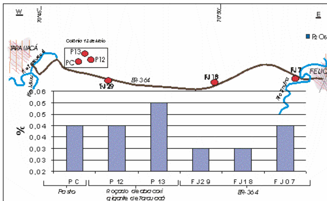
Figura 32 - Distribuição das porcentagens de P 2 O 5 nos solos da região Feijó-Tarauacá no intervalo de 0-10cm de profundidade.
