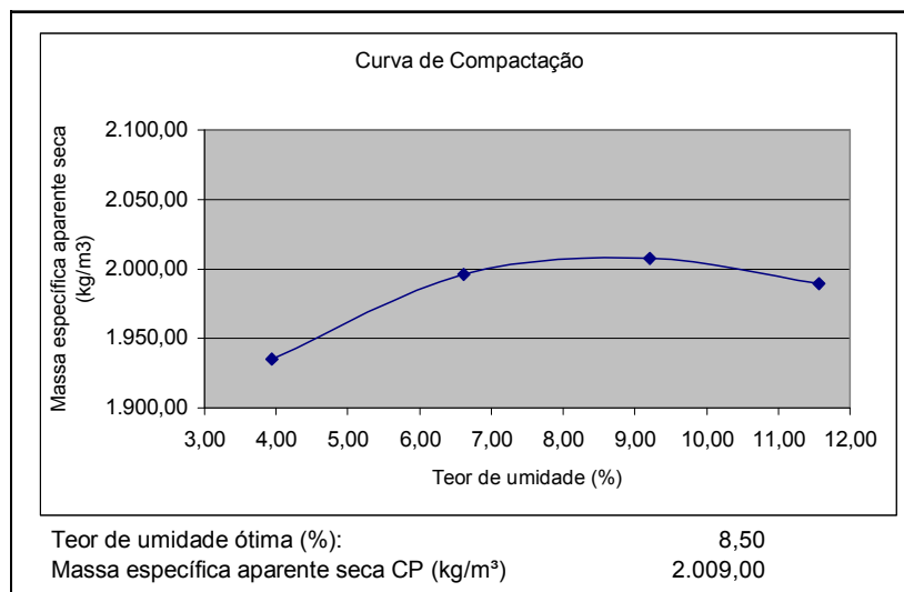
Figura 3.17- Curva de compactação- mistura de dosagem 60% BGS e 40% material fresado, com 3% de cimento.
