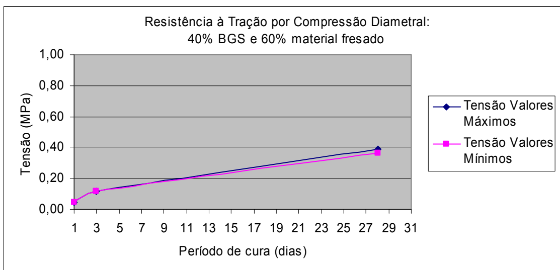
Figura 3.31- Resultado do ensaio de resistência à tração por compressão diametral para dosagem 40% BGS e 60% material fresado.
