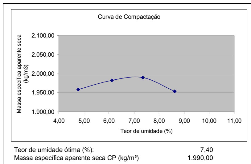
Figura 3.18- Curva de compactação- mistura de dosagem 50% BGS e 50% material fresado, com 3% de cimento.
