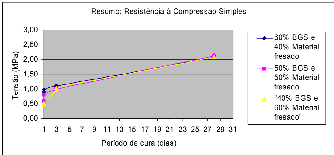
Figura 3.32- Resumo dos resultados do ensaio de resistência à compressão simples.
