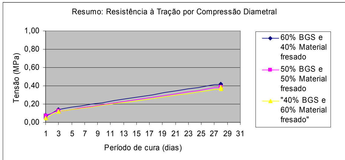
Figura 3.33- Resumo dos resultados do ensaio de resistência à tração por compressão diametral.
