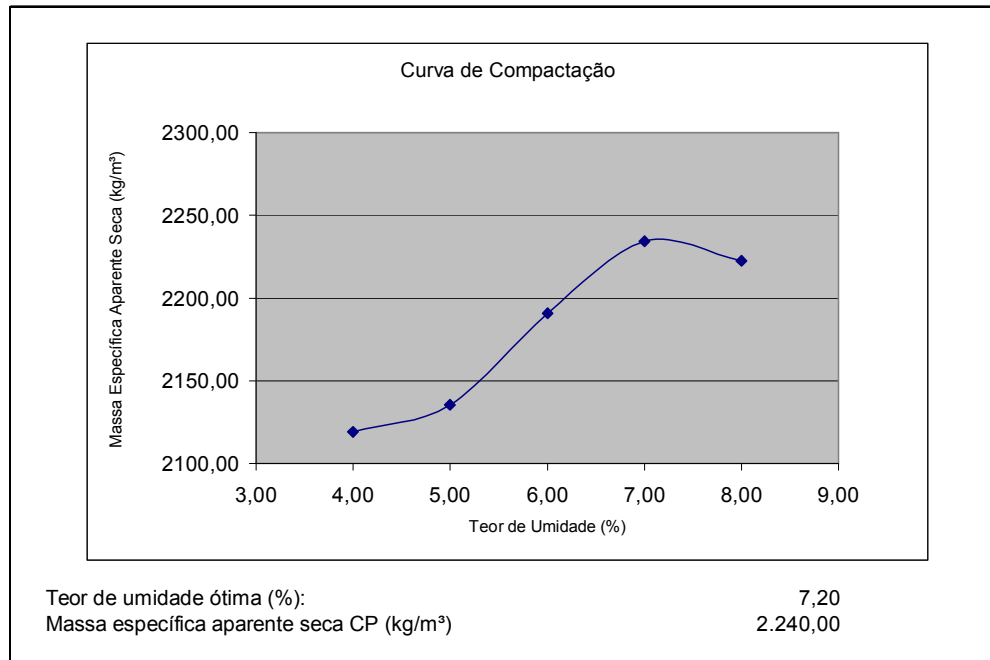
Figura 3.4- Curva de compactação da BGS
