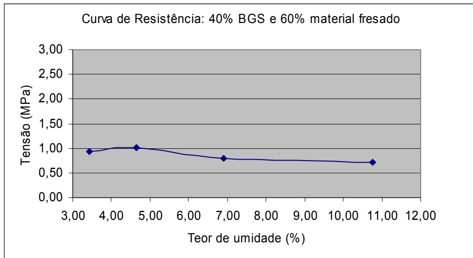
Figura 3.23- Curva de resistência- mistura de dosagem 40% BGS e 60% material fresado, com 3% de cimento.
