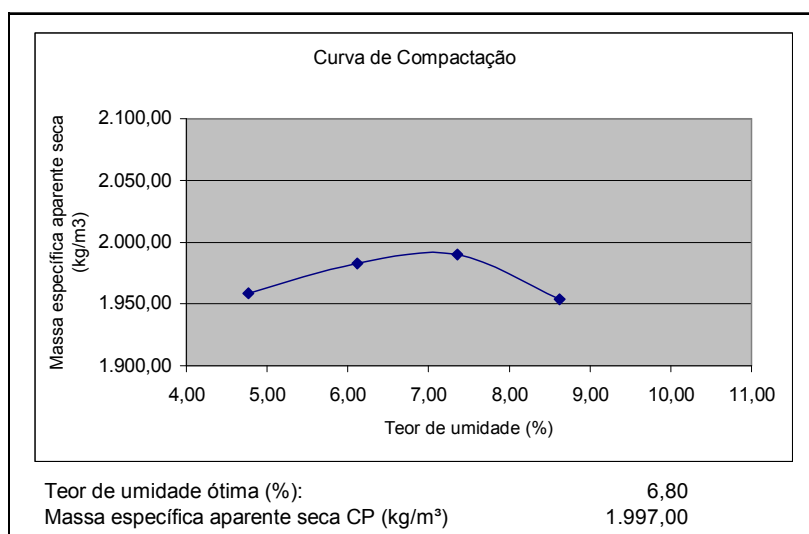
Figura 3.19- Curva de compactação- mistura de dosagem 40% BGS e 60% material fresado, com 3% de cimento.
