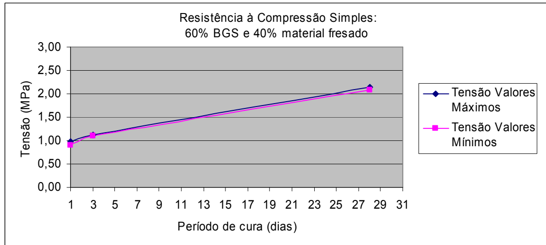
Figura 3.26- Resultado do ensaio de resistência à compressão simples para dosagem 60% BGS e 40% material fresado.
