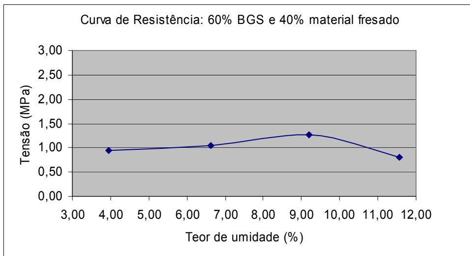
Figura 3.21- Curva de resistência- mistura de dosagem 60% BGS e 40% material fresado, com 3% de cimento.
