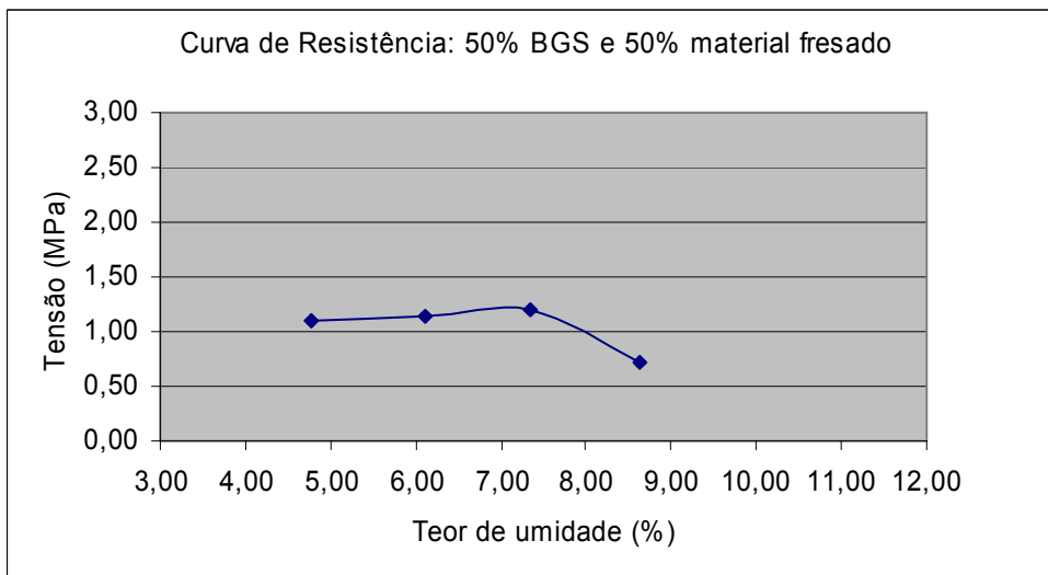
Figura 3.22- Curva de resistência- mistura de dosagem 50% BGS e 50% material fresado, com 3% de cimento.
