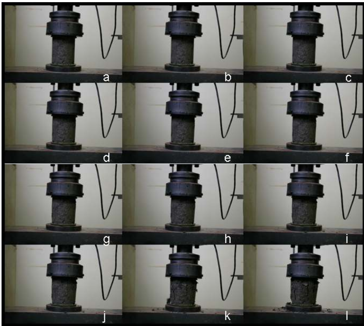
Figura- Seqüência de ruptura de corpo de prova no ensaio de resistência à compressão simples- 3ª série de ensaios.
