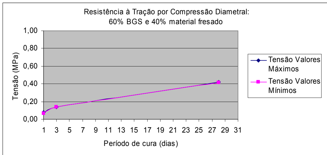
Figura 3.29- Resultado do ensaio de resistência à tração por compressão diametral para dosagem 60% BGS e 40% material fresado.
