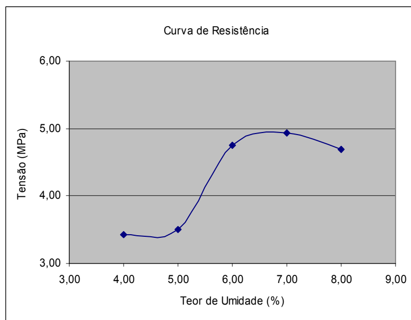
Figura 3.9- Curva de resistência (resistência x teor de umidade).
