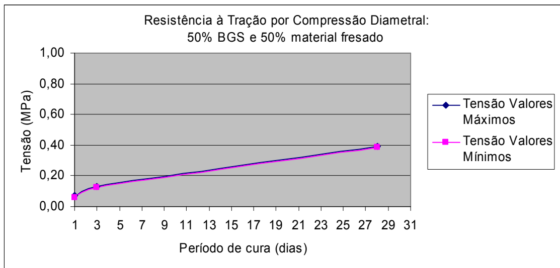
Figura 3.30- Resultado do ensaio de resistência à tração por compressão diametral para dosagem 50% BGS e 50% material fresado.
