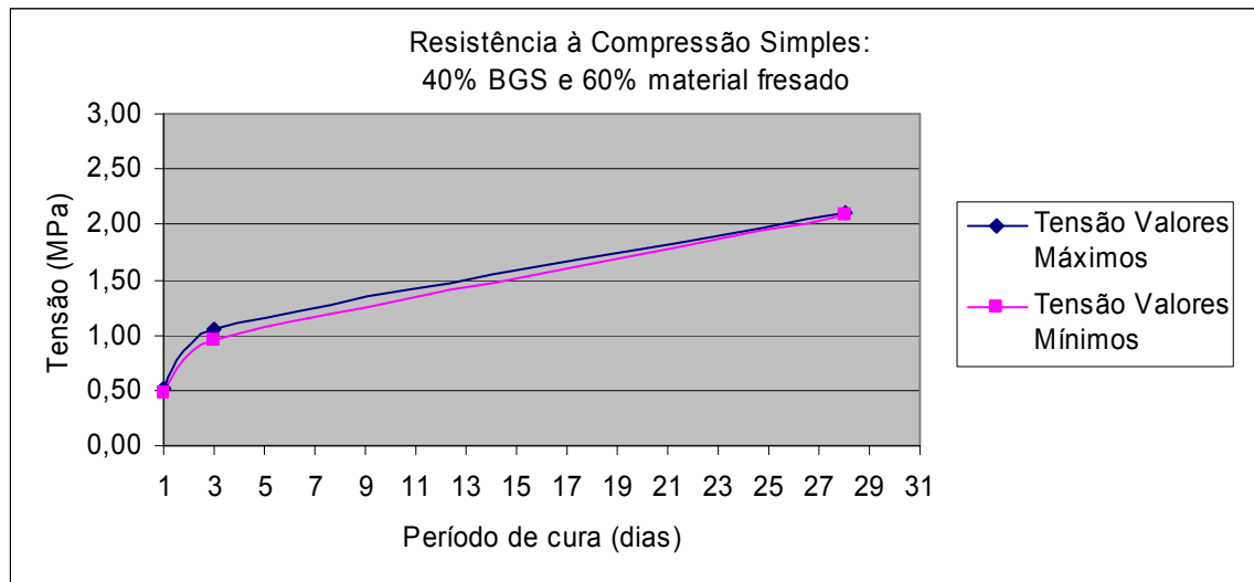
Figura 3.28- Resultado do ensaio de resistência à compressão simples para dosagem 40% BGS e 60% material fresado.
