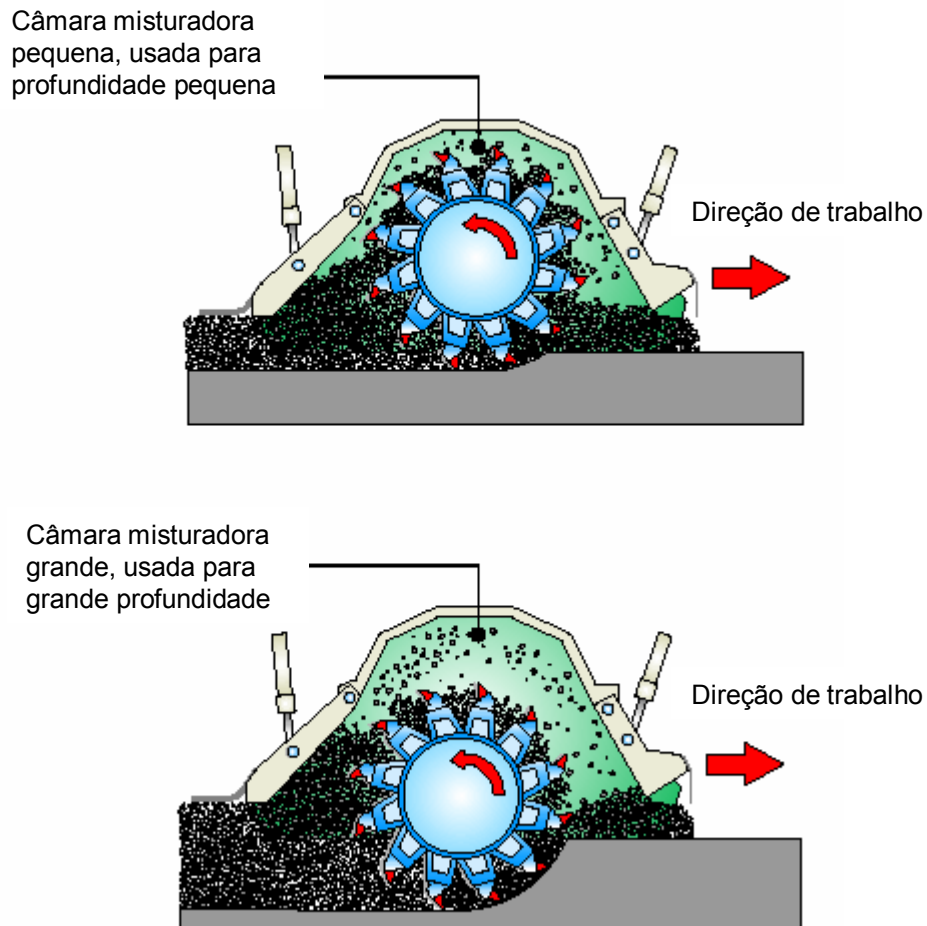
Figura 2.22- Câmara de trabalho e do bico para aspergir água ou emulsão Asfáltica- Raco 350- Wirtgen. Fonte: Wirtgen América (2006).
