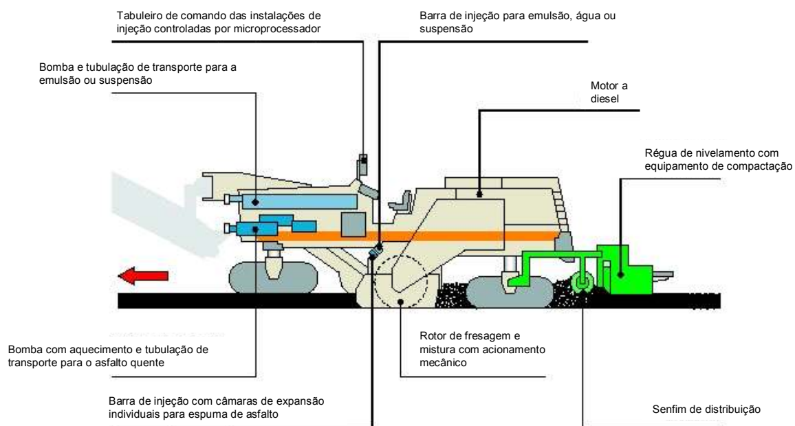
Figura 2.18- Vista detalhada- 2200 CR- Wirtgen. Fonte: Wirtgen América (2006).
