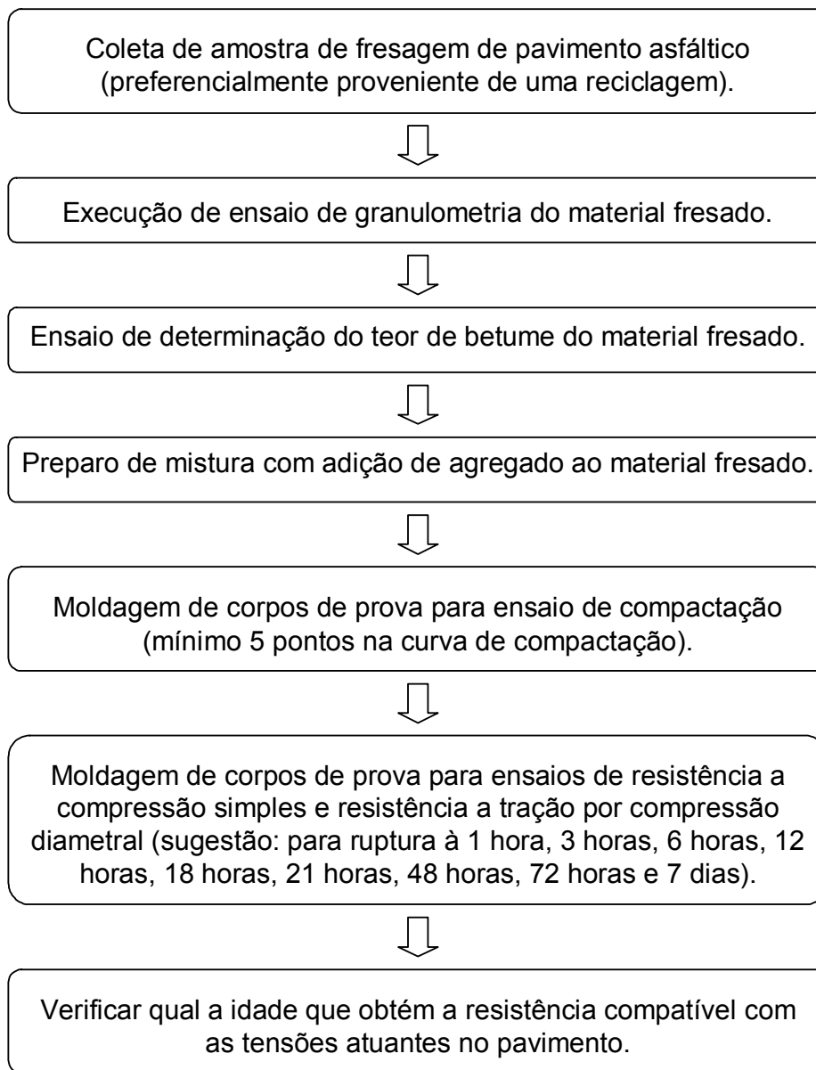
Figura 4.1- Proposta de dosagem na reciclagem de pavimento asfáltico com cimento Portland.
