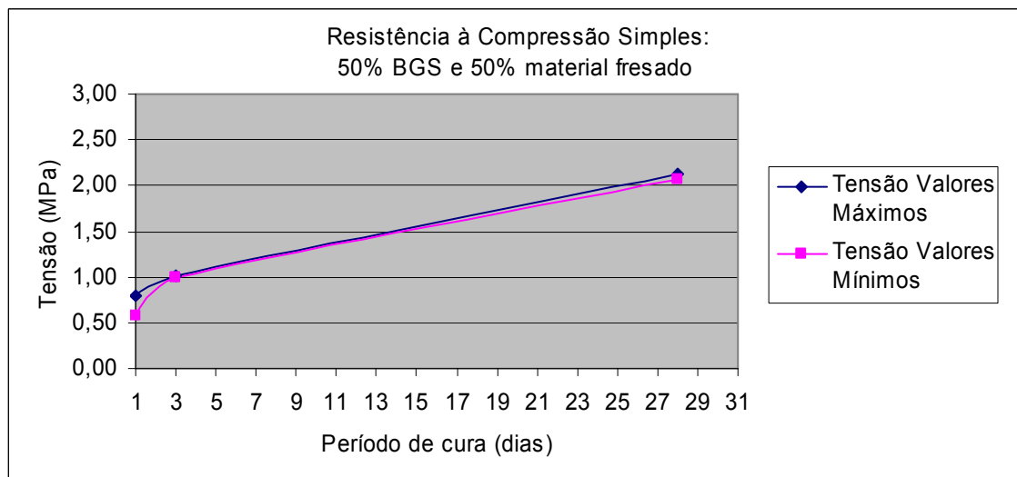
Figura 3.27- Resultado do ensaio de resistência à compressão simples para dosagem 50% BGS e 50% material fresado.
