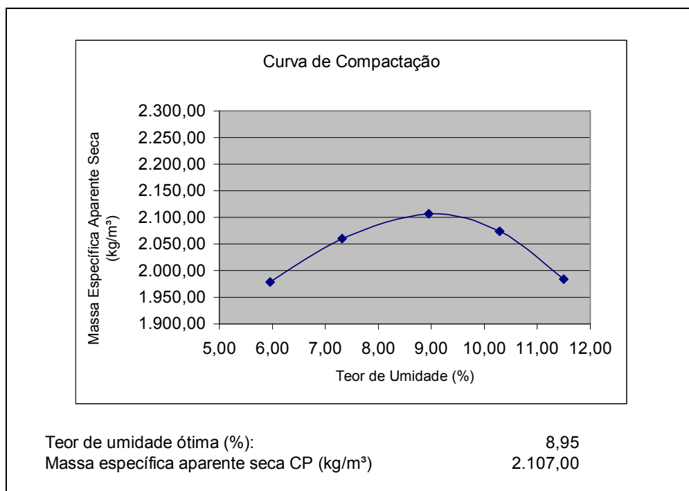
Figura 3.13- Curva de compactação.
