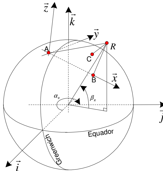
Figura 16. Coordenadas transladas do centro do planeta para a sua superfície, centradas na base A[37].
