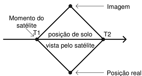
Figura 3: O cruzamento dos cones gera uma posição real e imaginária[9].
