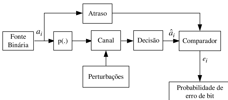
Figura 14: Modelo de simulação utilizando o método de Monte Carlo.
