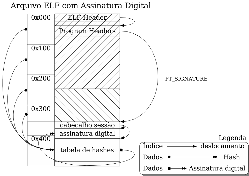
Figura 5.4: Exemplo de um arquivo ELF com assinatura digital embutida
