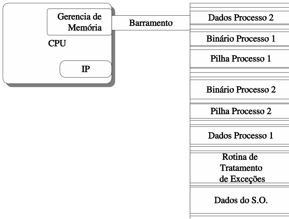
Figura 2.4: Distribuição da memória do sistema
