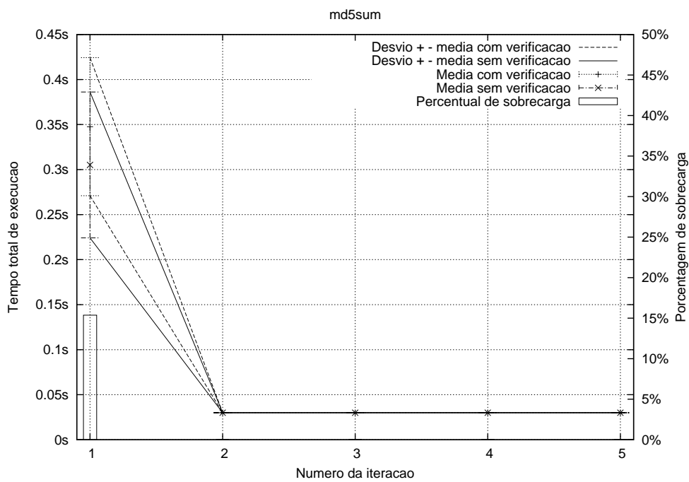
Figura 6.2: Gráfico de impacto sobre a velocidade do programa md5sum
