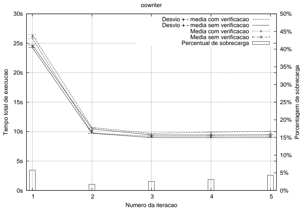
Figura 6.5: Gráfico de impacto sobre a velocidade do programa Open Office
