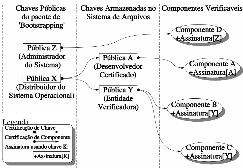
Figura 3.3: Exemplo de sistema utilizando uma árvore de certificações
