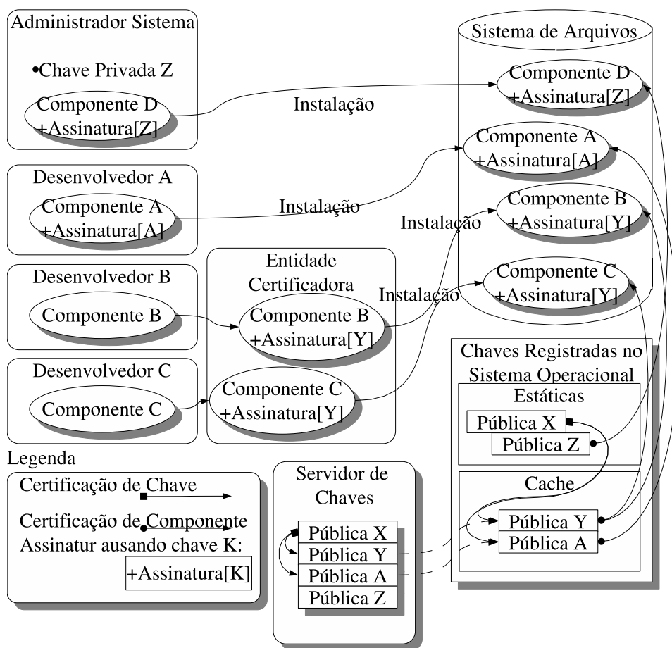
Figura 3.5: Relações entre certificadores e verificação para sistema baseado em chaves públicas
