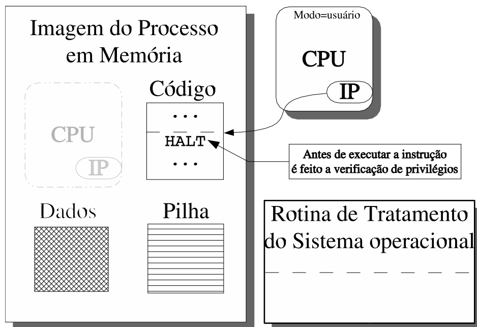
Figura 2.1: Verificação do nível de segurança
