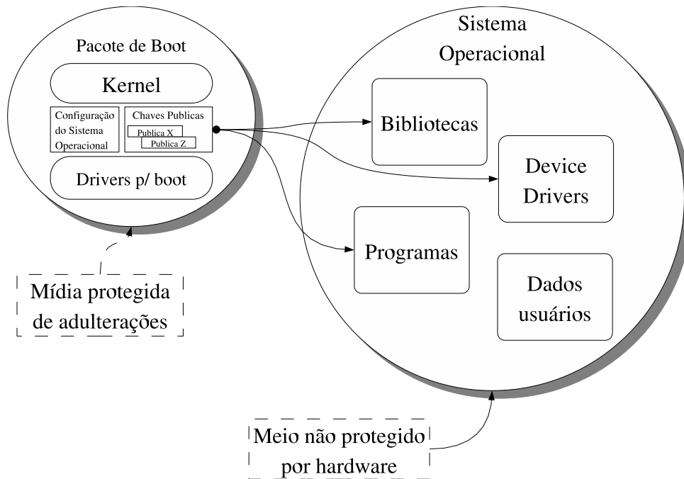
Figura 3.4: Configuração de um sistema com bootstrap para verificação de assinaturas
