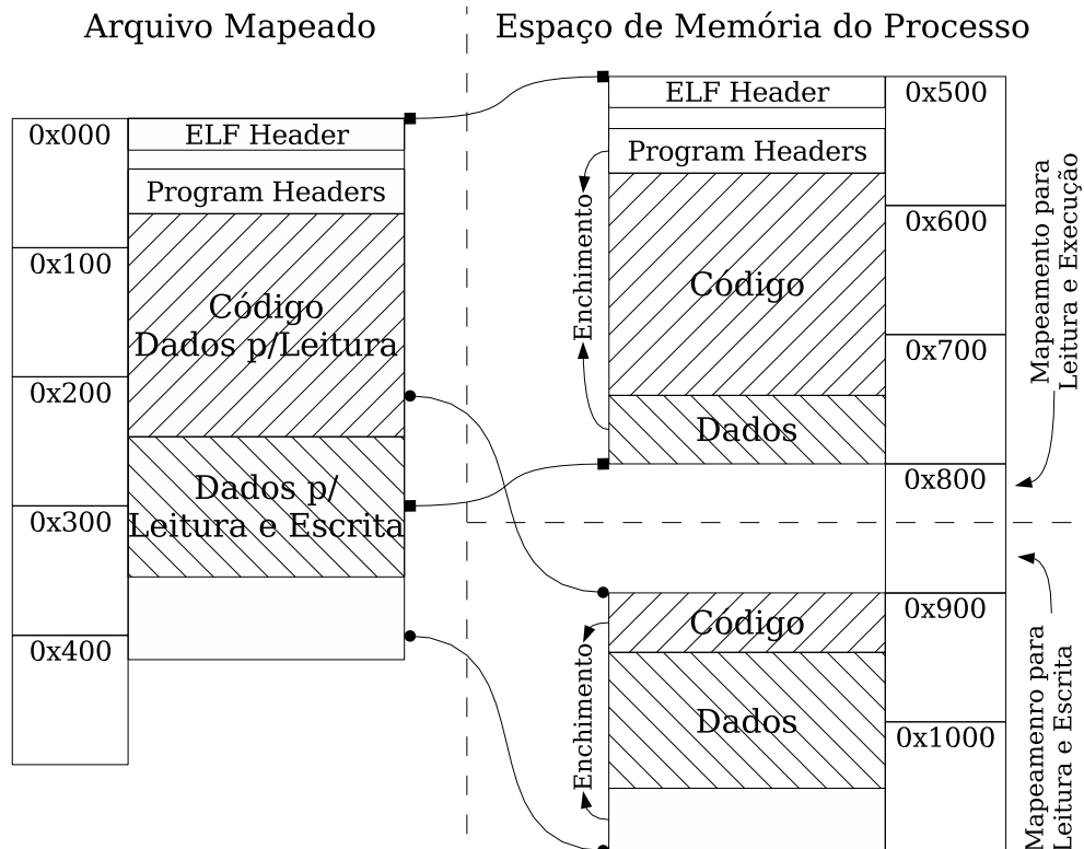
Figura 5.3: Correspondência entre arquivo mapeado em memória e a imagem do processo
