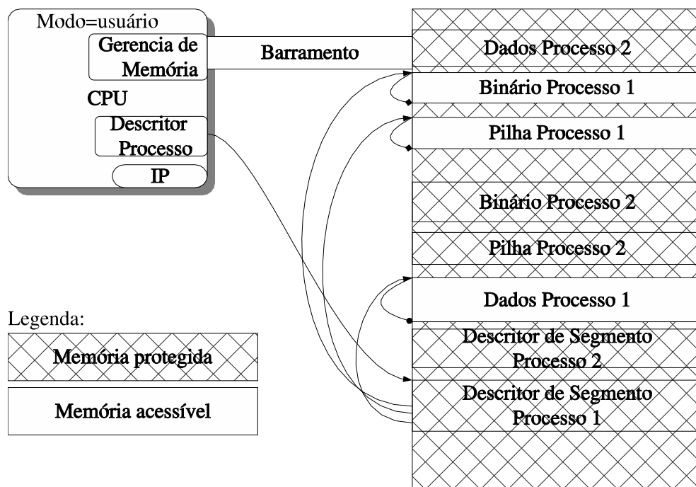
Figura 2.5: Exemplo de processador em modo protegido, utilizando segmentação
