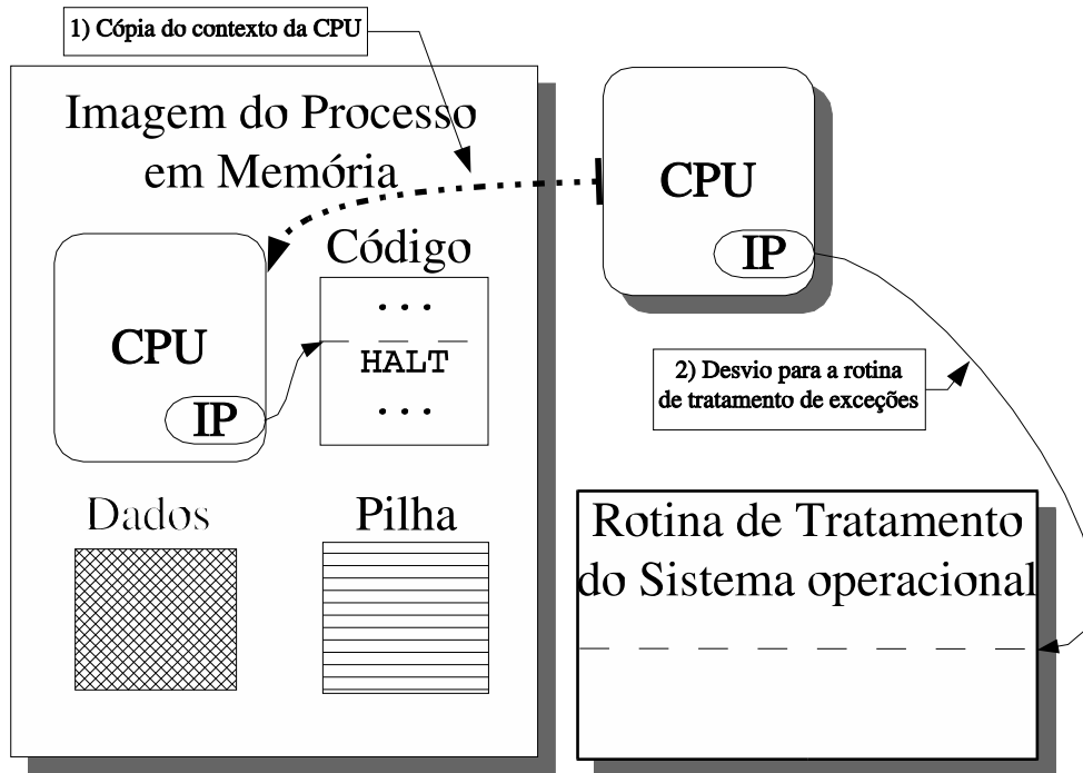
Figura 2.2: Desvio do fluxo de execução
