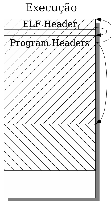
Figura 5.2: Formato ELF , destacando as áreas de mapeamento em memória
