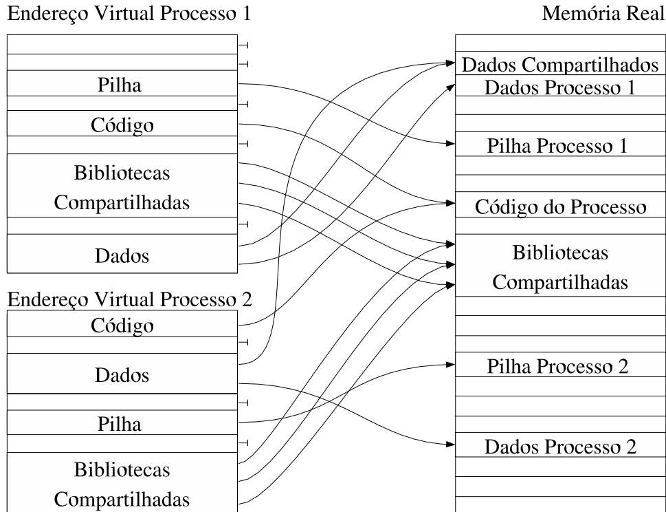
Figura 2.7: Exemplo de dois endereços virtuais que utilizam um mesmo endereço físico
