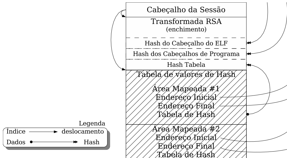
Figura 5.5: Formato da sessão com as estruturas de controle da assinatura digital
