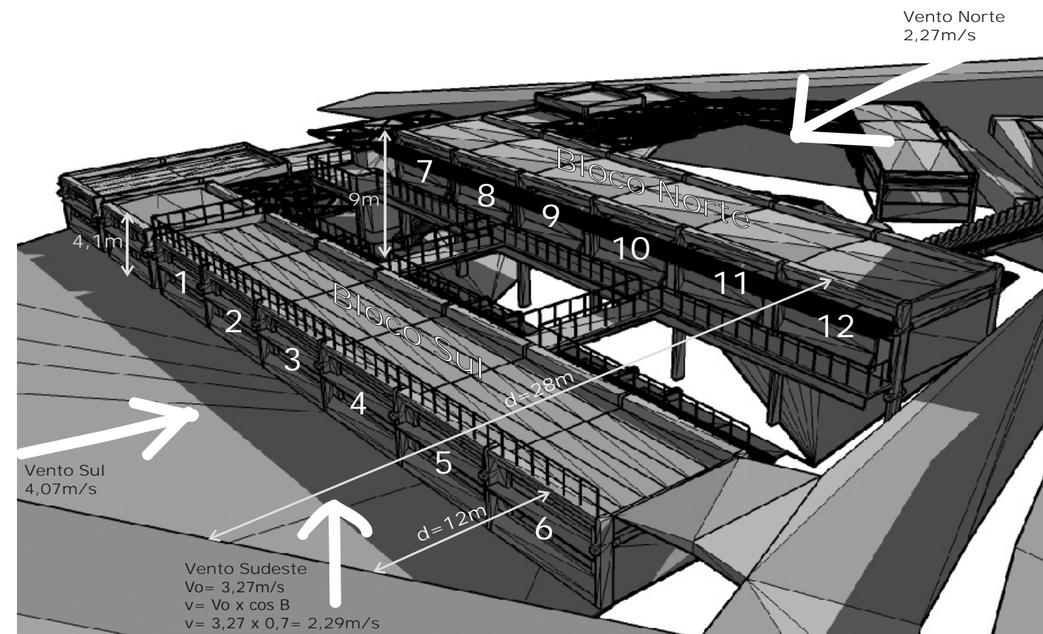
Figura 86- Esquema geral da ventilação sobre os blocos de salas de aula: direção, velocidade dos ventos, distância dos ante-paraos
