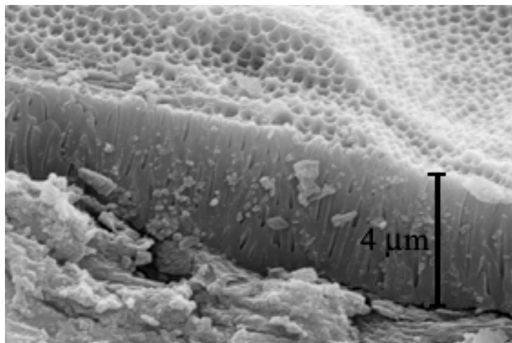
Figura 24 : Micrografias transversal do eletrodo S06, anodizado em 0,1 M H_3PO_4 com 20 \text{ mA/cm}^2 em duas etapas. A primeira realizada por 3600 s à 6^\circ\text{C} e a segunda por 1800 s à 24^\circ\text{C} . Entre as duas etapas o óxido foi removido em solução mista de ácido crômico e fosfórico, conforme Tabela 1.
