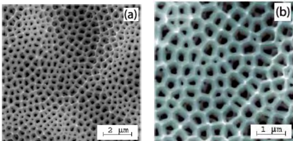
Figura 25 : Micrografias de diferentes regiões do eletrodo S07, anodizado em 0,1 M H_3PO_4 em duas etapas. A primeira realizada por 3600 s à 6 °C com 10 mA/cm 2 e a segunda por 1800 s à 24 °C com 20 mA/cm 2 . Entre as duas etapas o óxido foi removido em solução mista de ácido crômico e fosfórico, conforme Tabela 1.
