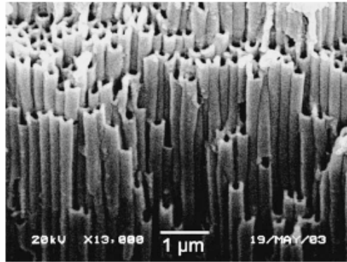
Figura 38 : A direita uma micrografia de SEM dos nanotubos de cobalto [52] .
