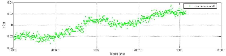
Figura 19 - Componente Norte
