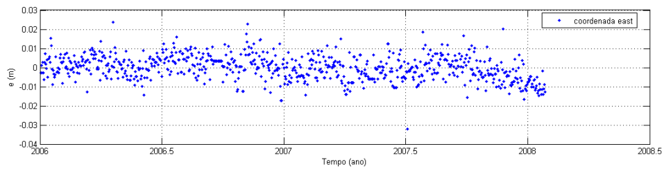
Figura 18 - Componente Leste
