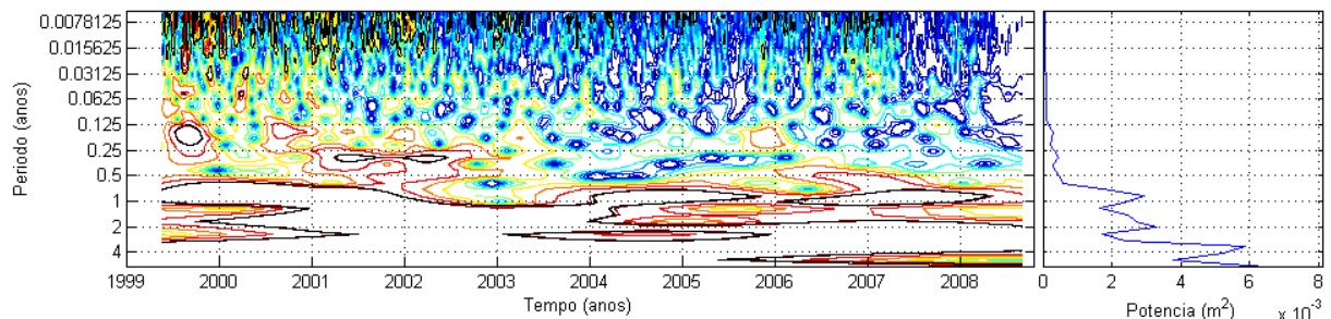
Figura 41 – Espectro de wavelets e potência para a componente após a remoção do efeito anual
