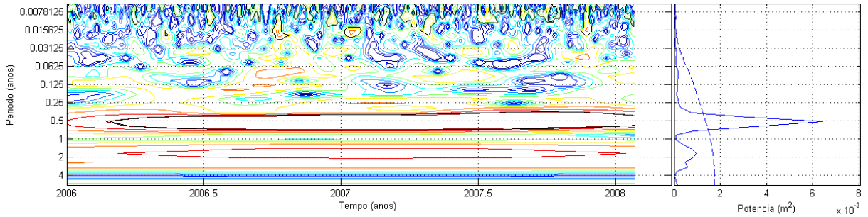
Figura 23 - Espectro de wavelets para a componente Vertical com efeito anual removido
