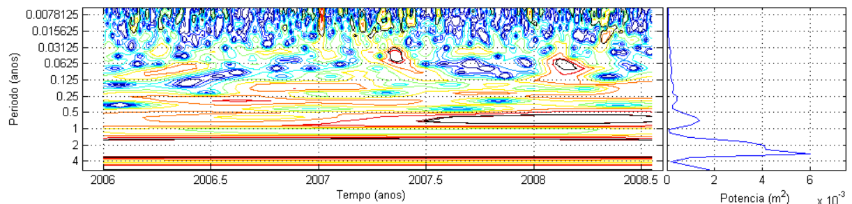
Figura 46 – Espectro de wavelets e potência para a componente Vertical com o efeito anual removido
