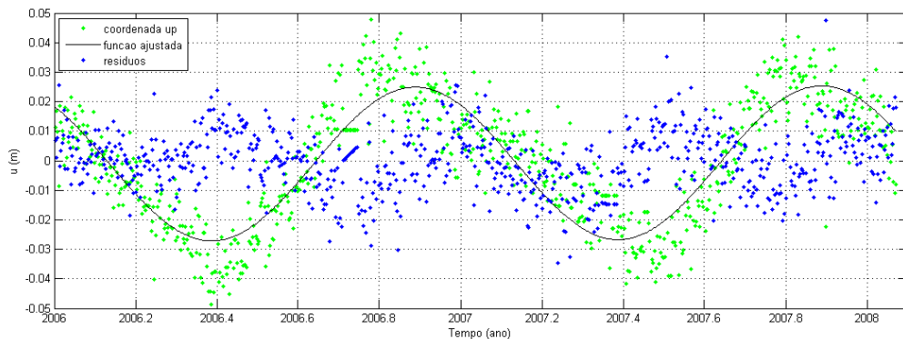
Figura 22 – Série temporal da componente Vertical e curva ajustada
