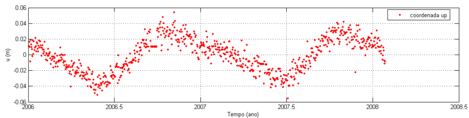
Figura 20 - Componente Vertical
