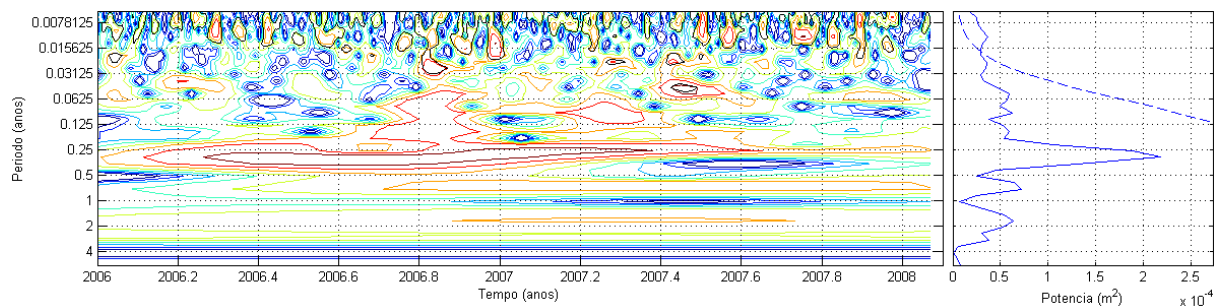
Figura 31 – Espectro de wavelets para a componente leste removido os efeitos anual e semianual
