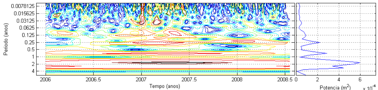
Figura 51 - Espectro de wavelets e potência para a componente Leste após a remoção do efeito anual
