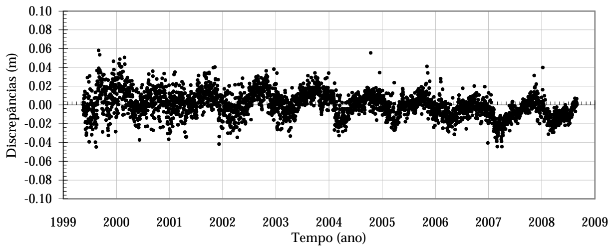
Figura 33 – Componente Norte
