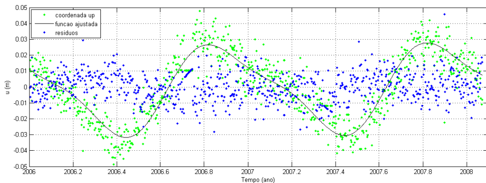
Figura 24 - Componente Vertical com efeitos anual e semi-anual removidos
