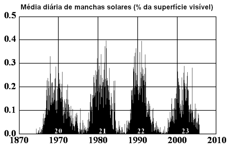
Figura 37 - Manchas solares
