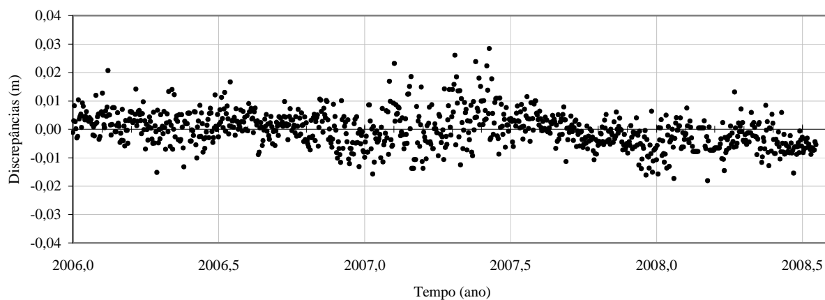
Figura 42 – Componente Leste
