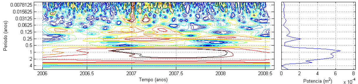
Figura 50 – Espectro de wavelets e potência para a componente Leste
