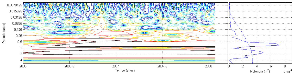
Figura 28 – Espectro de wavelets para a série da componente Norte corrigida dos efeitos anual e semi-anual
